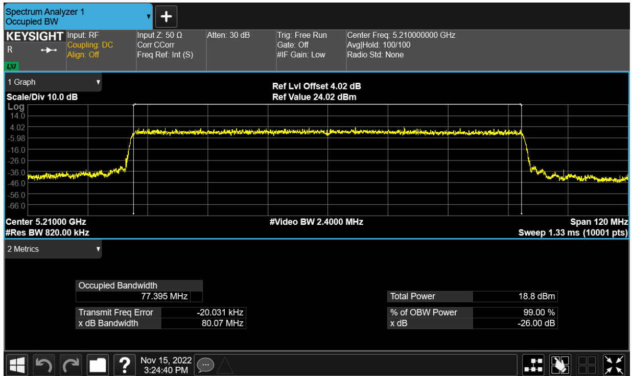
OBW NVNT ax80 5210MHz Ant24
