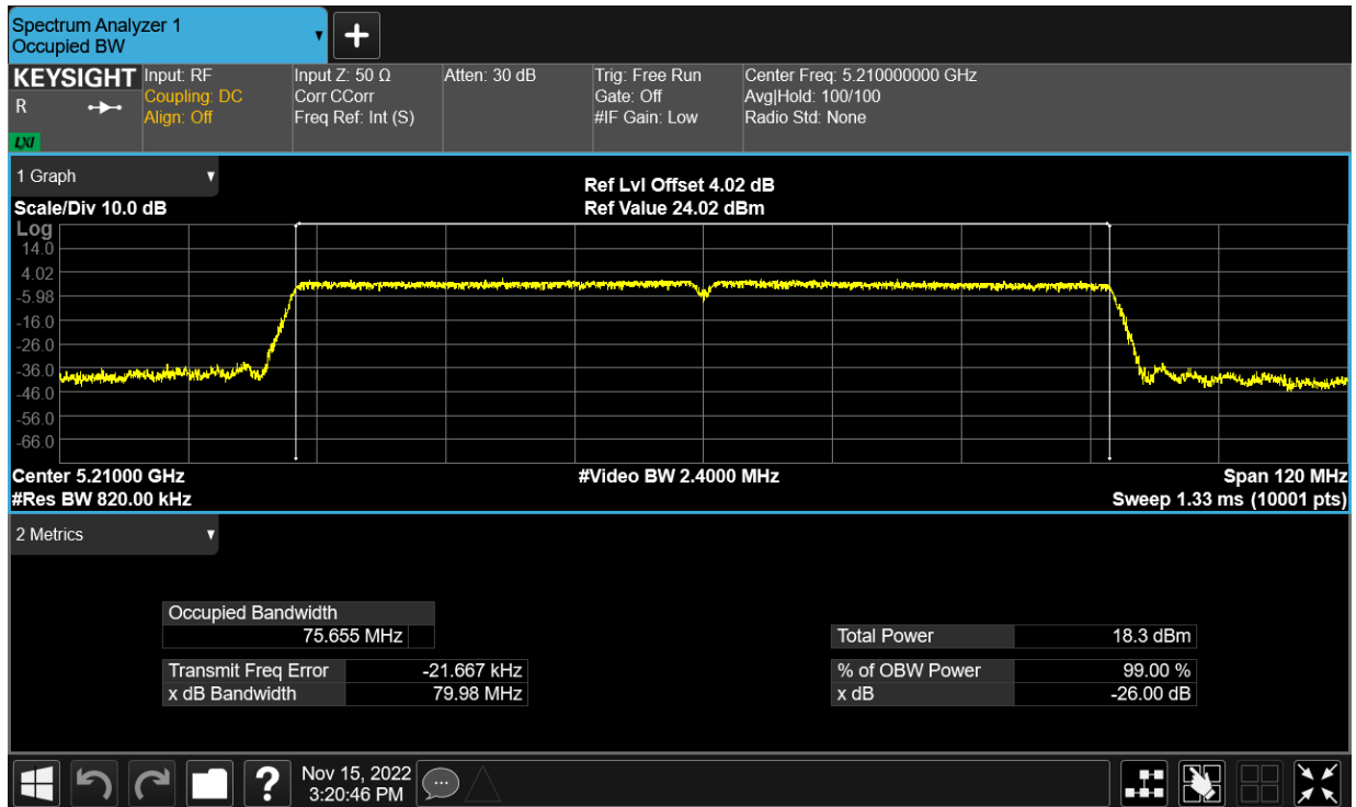
OBW NVNT ac80 5210MHz Ant24
