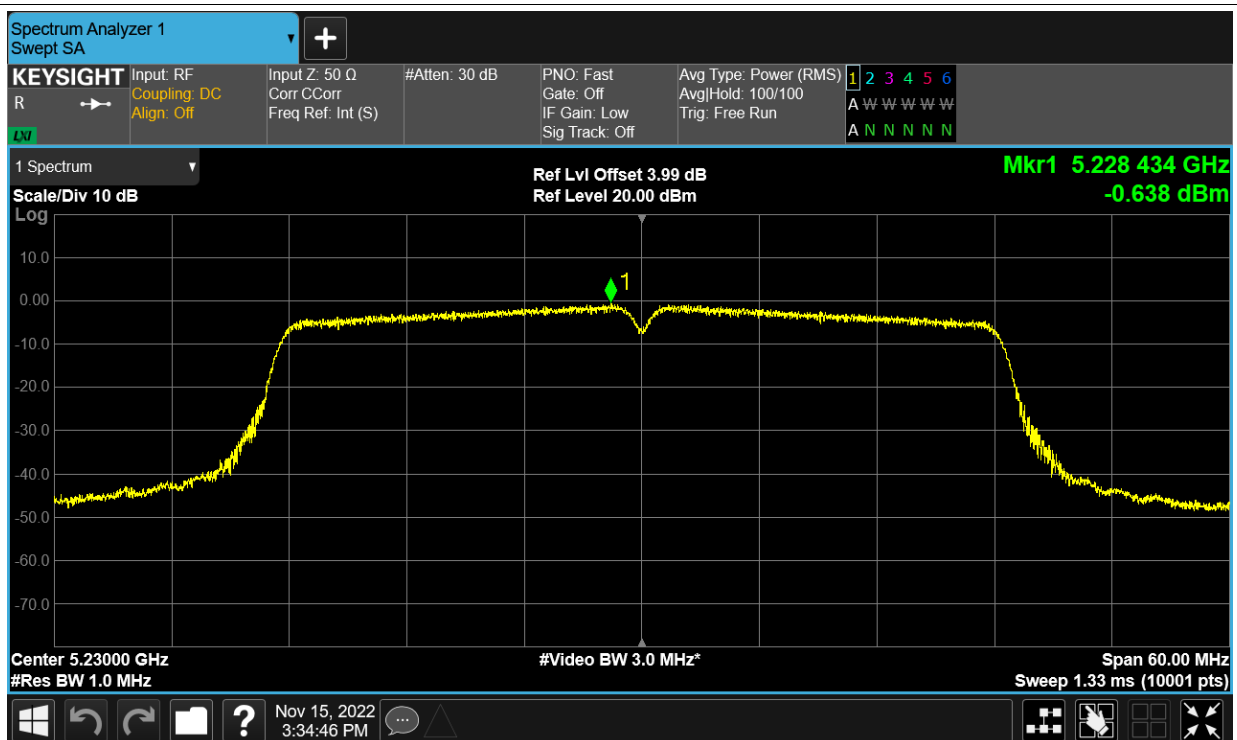
PSD NVNT n40 5230MHz Ant24
