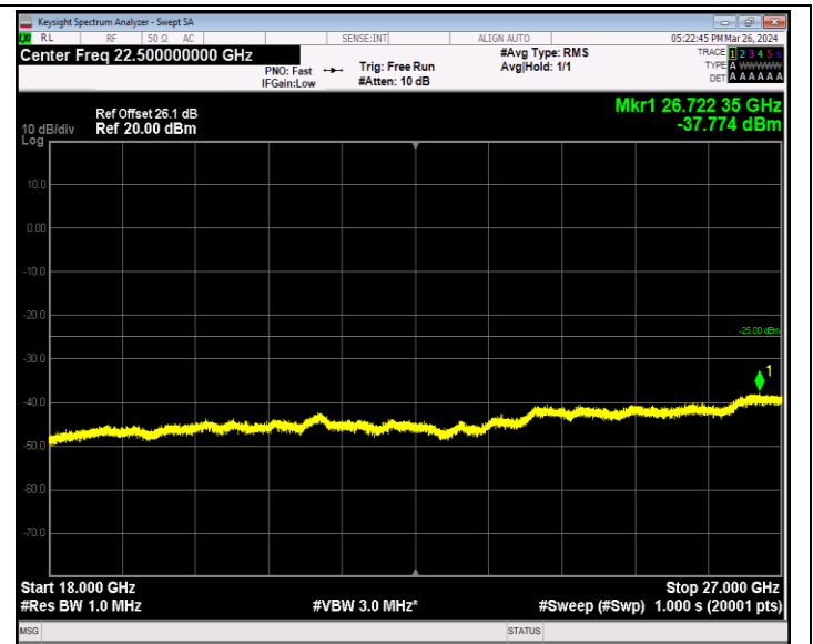
Band7_20MHz_QPSK_20850_1RB#0_18000~27000_18000~27000
