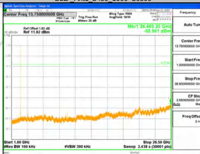
BLE_Ant1_2480_1000~26500
