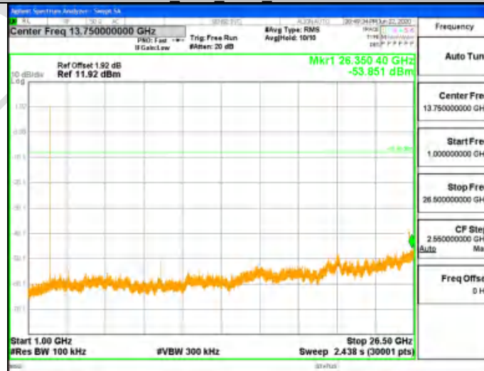
BLE_Ant1_2442_1000~26500
