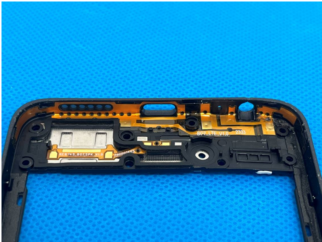
WWAN DIV ANT (PCS1900/WCDMA B2/4/LTE B2/4/7/38/40/41/66)
