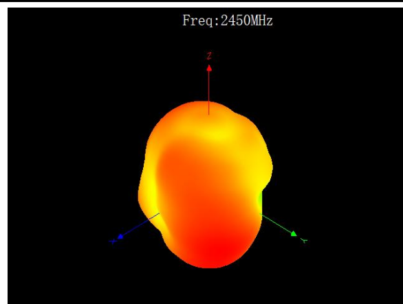
2450Mhz 3D
