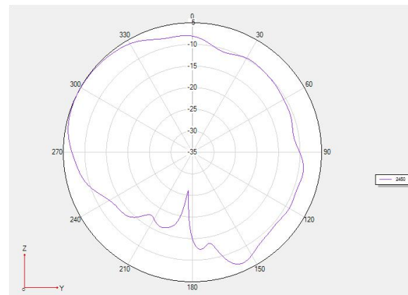
2450Mhz 3D
