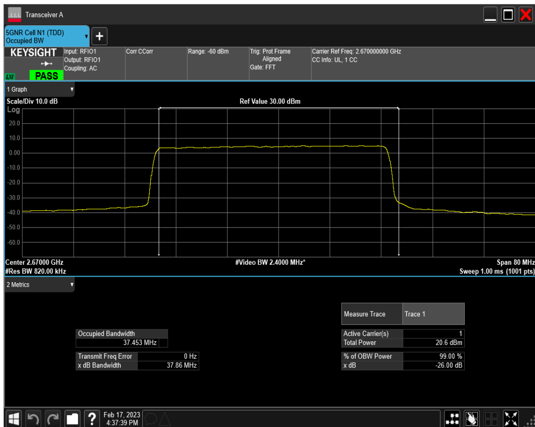
n41 SCS=30kHz CP_QPSK BW=40MHz Channel=534000 RB=106@0
