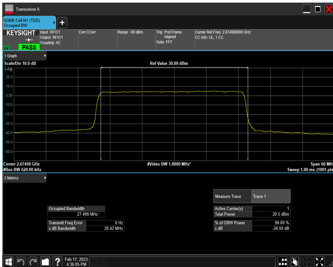
n41 SCS=30kHz CP_QPSK BW=30MHz Channel=534996 RB=78@0
