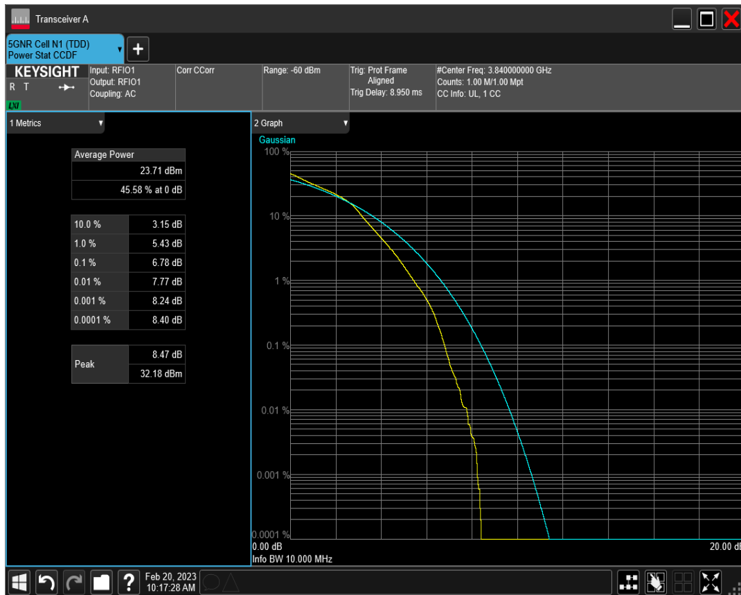
n77(3700-3980) SCS=15kHz DFT_QAM64 BW=10MHz Channel=656000 RB=50@0
