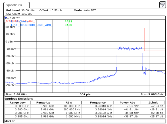
20MHz_15kHz_3970MHz_DFT-s-OFDM QPSK_RB100@0&amp;-35.60 dBm
