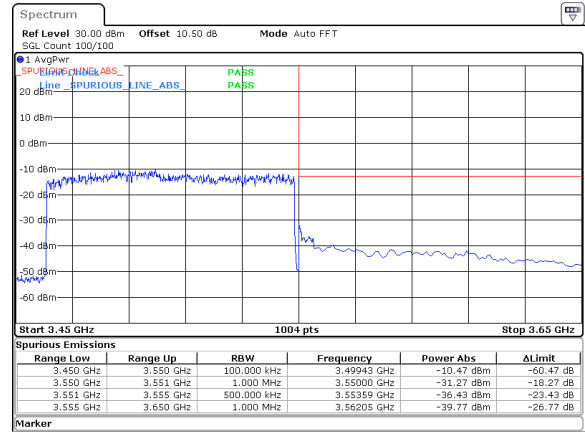
90MHz_30kHz_3505MHz_DFT-s-OFDM QPSK_RB243@0&-31.27 dBm
