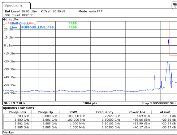
10MHz_30kHz_3795MHz_DFT-s-OFDM QPSK_RB1@23&amp;-33.99 dBm
