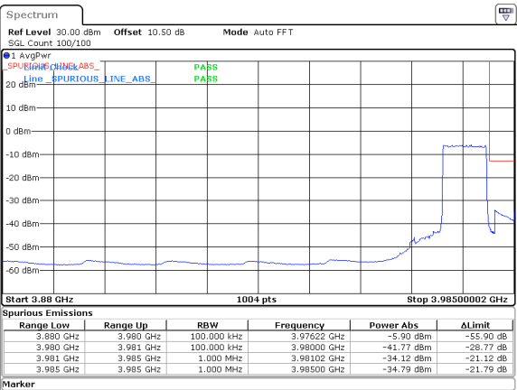
10MHz_15kHz_3975MHz_DFT-s-OFDM QPSK_RB50@0&-34.12 dBm
