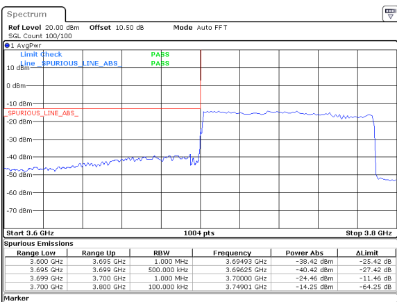
90MHz_30kHz_3745MHz_DFT-s-OFDM QPSK_RB243@0&-24.46 dBm
