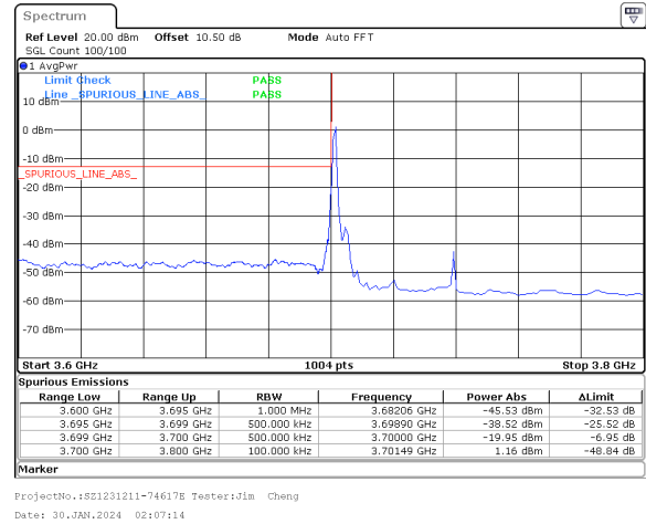
40MHz_30kHz_3720MHz_DFT-s-OFDM QPSK_RB1@0&-19.95 dBm
