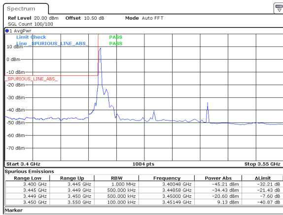
60MHz_30kHz_3480MHz_DFT-s-OFDM QPSK_RB1@0&amp;-20.60 dBm
