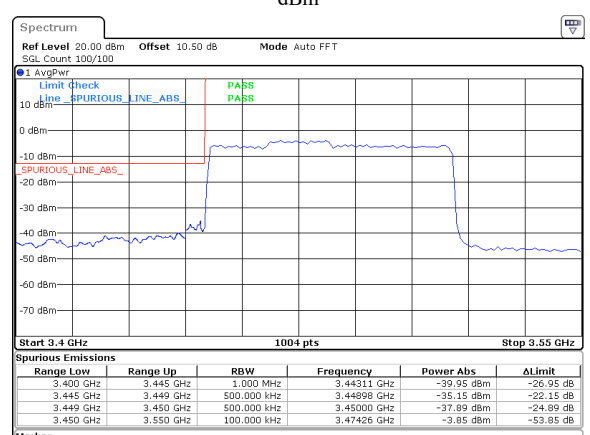
70MHz_30kHz_3485MHz_DFT-s-OFDM QPSK_RB180@0&amp;-35.15 dBm
