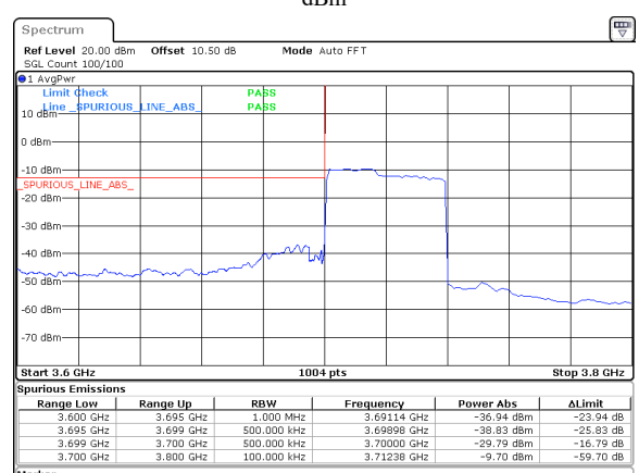
40MHz_15kHz_3720MHz_DFT-s-OFDM QPSK_RB216@0&amp;-29.79 dBm
