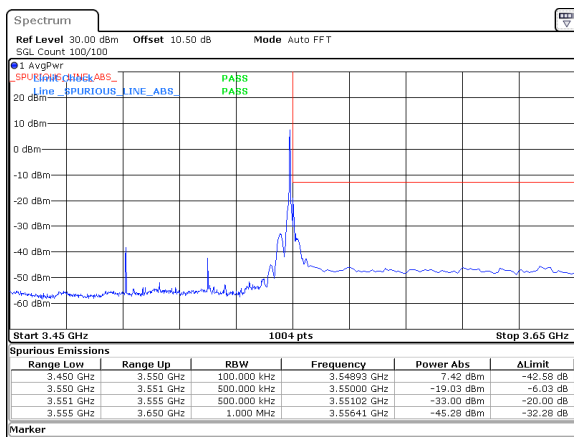
60MHz_30kHz_3520MHz_DFT-s-OFDM QPSK_RB1@161&amp;-19.03 dBm
