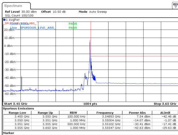
80MHz_30kHz_3510MHz_DFT-s-OFDM QPSK_RB1@216&amp;-14.07 dBm
