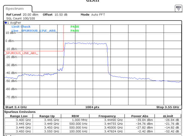
40MHz_30kHz_3470MHz_DFT-s-OFDM QPSK_RB100@0&amp;-27.82 dBm
