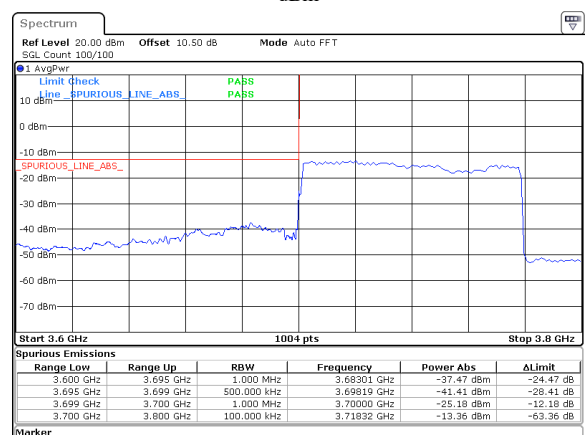
80MHz_30kHz_3740MHz_DFT-s-OFDM QPSK_RB216@0&amp;-25.18 dBm
