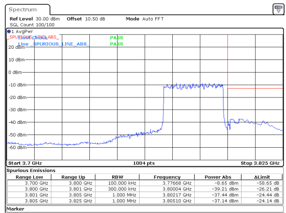
30MHz_30kHz_3785MHz_DFT-s-OFDM QPSK_RB75@0&amp;-37.14 dBm
