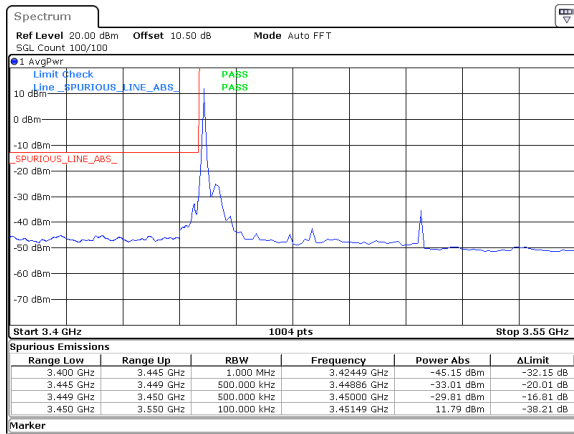
60MHz_30kHz_3480MHz_DFT-s-OFDM QPSK_RB1@0&amp;-29.81 dBm
