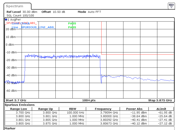
80MHz_30kHz_3760MHz_DFT-s-OFDM QPSK_RB216@0&amp;-38.64 dBm
