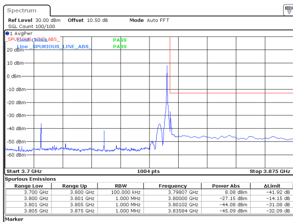
80MHz_30kHz_3760MHz_DFT-s-OFDM QPSK_RB1@216&amp;-27.15 dBm
