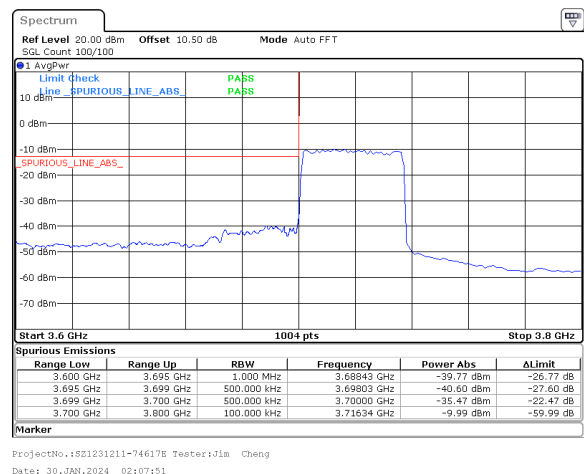
40MHz_30kHz_3720MHz_DFT-s-OFDM QPSK_RB100@0&-35.47 dBm
