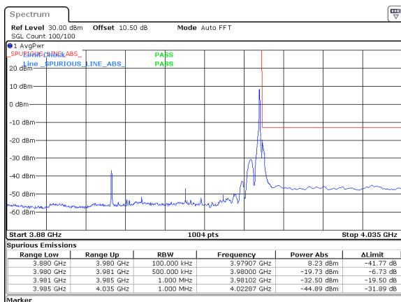
60MHz_30kHz_3950MHz_DFT-s-OFDM QPSK_RB1@161&amp;-19.73 dBm
