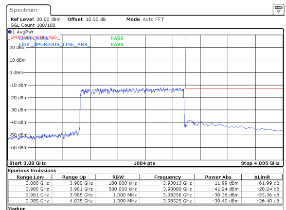
60MHz_30kHz_3950MHz_DFT-s-OFDM QPSK_RB162@0&amp;-38.36 dBm
