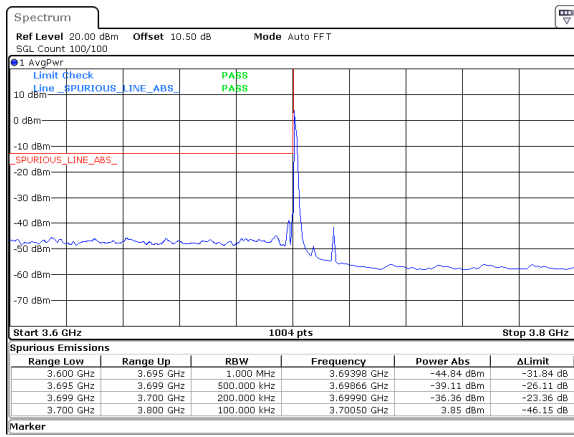
15MHz_30kHz_3707.5MHz_DFT-s-OFDM QPSK_RB1@0&amp;-36.36 dBm
