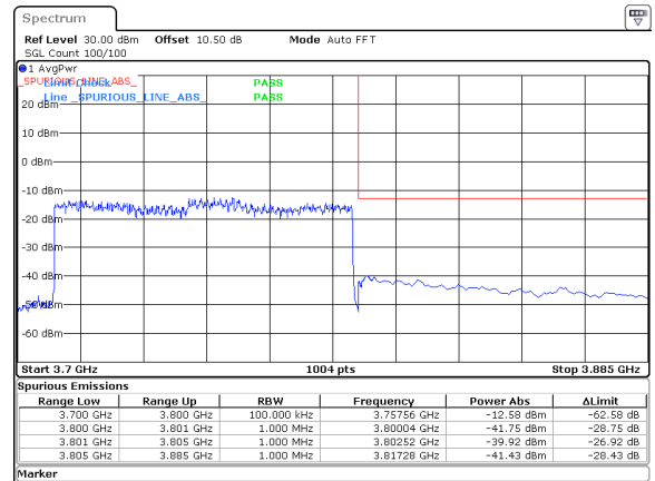
90MHz_30kHz_3755MHz_DFT-s-OFDM QPSK_RB243@0&amp;-39.92 dBm
