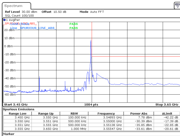
60MHz_30kHz_3520MHz_DFT-s-OFDM QPSK_RB1@161&amp;-30.39 dBm
