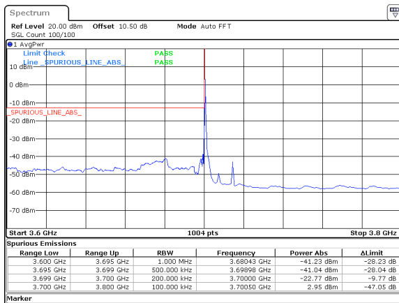
15MHz_15kHz_3707.5MHz_DFT-s-OFDM QPSK_RB1@0&amp;-22.77 dBm
