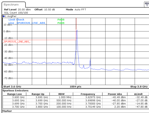
20MHz_30kHz_3710MHz_DFT-s-OFDM QPSK_RB1@0&amp;-27.85 dBm
