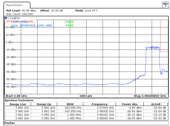
10MHz_30kHz_3975MHz_DFT-s-OFDM QPSK_RB24@0&amp;-36.15 dBm
