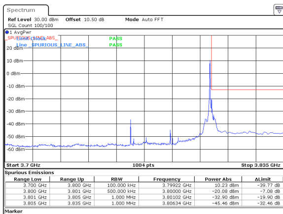
40MHz_15kHz_3780MHz_DFT-s-OFDM QPSK_RB1@215&amp;-20.08 dBm
