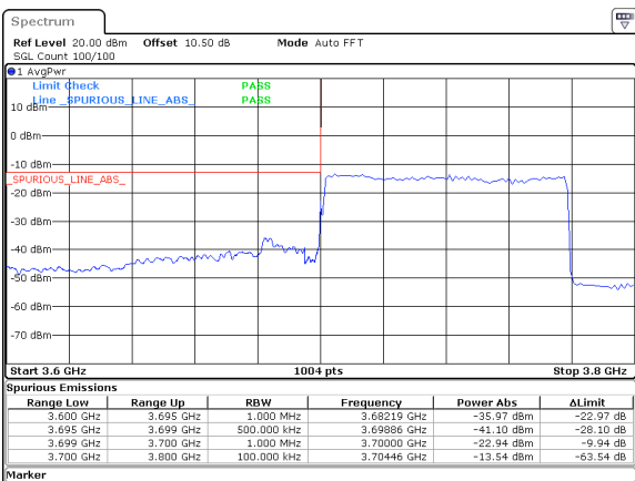
80MHz_30kHz_3740MHz_DFT-s-OFDM QPSK_RB216@0&-22.94 dBm
