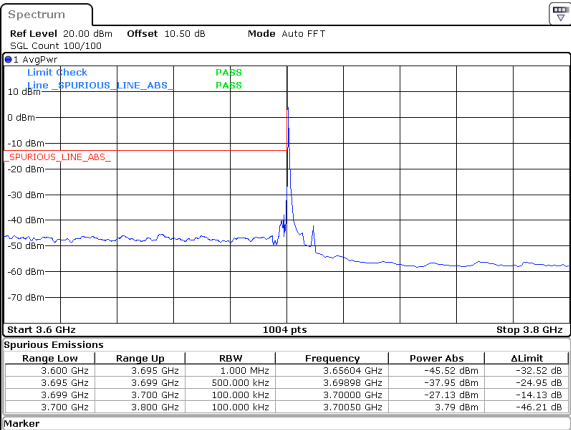
10MHz_15kHz_3705MHz_DFT-s-OFDM QPSK_RB1@0&-27.13 dBm
