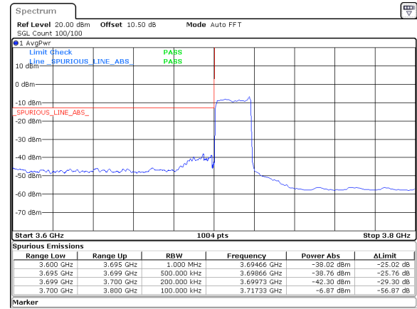
20MHz_15kHz_3710MHz_DFT-s-OFDM QPSK_RB100@0&-38.02 dBm
