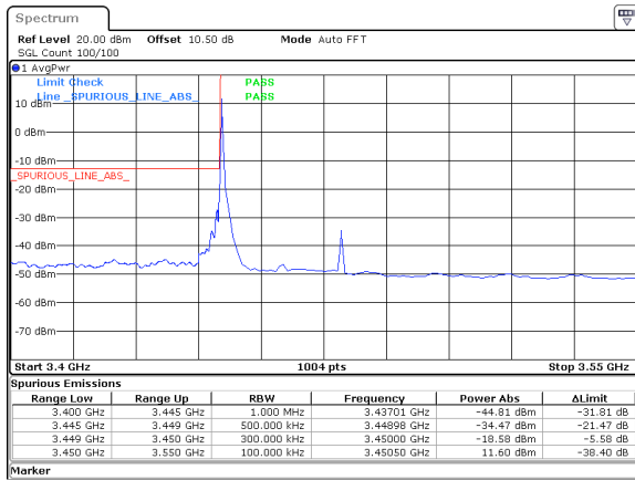
30MHz_15kHz_3465MHz_DFT-s-OFDM QPSK_RB1@0&amp;-18.58 dBm
