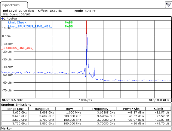
10MHz_30kHz_3705MHz_DFT-s-OFDM QPSK_RB1@0&-38.07 dBm
