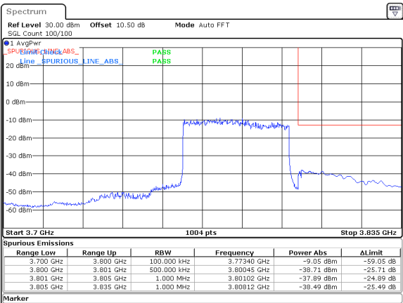
40MHz_30kHz_3780MHz_DFT-s-OFDM QPSK_RB100@0&-37.89 dBm
