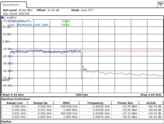
90MHz_30kHz_3505MHz_DFT-s-OFDM QPSK_RB243@0&-33.84 dBm
