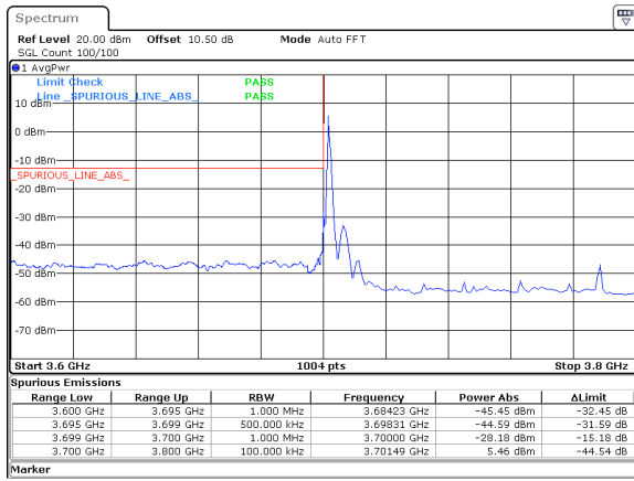
90MHz_30kHz_3745MHz_DFT-s-OFDM QPSK_RB1@0&amp;-28.18 dBm
