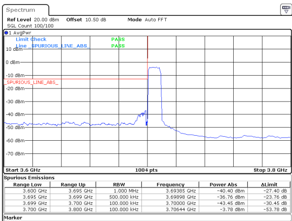
10MHz_15kHz_3705MHz_DFT-s-OFDM QPSK_RB50@0&-36.76 dBm
