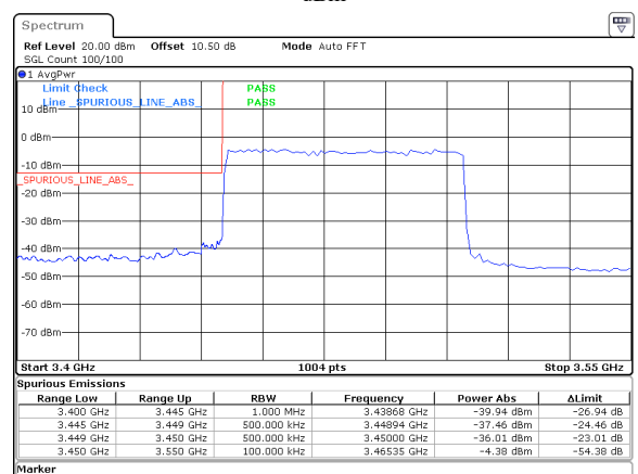
60MHz_30kHz_3480MHz_DFT-s-OFDM QPSK_RB162@0&amp;-36.01 dBm
