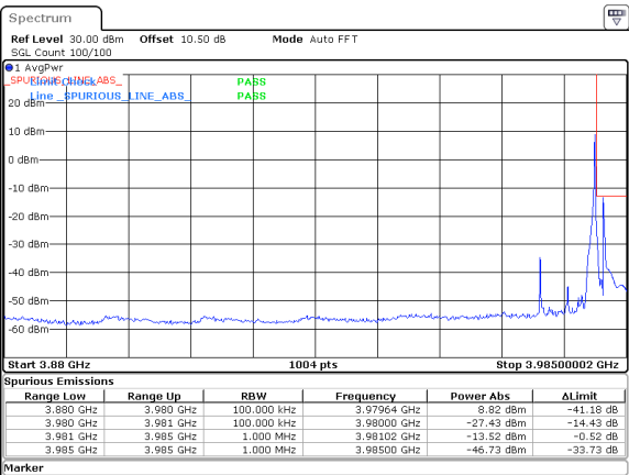
10MHz_15kHz_3975MHz_DFT-s-OFDM QPSK_RB1@51&-13.52 dBm
