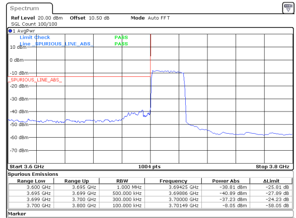
25MHz_30kHz_3712.5MHz_DFT-s-OFDM QPSK_RB64@0&amp;-37.23 dBm
