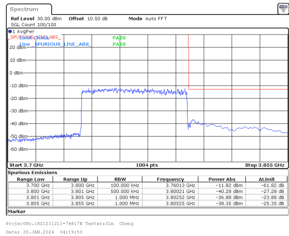
60MHz_30kHz_3770MHz_DFT-s-OFDM QPSK_RB162@0&-36.88 dBm
