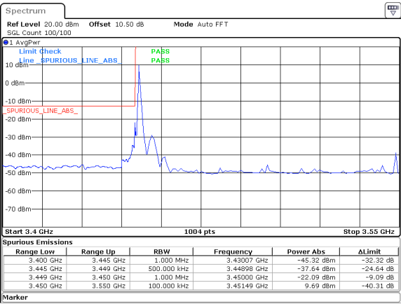
100MHz_30kHz_3500MHz_DFT-s-OFDM QPSK_RB1@0&-22.09 dBm
