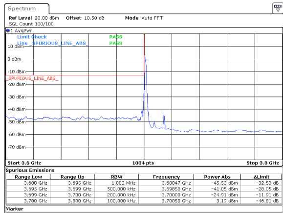
15MHz_30kHz_3707.5MHz_DFT-s-OFDM QPSK_RB1@0&-24.91 dBm
