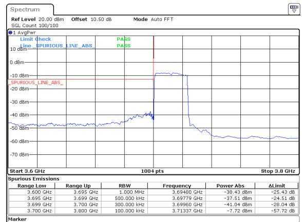
25MHz_15kHz_3712.5MHz_DFT-s-OFDM QPSK_RB128@0&amp;-37.51 dBm
