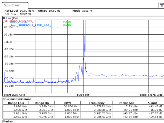
100MHz_30kHz_3930MHz_DFT-s-OFDM QPSK_RB1@272&amp;-29.31 dBm
