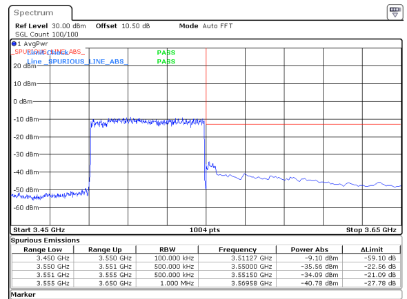
60MHz_30kHz_3520MHz_DFT-s-OFDM QPSK_RB162@0&amp;-34.09 dBm
