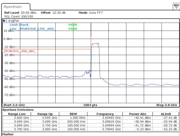
10MHz_30kHz_3705MHz_DFT-s-OFDM QPSK_RB24@0&-38.94 dBm
