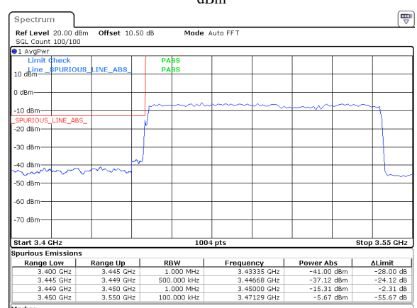
90MHz_30kHz_3495MHz_DFT-s-OFDM QPSK_RB243@0&amp;-15.31 dBm
