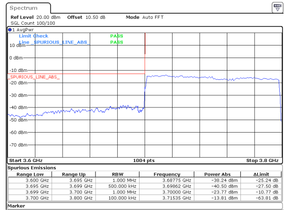
100MHz_30kHz_3750MHz_DFT-s-OFDM QPSK_RB270@0&amp;-23.77 dBm
