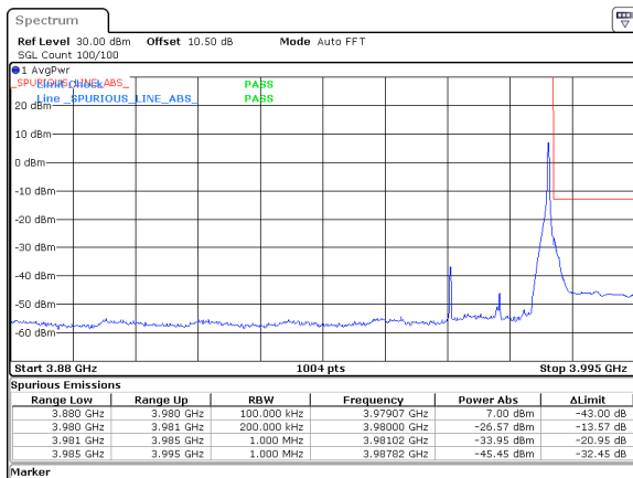
20MHz_30kHz_3970MHz_DFT-s-OFDM QPSK_RB1@50&amp;-26.57 dBm
