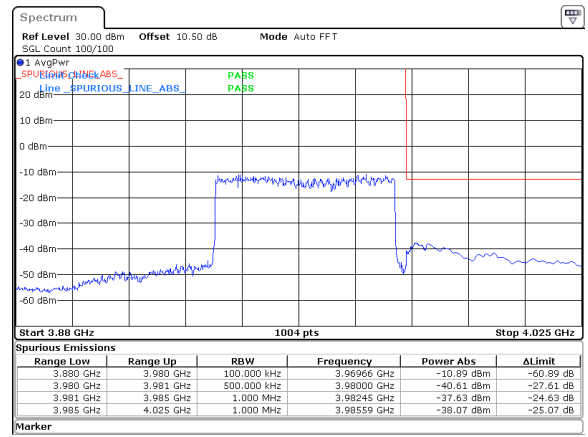
50MHz_30kHz_3955MHz_DFT-s-OFDM QPSK_RB128@0&amp;-37.63 dBm
