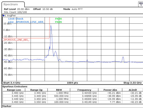
80MHz_30kHz_3490MHz_DFT-s-OFDM QPSK_RB1@0&amp;-24.99 dBm
