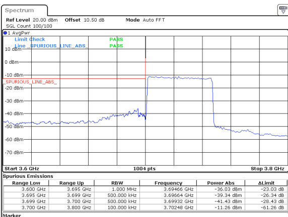
50MHz_30kHz_3725MHz_DFT-s-OFDM QPSK_RB128@0&-36.03 dBm
