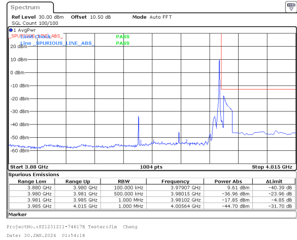
40MHz_15kHz_3960MHz_DFT-s-OFDM QPSK_RB1@215&-17.85 dBm
