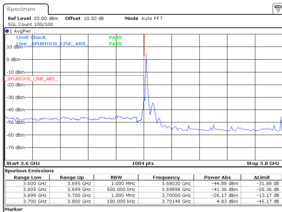
100MHz_30kHz_3750MHz_DFT-s-OFDM QPSK_RB1@0&amp;-26.17 dBm
