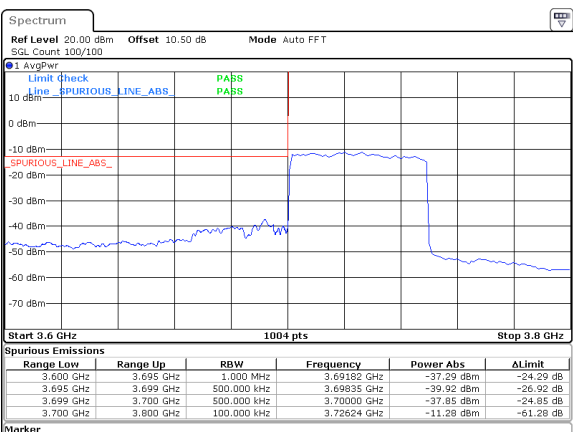
50MHz_15kHz_3725MHz_DFT-s-OFDM QPSK_RB270@0&-37.29 dBm
