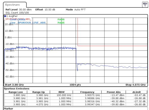
100MHz_30kHz_3930MHz_DFT-s-OFDM QPSK_RB270@0&amp;-39.80 dBm
