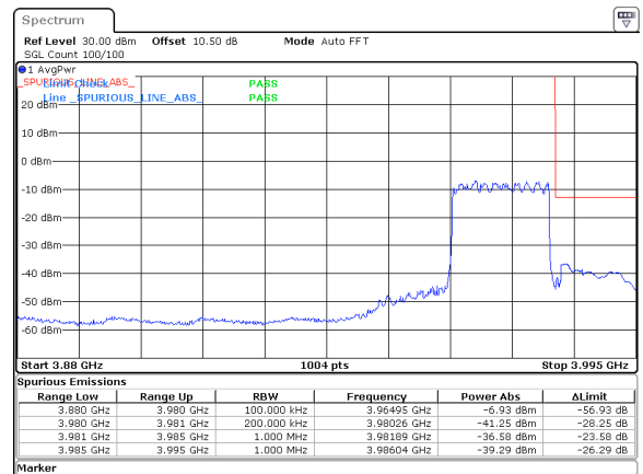
20MHz_30kHz_3970MHz_DFT-s-OFDM QPSK_RB50@0&amp;-36.58 dBm
