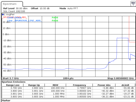
10MHz_15kHz_3795MHz_DFT-s-OFDM QPSK_RB50@0&-32.27 dBm
