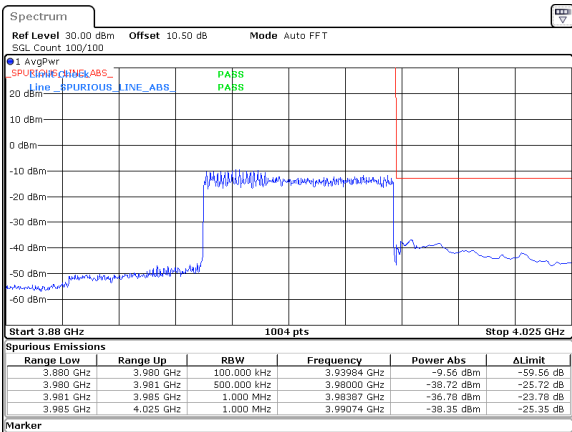
50MHz_15kHz_3955MHz_DFT-s-OFDM QPSK_RB270@0&-36.78 dBm
