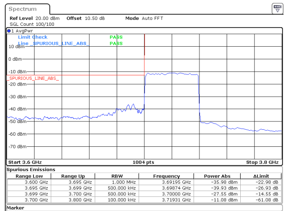
40MHz_15kHz_3720MHz_DFT-s-OFDM QPSK_RB216@0&amp;-27.55 dBm
