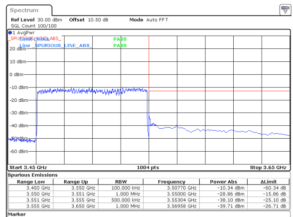
80MHz_30kHz_3510MHz_DFT-s-OFDM QPSK_RB216@0&amp;-28.86 dBm
