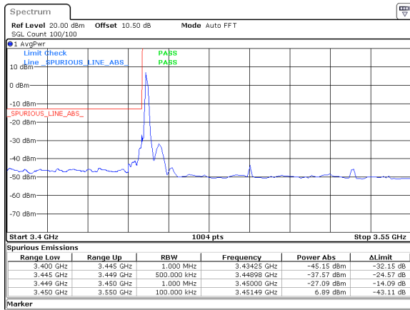
80MHz_30kHz_3490MHz_DFT-s-OFDM QPSK_RB1@0&amp;-27.09 dBm
