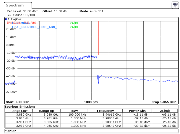
90MHz_30kHz_3935MHz_DFT-s-OFDM QPSK_RB243@0&amp;-39.10 dBm
