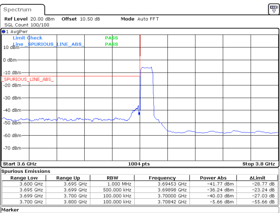
10MHz_15kHz_3705MHz_DFT-s-OFDM QPSK_RB50@0&-36.24 dBm
