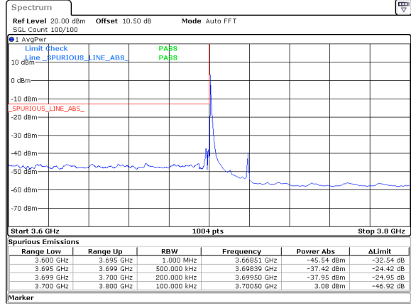
20MHz_15kHz_3710MHz_DFT-s-OFDM QPSK_RB1@0&-37.42 dBm
