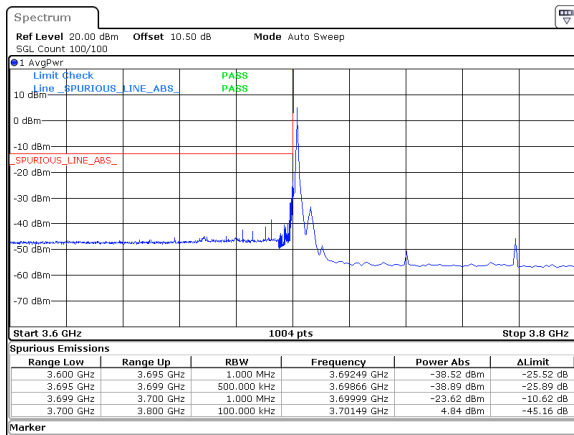
80MHz_30kHz_3740MHz_DFT-s-OFDM QPSK_RB1@0&amp;-23.62 dBm
