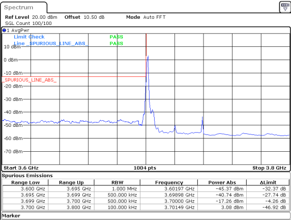
40MHz_30kHz_3720MHz_DFT-s-OFDM QPSK_RB1@0&-17.26 dBm
