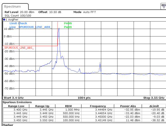
40MHz_30kHz_3470MHz_DFT-s-OFDM QPSK_RB1@0&amp;-22.03 dBm
