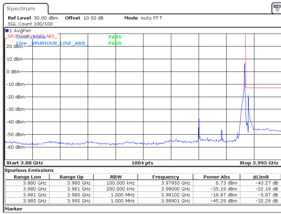
20MHz_15kHz_3970MHz_DFT-s-OFDM QPSK_RB1@105&amp;-18.87 dBm
