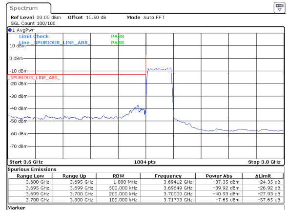
20MHz_30kHz_3710MHz_DFT-s-OFDM QPSK_RB50@0&amp;-37.35 dBm
