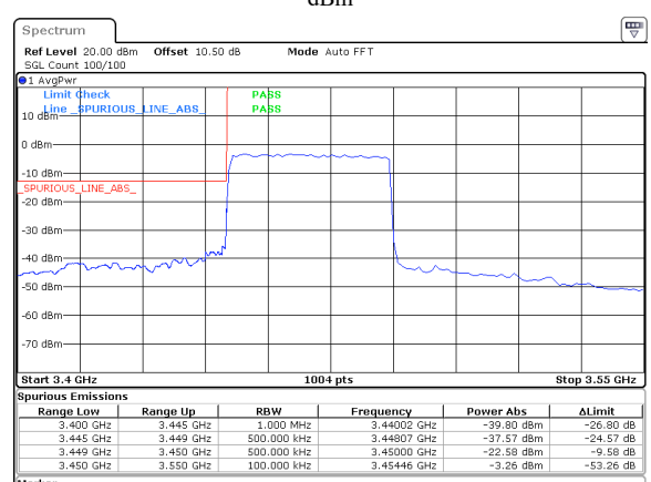
40MHz_15kHz_3470MHz_DFT-s-OFDM QPSK_RB216@0&amp;-22.58 dBm
