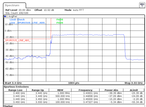
80MHz_30kHz_3490MHz_DFT-s-OFDM QPSK_RB216@0&amp;-15.20 dBm
