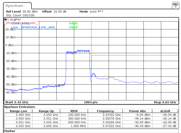
30MHz_30kHz_3535MHz_DFT-s-OFDM QPSK_RB75@0&amp;-35.09 dBm
