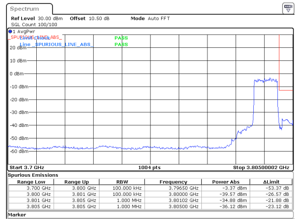
10MHz_30kHz_3795MHz_DFT-s-OFDM QPSK_RB24@0&amp;-34.88 dBm
