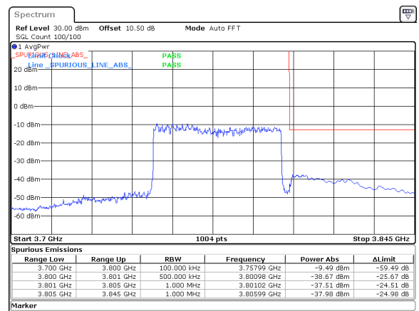
50MHz_30kHz_3775MHz_DFT-s-OFDM QPSK_RB128@0&amp;-37.51 dBm
