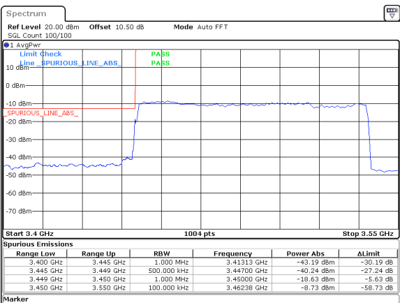
90MHz_30kHz_3495MHz_DFT-s-OFDM QPSK_RB243@0&-18.63 dBm
