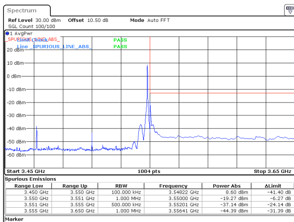
80MHz_30kHz_3510MHz_DFT-s-OFDM QPSK_RB1@216&amp;-19.27 dBm
