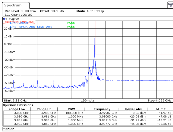
90MHz_30kHz_3935MHz_DFT-s-OFDM QPSK_RB1@244&amp;-20.08 dBm
