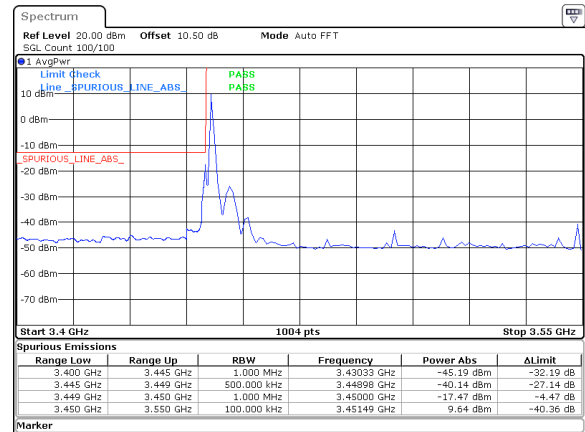
100MHz_30kHz_3500MHz_DFT-s-OFDM QPSK_RB1@0&-17.47 dBm
