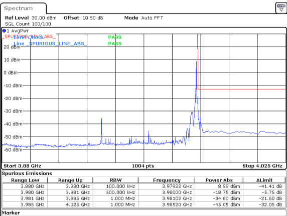
50MHz_15kHz_3955MHz_DFT-s-OFDM QPSK_RB1@269&-18.75 dBm
