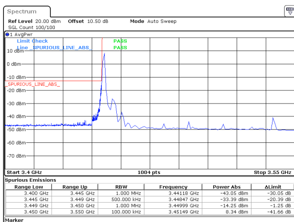
90MHz_30kHz_3495MHz_DFT-s-OFDM QPSK_RB1@0&amp;-14.25 dBm
