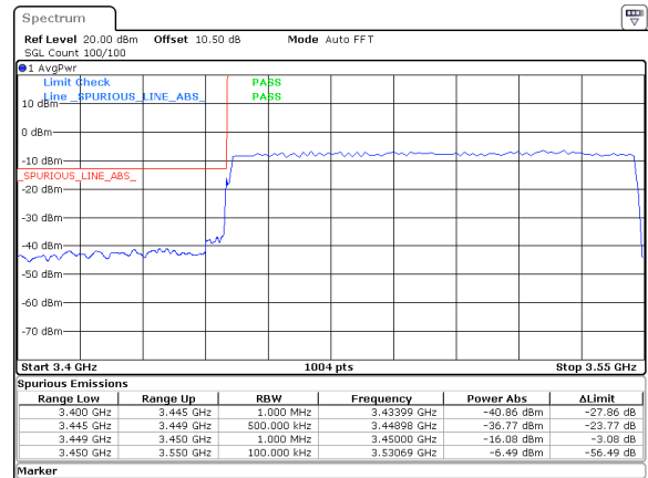
100MHz_30kHz_3500MHz_DFT-s-OFDM QPSK_RB270@0&-16.08 dBm
