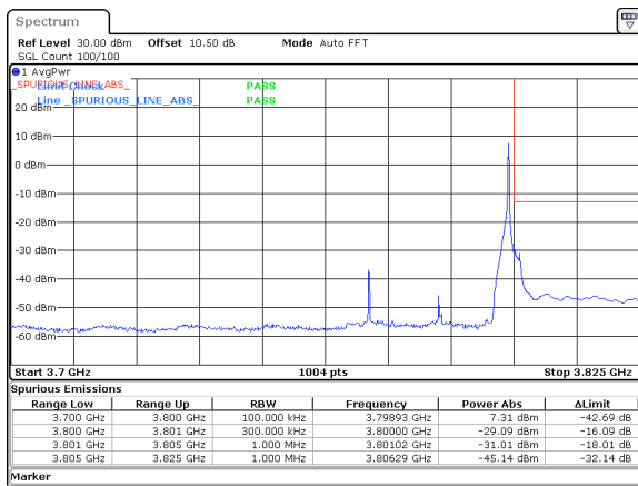
30MHz_30kHz_3785MHz_DFT-s-OFDM QPSK_RB1@77&amp;-29.09 dBm
