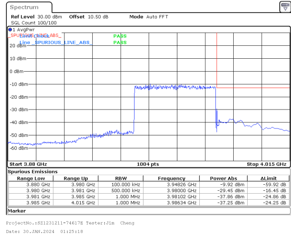
40MHz_15kHz_3960MHz_DFT-s-OFDM QPSK_RB216@0&-29.45 dBm
