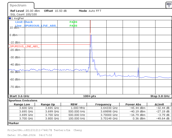
60MHz_30kHz_3730MHz_DFT-s-OFDM QPSK_RB1@0&-16.79 dBm
