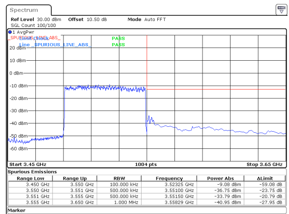
60MHz_30kHz_3520MHz_DFT-s-OFDM QPSK_RB162@0&amp;-33.79 dBm
