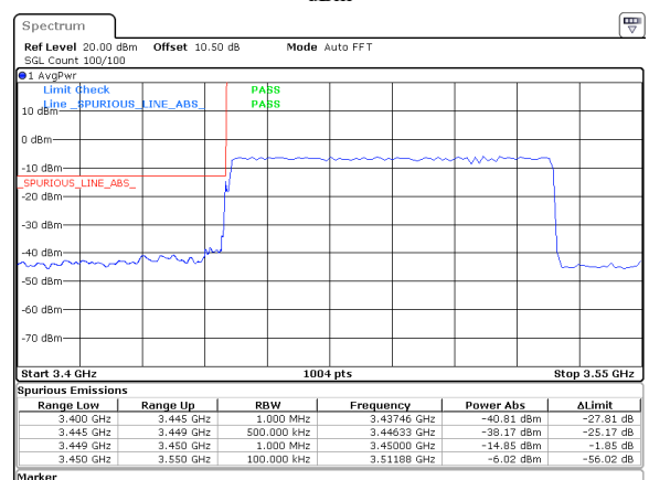
80MHz_30kHz_3490MHz_DFT-s-OFDM QPSK_RB216@0&amp;-14.85 dBm
