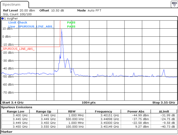
90MHz_30kHz_3495MHz_DFT-s-OFDM QPSK_RB1@0&-22.58 dBm
