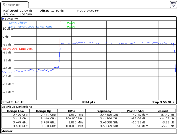
100MHz_30kHz_3500MHz_DFT-s-OFDM QPSK_RB270@0&-16.35 dBm
