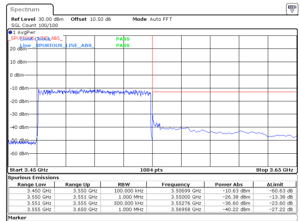
80MHz_30kHz_3510MHz_DFT-s-OFDM QPSK_RB216@0&amp;-26.38 dBm
