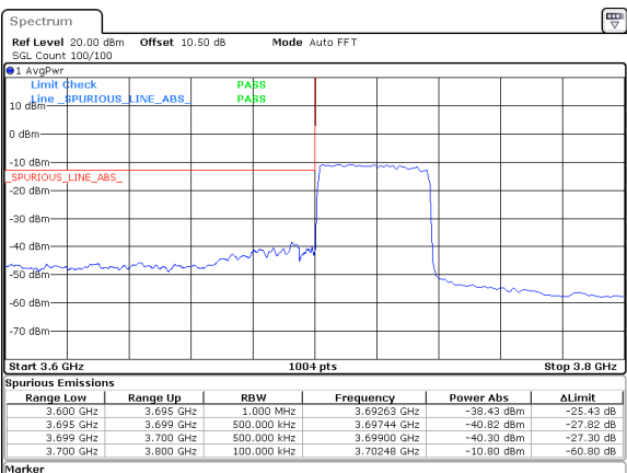
40MHz_30kHz_3720MHz_DFT-s-OFDM QPSK_RB100@0&-38.43 dBm
