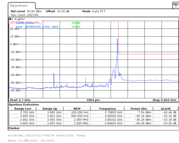
60MHz_30kHz_3770MHz_DFT-s-OFDM QPSK_RB1@161&-36.16 dBm
