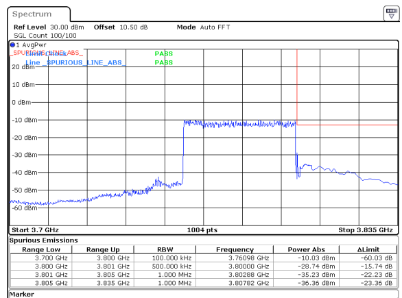
40MHz_15kHz_3780MHz_DFT-s-OFDM QPSK_RB216@0&amp;-28.74 dBm
