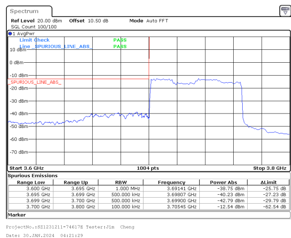
70MHz_30kHz_3735MHz_DFT-s-OFDM QPSK_RB180@0&-38.75 dBm
