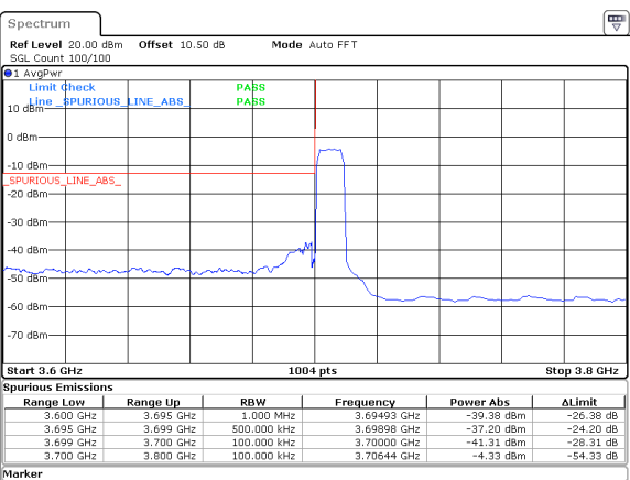
10MHz_30kHz_3705MHz_DFT-s-OFDM QPSK_RB24@0&-37.20 dBm
