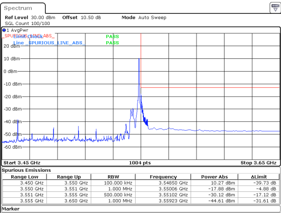
90MHz_30kHz_3505MHz_DFT-s-OFDM QPSK_RB1@244&-17.88 dBm
