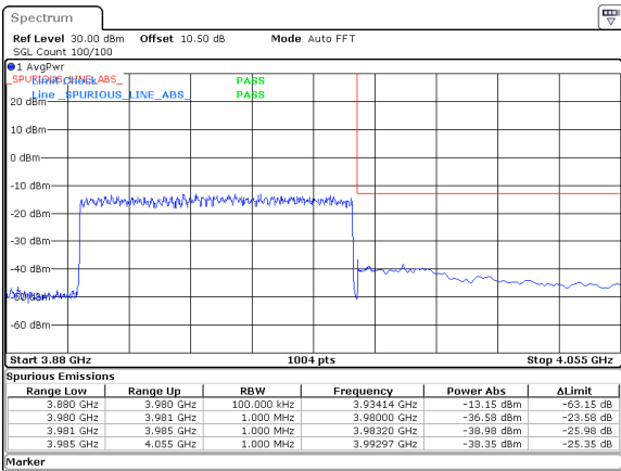
80MHz_30kHz_3940MHz_DFT-s-OFDM QPSK_RB216@0&-36.58 dBm
