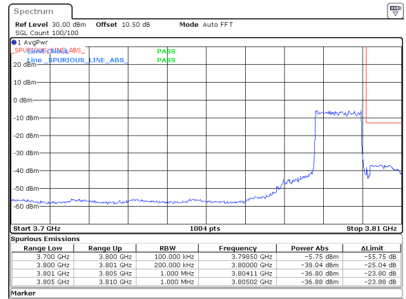
15MHz_30kHz_3792.5MHz_DFT-s-OFDM QPSK_RB36@0&amp;-36.80 dBm
