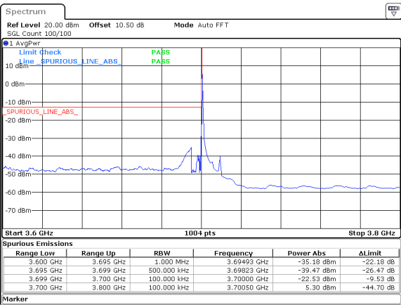
10MHz_30kHz_3705MHz_DFT-s-OFDM QPSK_RB1@0&-22.53 dBm
