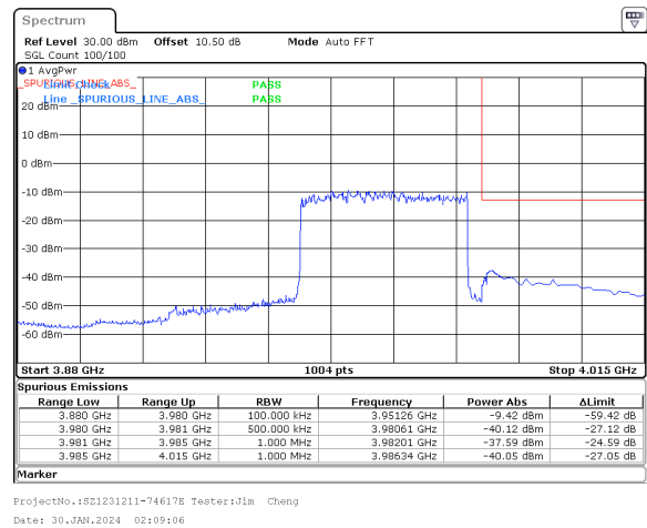
40MHz_30kHz_3960MHz_DFT-s-OFDM QPSK_RB100@0&-37.59 dBm
