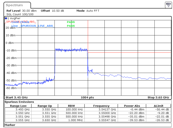
40MHz_15kHz_3530MHz_DFT-s-OFDM QPSK_RB216@0&amp;-22.20 dBm
