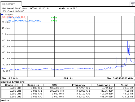
10MHz_15kHz_3795MHz_DFT-s-OFDM QPSK_RB1@51&-17.08 dBm
