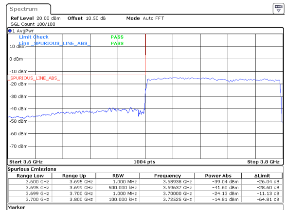
100MHz_30kHz_3750MHz_DFT-s-OFDM QPSK_RB270@0&amp;-24.13 dBm
