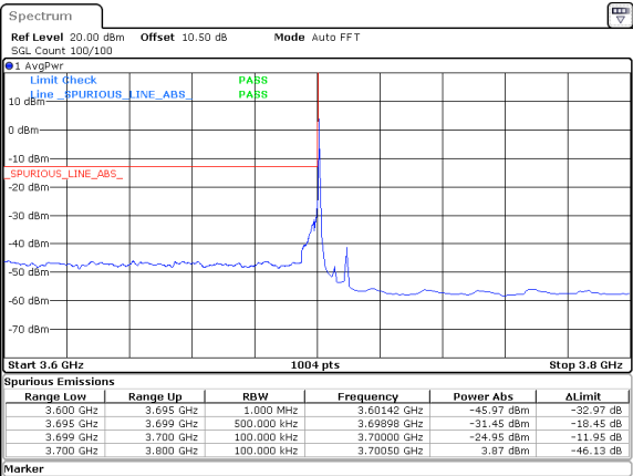
10MHz_15kHz_3705MHz_DFT-s-OFDM QPSK_RB1@0&-24.95 dBm
