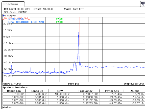
90MHz_30kHz_3755MHz_DFT-s-OFDM QPSK_RB1@244&amp;-29.55 dBm
