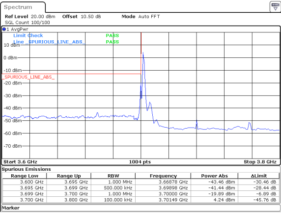
80MHz_30kHz_3740MHz_DFT-s-OFDM QPSK_RB1@0&-19.89 dBm
