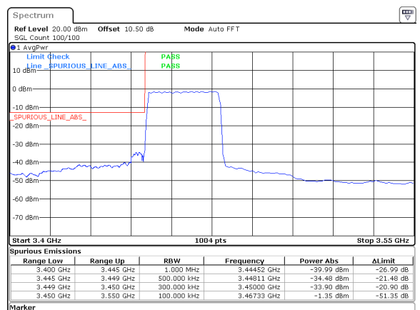
30MHz_30kHz_3465MHz_DFT-s-OFDM QPSK_RB75@0&amp;-33.90 dBm
