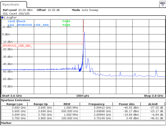
90MHz_30kHz_3745MHz_DFT-s-OFDM QPSK_RB1@0&-19.84 dBm
