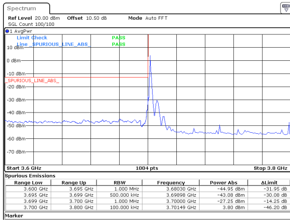
100MHz_30kHz_3750MHz_DFT-s-OFDM QPSK_RB1@0&amp;-27.25 dBm
