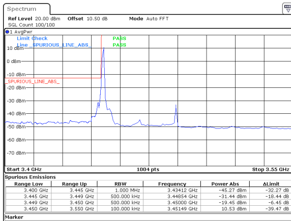
40MHz_30kHz_3470MHz_DFT-s-OFDM QPSK_RB1@0&amp;-19.45 dBm
