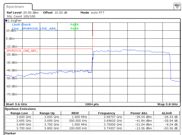
90MHz_30kHz_3745MHz_DFT-s-OFDM QPSK_RB243@0&amp;-21.04 dBm
