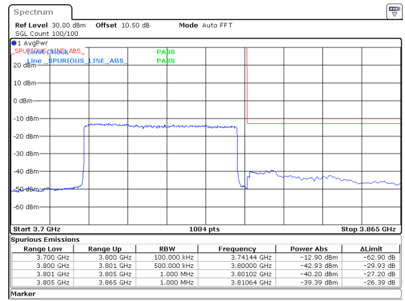
70MHz_30kHz_3765MHz_DFT-s-OFDM QPSK_RB180@0&amp;-39.39 dBm
