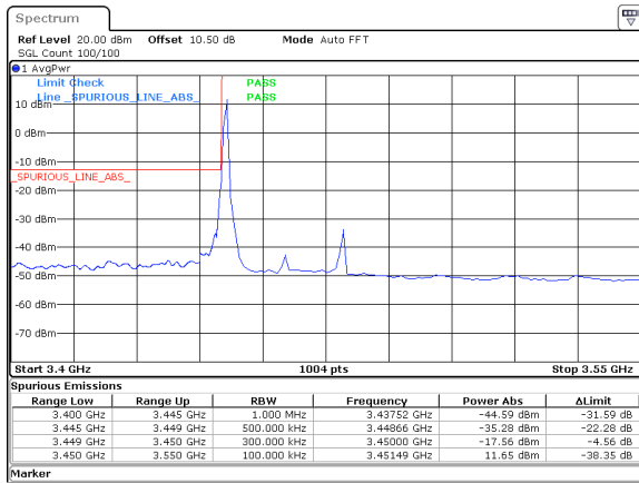
30MHz_30kHz_3465MHz_DFT-s-OFDM QPSK_RB1@0&amp;-17.56 dBm
