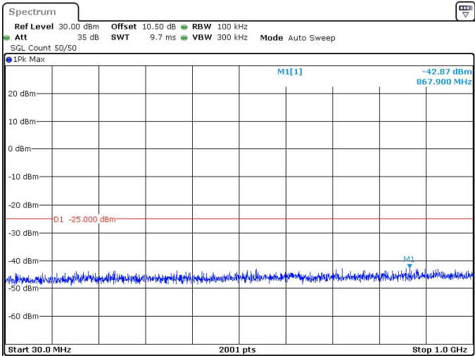
15MHz_30kHz_2595MHz_DFT-s-OFDM QPSK_RB1@0 -42.87 dBm
