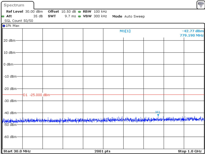
15MHz_30kHz_2595MHz_DFT-s-OFDM QPSK_RB1@37 -42.77 dBm
