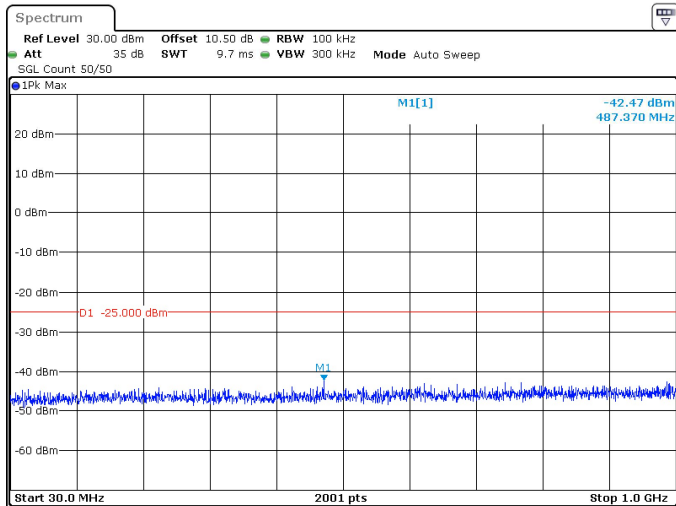
10MHz_30kHz_2501.01MHz_DFT-s-OFDM QPSK_RB1@0 -42.47 dBm
