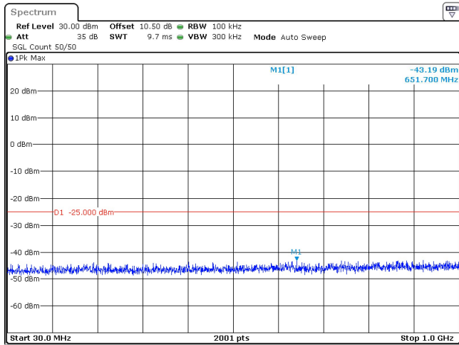
10MHz_30kHz_2501.01MHz_DFT-s-OFDM QPSK_RB24@0 -43.19 dBm
