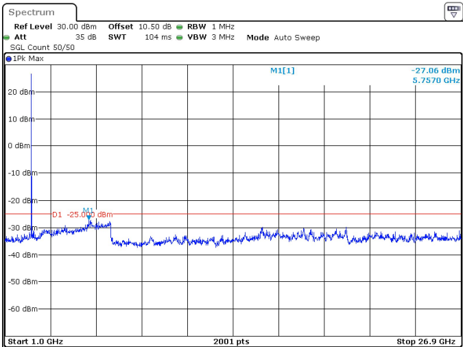
10MHz_30kHz_2501.01MHz_DFT-s-OFDM QPSK_RB1@0 -27.06 dBm
