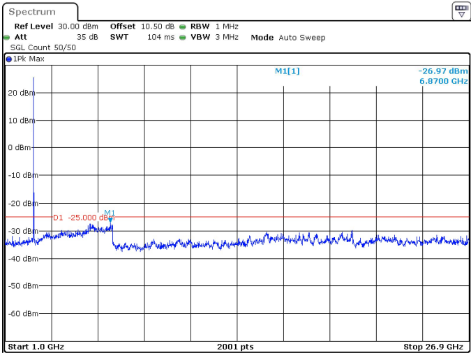
10MHz_30kHz_2592.99MHz_DFT-s-OFDM QPSK_RB1@0 -26.97 dBm
