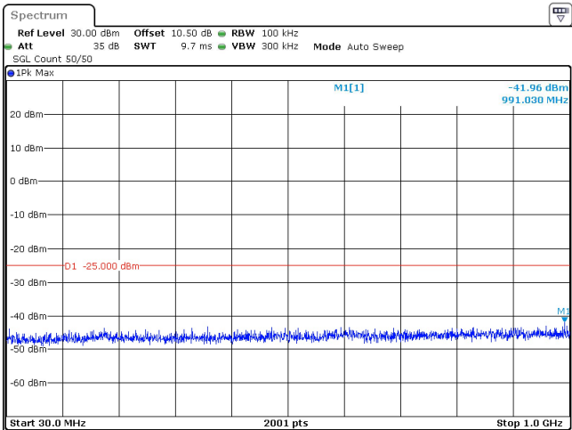
10MHz_30kHz_2685MHz_DFT-s-OFDM QPSK_RB1@23 -41.96 dBm
