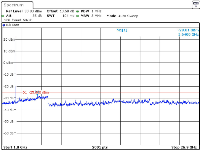
10MHz_30kHz_2685MHz_DFT-s-OFDM QPSK_RB24@0 -28.01 dBm
