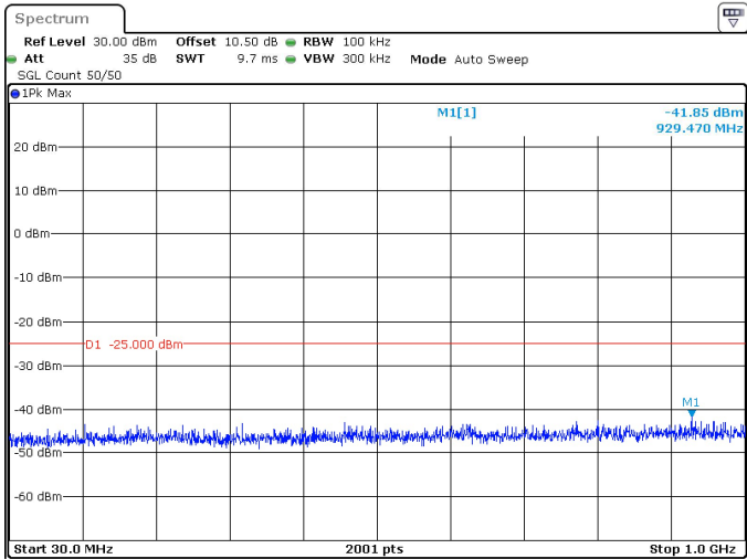
10MHz_30kHz_2685MHz_DFT-s-OFDM QPSK_RB1@0 -41.85 dBm
