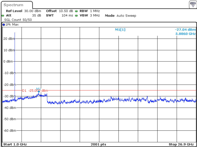
10MHz_30kHz_2685MHz_DFT-s-OFDM QPSK_RB1@0 -27.04 dBm
