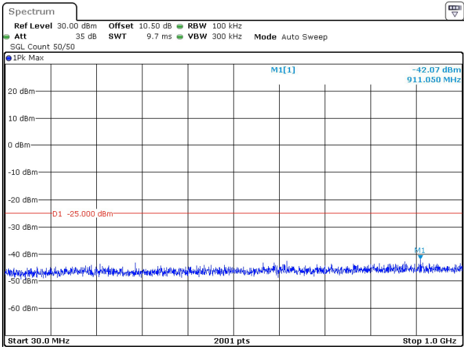
10MHz_30kHz_2592.99MHz_DFT-s-OFDM QPSK_RB24@0 -42.07 dBm
