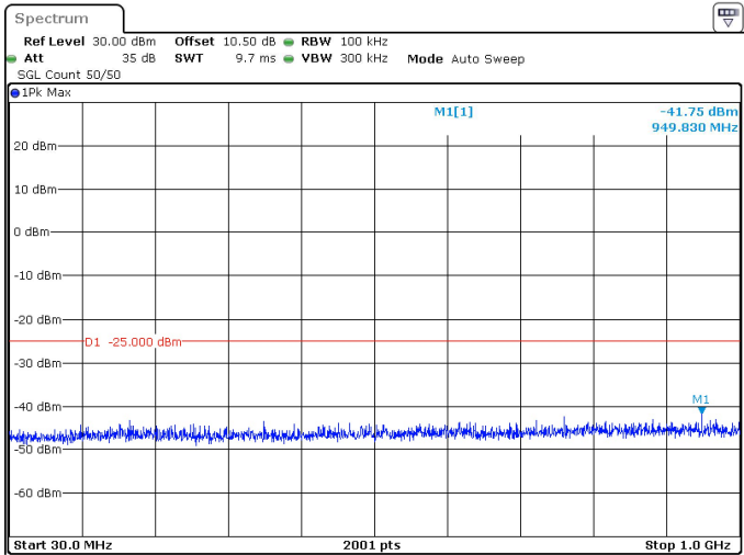
10MHz_30kHz_2592.99MHz_DFT-s-OFDM QPSK_RB1@0 -41.75 dBm
