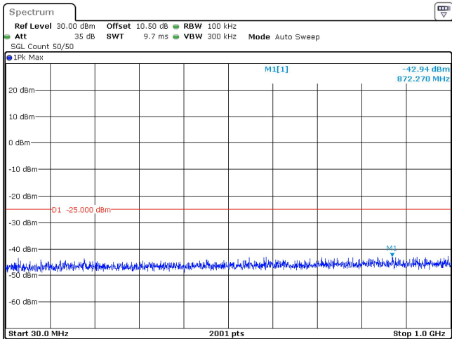
10MHz_30kHz_2685MHz_DFT-s-OFDM QPSK_RB24@0 -42.94 dBm
