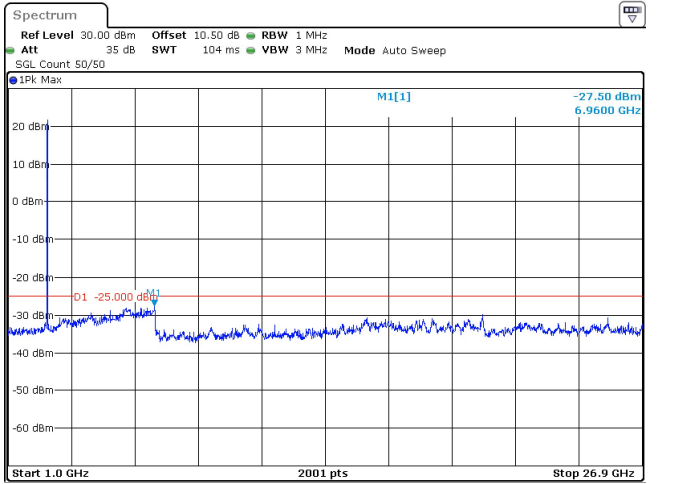
10MHz_30kHz_2592.99MHz_DFT-s-OFDM QPSK_RB24@0 -27.50 dBm
