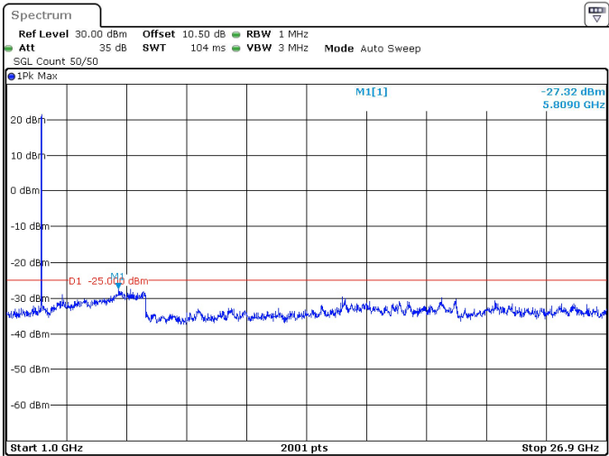
10MHz_30kHz_2501.01MHz_DFT-s-OFDM QPSK_RB24@0 -27.32 dBm
