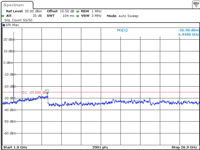
15MHz_30kHz_2503.5MHz_DFT-s-OFDM QPSK_RB1@0 -26.98 dBm
