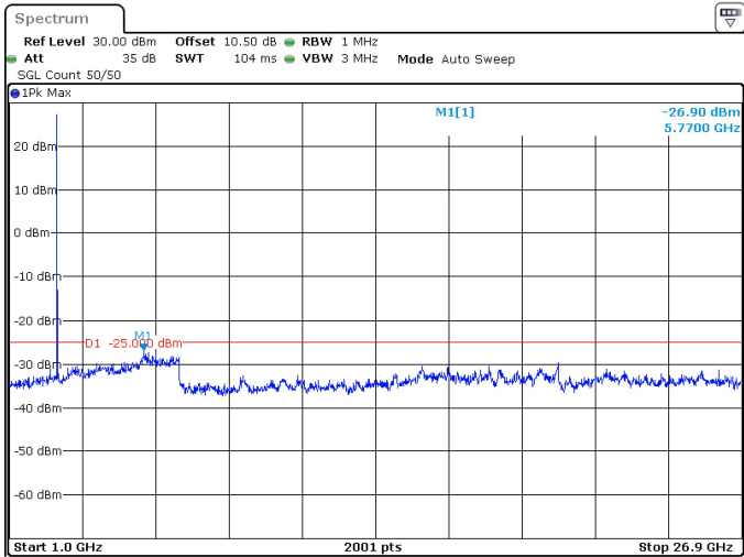
10MHz_30kHz_2685MHz_DFT-s-OFDM QPSK_RB1@23 -26.90 dBm
