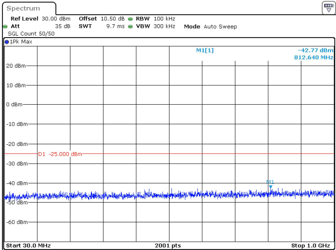
15MHz_30kHz_2682.48MHz_DFT-s-OFDM QPSK_RB1@0 -42.77 dBm
