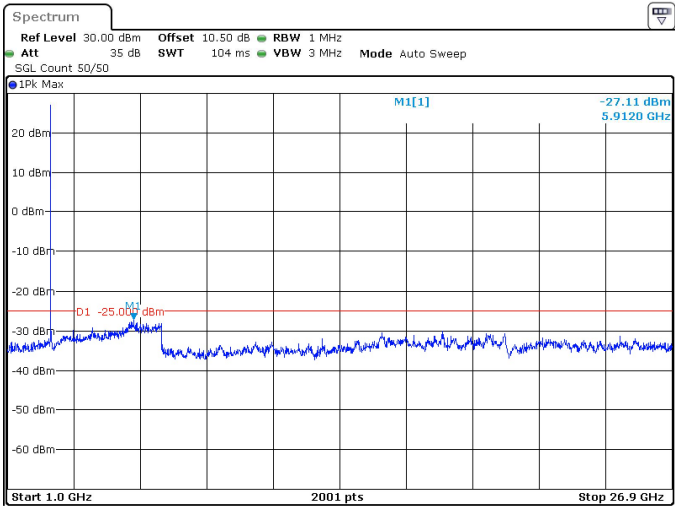
15MHz_30kHz_2682.48MHz_DFT-s-OFDM QPSK_RB1@0 -27.11 dBm
