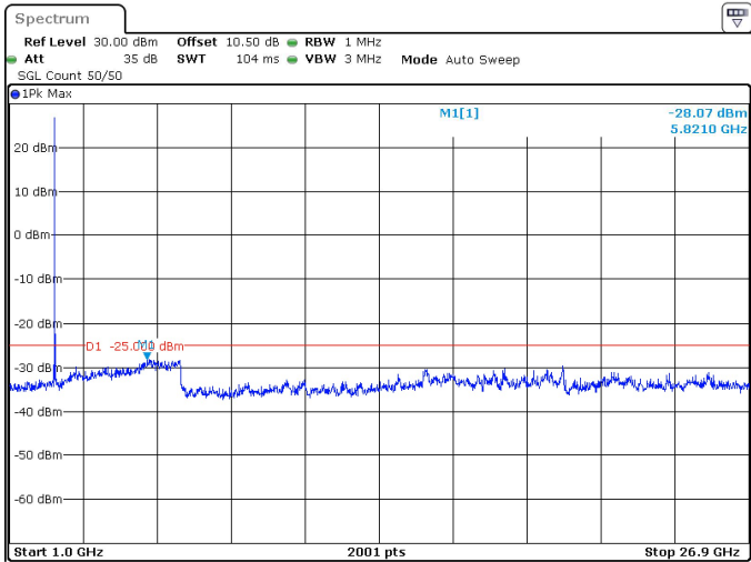
20MHz_30kHz_2592.99MHz_DFT-s-OFDM QPSK_RB1@0 -28.07 dBm
