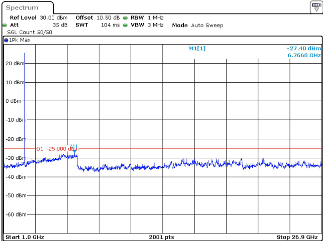
20MHz_30kHz_2679.99MHz_DFT-s-OFDM QPSK_RB1@50 -27.40 dBm
