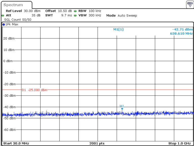
20MHz_30kHz_2506.02MHz_DFT-s-OFDM QPSK_RB50@0 -42.71 dBm
