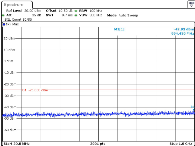
20MHz_30kHz_2592.99MHz_DFT-s-OFDM QPSK_RB50@0 -42.93 dBm
