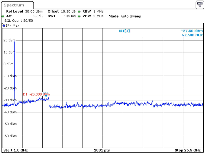
20MHz_30kHz_2592.99MHz_DFT-s-OFDM QPSK_RB50@0 -27.50 dBm
