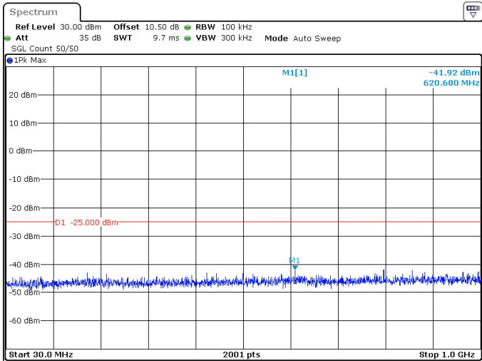
20MHz_30kHz_2592.99MHz_DFT-s-OFDM QPSK_RB1@50 -41.92 dBm
