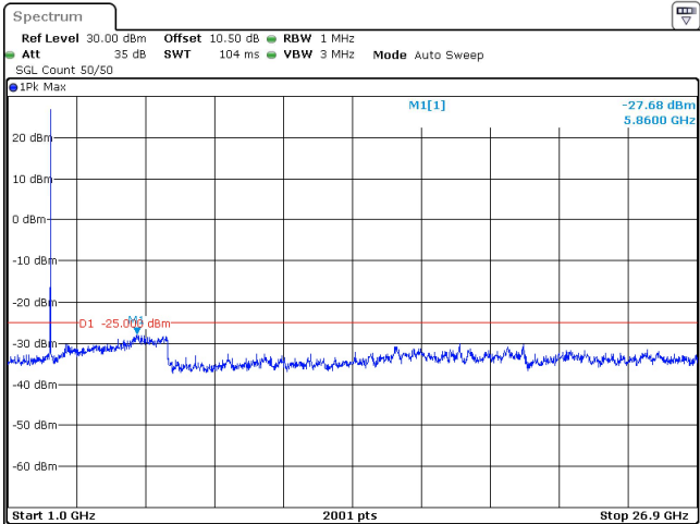
20MHz_30kHz_2592.99MHz_DFT-s-OFDM QPSK_RB1@50 -27.68 dBm
