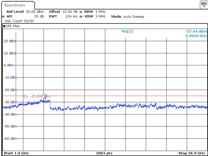
20MHz_30kHz_2679.99MHz_DFT-s-OFDM QPSK_RB1@0 -27.44 dBm
