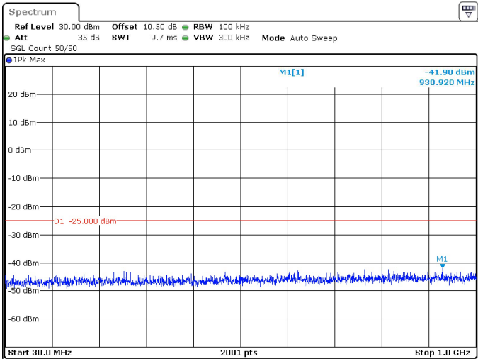
20MHz_30kHz_2592.99MHz_DFT-s-OFDM QPSK_RB1@0 -41.90 dBm
