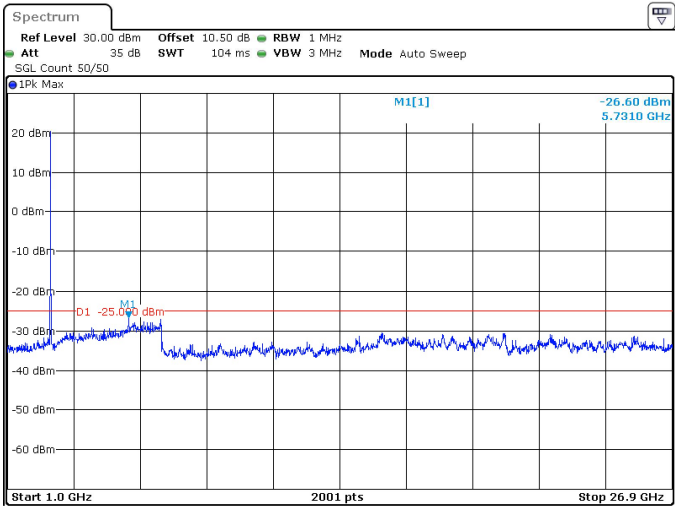
20MHz_30kHz_2679.99MHz_DFT-s-OFDM QPSK_RB50@0 -26.60 dBm
