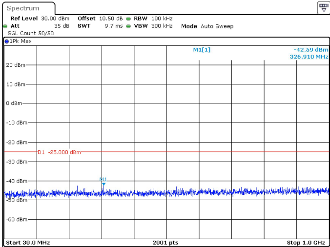
20MHz_30kHz_2679.99MHz_DFT-s-OFDM QPSK_RB1@50 -42.59 dBm
