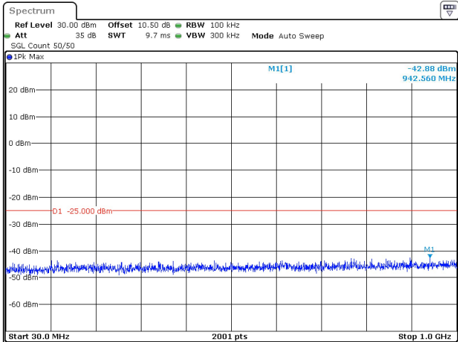
20MHz_30kHz_2679.99MHz_DFT-s-OFDM QPSK_RB50@0 -42.88 dBm
