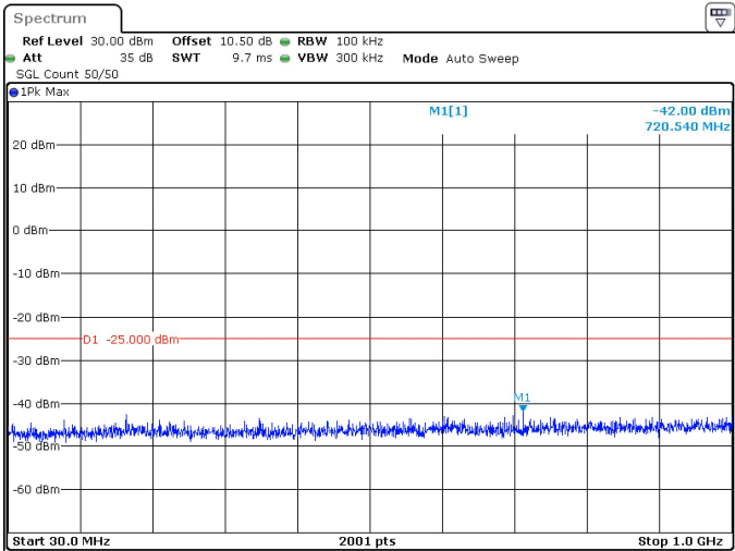
20MHz_30kHz_2679.99MHz_DFT-s-OFDM QPSK_RB1@0 -42.00 dBm
