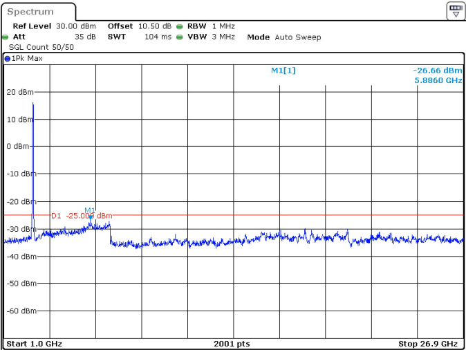
60MHz_30kHz_2659.98MHz_DFT-s-OFDM QPSK_RB162@0 -26.66 dBm
