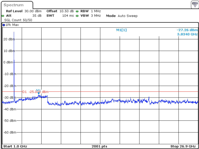
60MHz_30kHz_2592.99MHz_DFT-s-OFDM QPSK_RB1@0 -27.26 dBm
