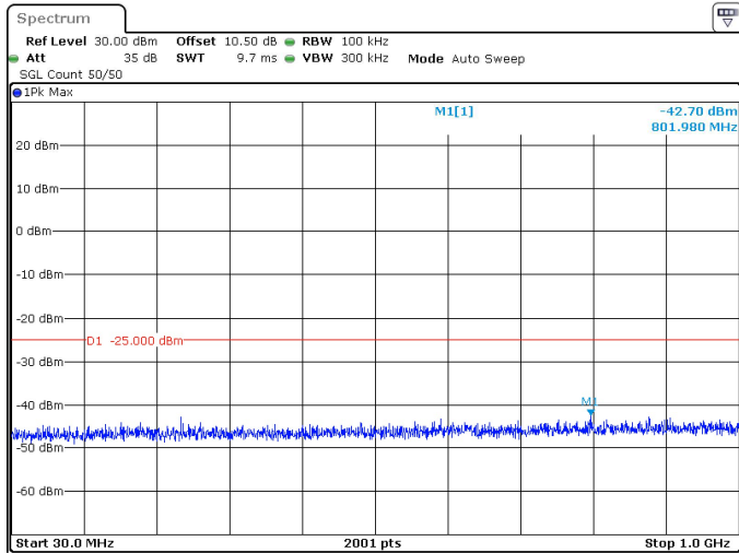
60MHz_30kHz_2659.98MHz_DFT-s-OFDM QPSK_RB1@0 -42.70 dBm
