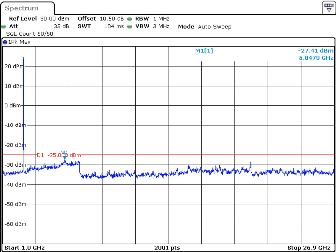
60MHz_30kHz_2659.98MHz_DFT-s-OFDM QPSK_RB1@0 -27.41 dBm
