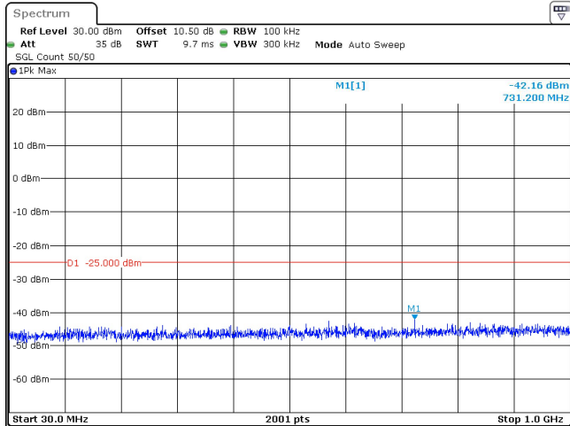
60MHz_30kHz_2659.98MHz_DFT-s-OFDM QPSK_RB162@0 -42.16 dBm
