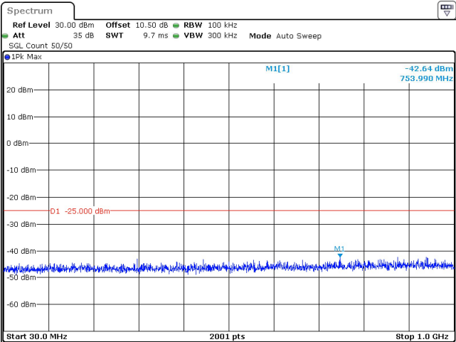
60MHz_30kHz_2659.98MHz_DFT-s-OFDM QPSK_RB1@161 -42.64 dBm
