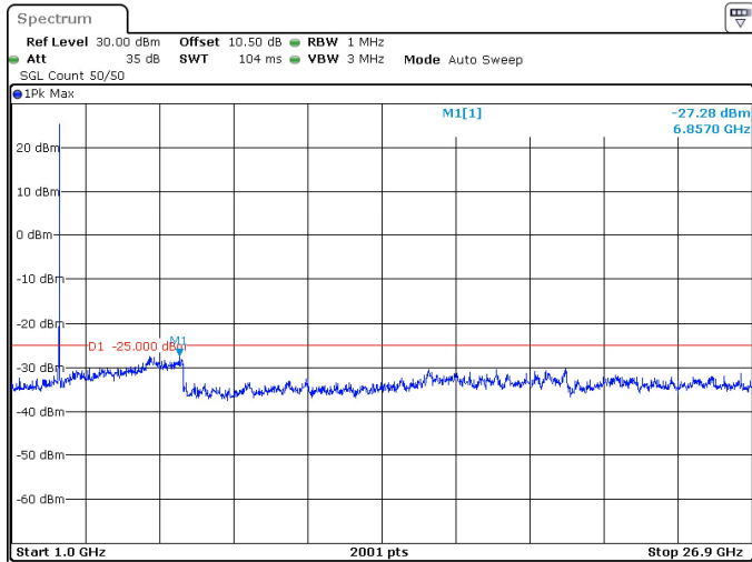
60MHz_30kHz_2659.98MHz_DFT-s-OFDM QPSK_RB1@161 -27.28 dBm
