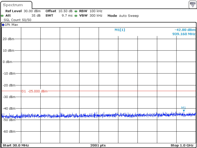
80MHz_30kHz_2649.99MHz_DFT-s-OFDM QPSK_RB1@0 -42.80 dBm
