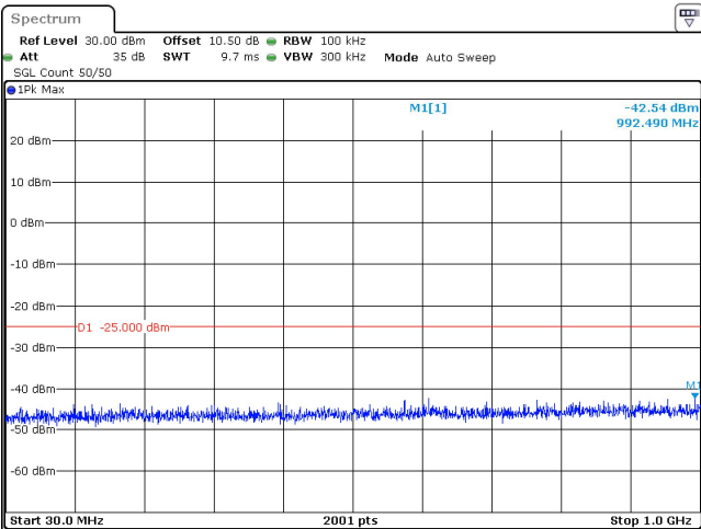
90MHz_30kHz_2541MHz_DFT-s-OFDM QPSK_RB1@244 -42.54 dBm
