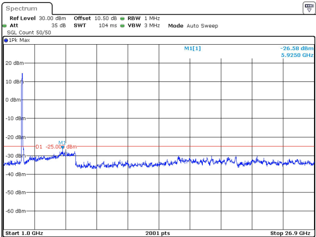
90MHz_30kHz_2541MHz_DFT-s-OFDM QPSK_RB243@0 -26.58 dBm
