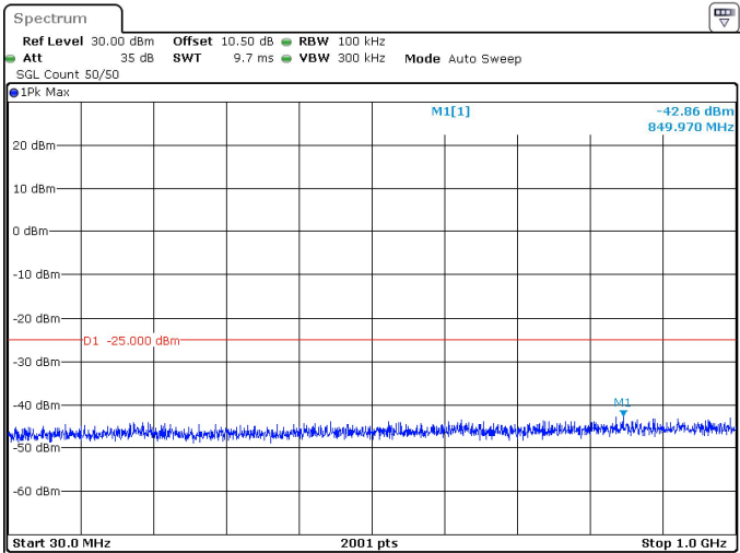
90MHz_30kHz_2541MHz_DFT-s-OFDM QPSK_RB1@0 -42.86 dBm
