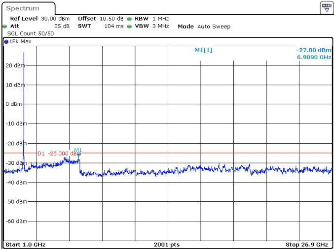
90MHz_30kHz_2541MHz_DFT-s-OFDM QPSK_RB1@244 -27.00 dBm
