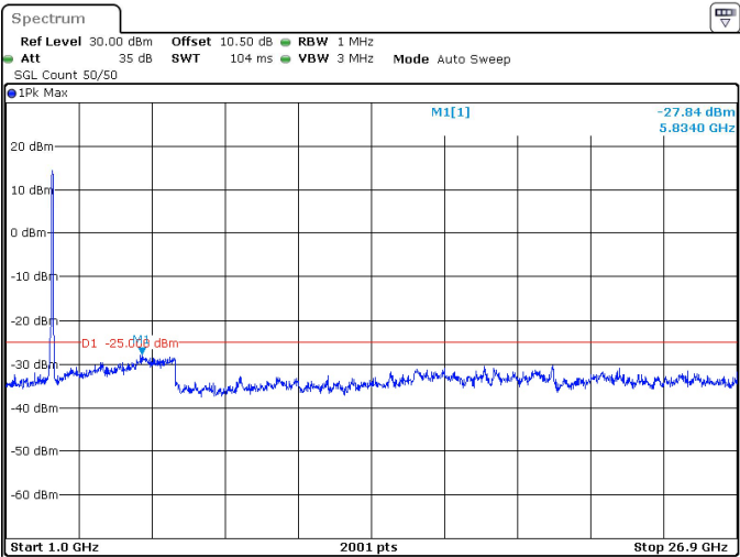
80MHz_30kHz_2649.99MHz_DFT-s-OFDM QPSK_RB216@0 -27.84 dBm
