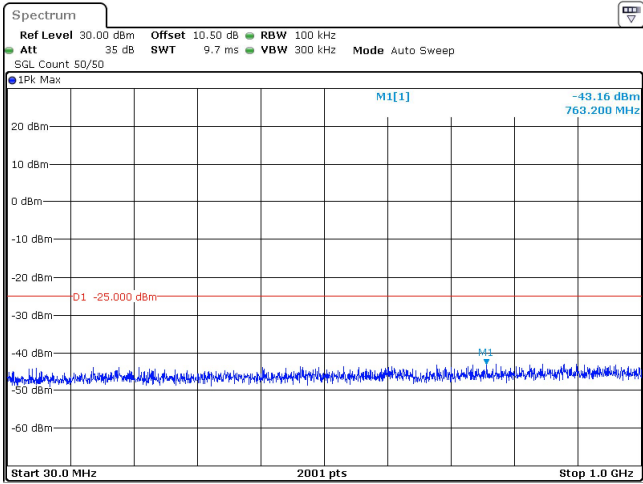
80MHz_30kHz_2649.99MHz_DFT-s-OFDM QPSK_RB216@0 -43.16 dBm
