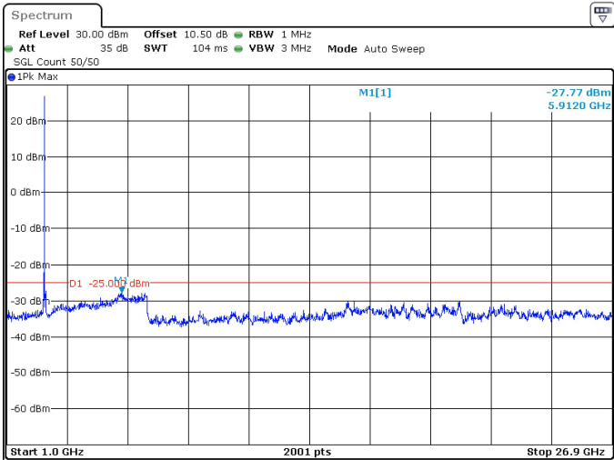
80MHz_30kHz_2649.99MHz_DFT-s-OFDM QPSK_RB1@0 -27.77 dBm
