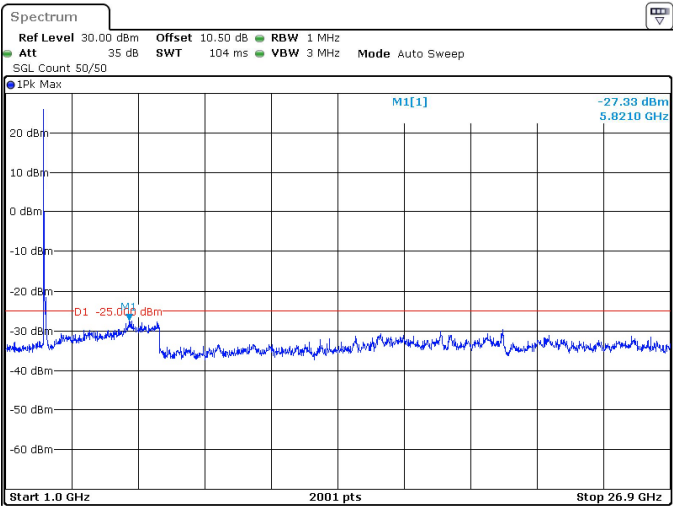
90MHz_30kHz_2541MHz_DFT-s-OFDM QPSK_RB1@0 -27.33 dBm
