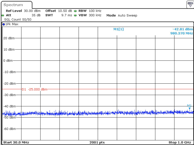
80MHz_30kHz_2649.99MHz_DFT-s-OFDM QPSK_RB1@216 -42.81 dBm
