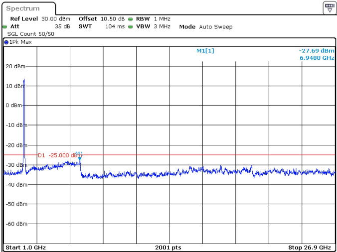
90MHz_30kHz_2592.99MHz_DFT-s-OFDM QPSK_RB243@0 -27.69 dBm
