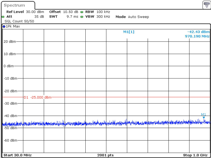
90MHz_30kHz_2541MHz_DFT-s-OFDM QPSK_RB243@0 -42.43 dBm
