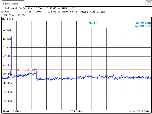
90MHz_30kHz_2644.98MHz_DFT-s-OFDM QPSK_RB243@0 -27.69 dBm
