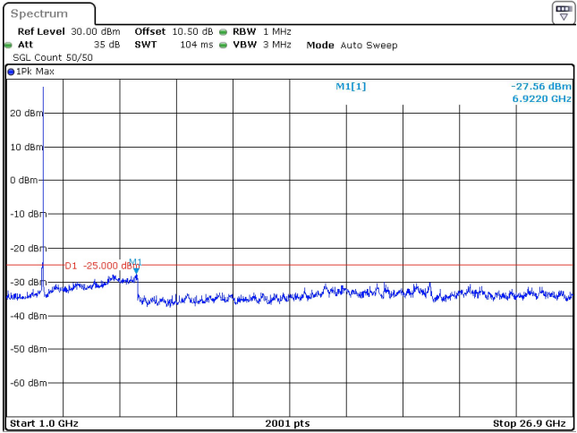
90MHz_30kHz_2644.98MHz_DFT-s-OFDM QPSK_RB1@244 -27.56 dBm
