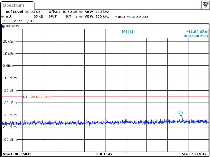
90MHz_30kHz_2644.98MHz_DFT-s-OFDM QPSK_RB243@0 -41.60 dBm
