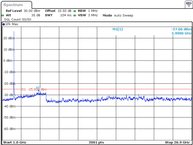
90MHz_30kHz_2644.98MHz_DFT-s-OFDM QPSK_RB1@0 -27.06 dBm
