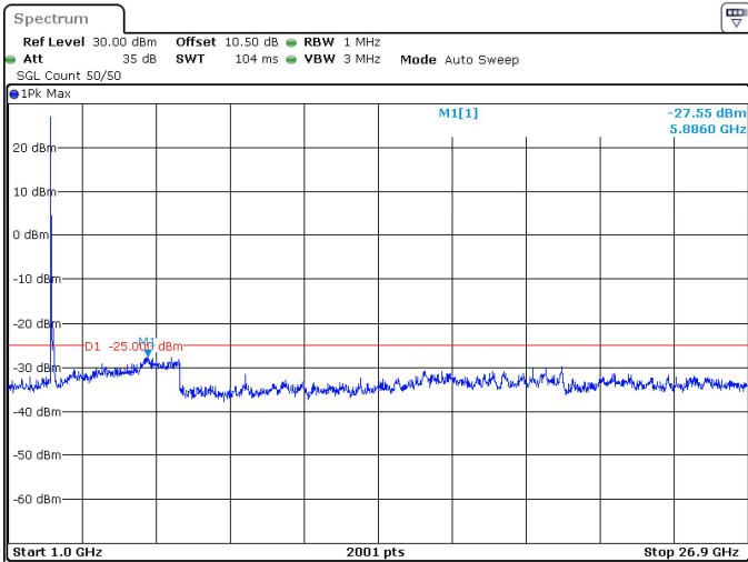
100MHz_30kHz_2546.01MHz_DFT-s-OFDM QPSK_RB1@0 -27.55 dBm
