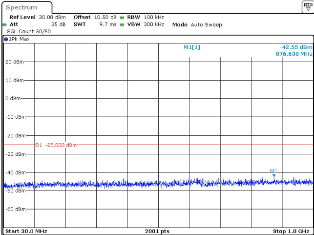
100MHz_30kHz_2546.01MHz_DFT-s-OFDM QPSK_RB270@0 -42.55 dBm
