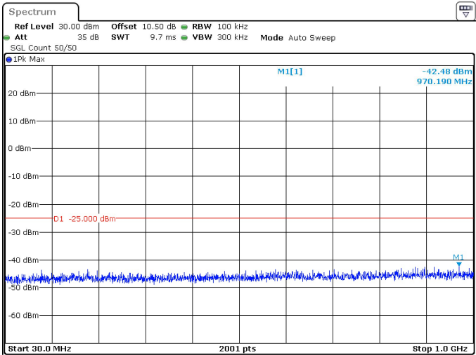
90MHz_30kHz_2644.98MHz_DFT-s-OFDM QPSK_RB1@0 -42.48 dBm
