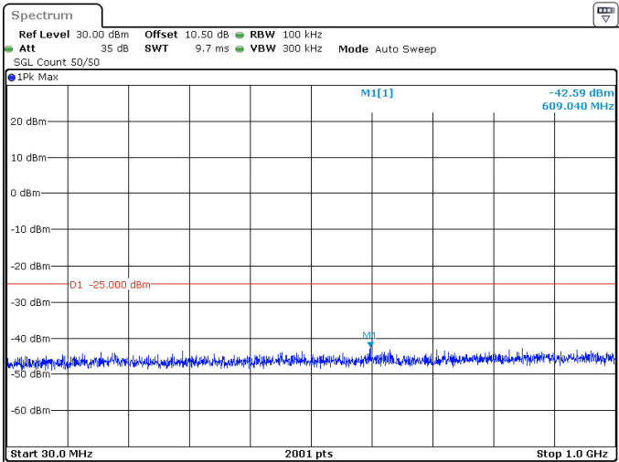
90MHz_30kHz_2644.98MHz_DFT-s-OFDM QPSK_RB1@244 -42.59 dBm
