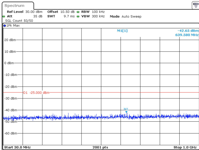
100MHz_30kHz_2640MHz_DFT-s-OFDM QPSK_RB1@272 -42.65 dBm
