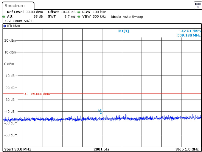
100MHz_30kHz_2640MHz_DFT-s-OFDM QPSK_RB1@0 -42.51 dBm
