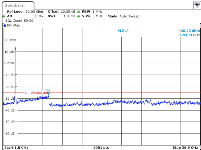
100MHz_30kHz_2592.99MHz_DFT-s-OFDM QPSK_RB270@0 -26.73 dBm
