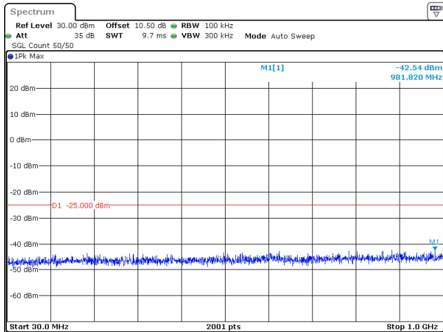
100MHz_30kHz_2640MHz_DFT-s-OFDM QPSK_RB270@0 -42.54 dBm
