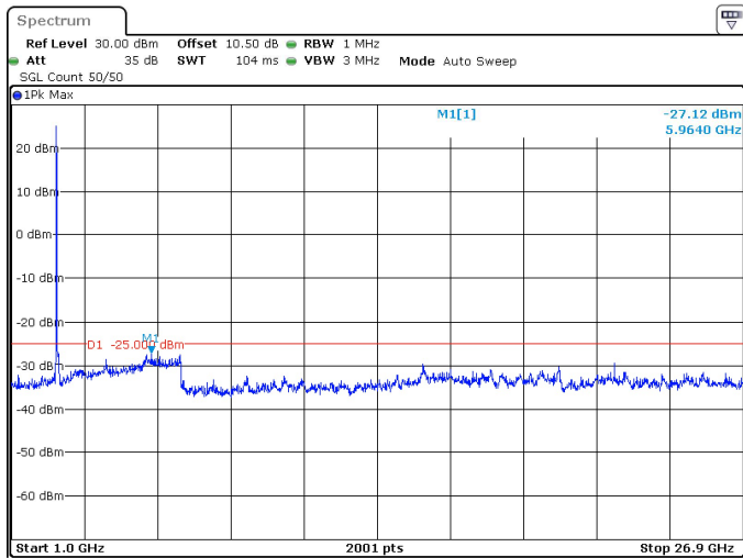
100MHz_30kHz_2640MHz_DFT-s-OFDM QPSK_RB1@0 -27.12 dBm
