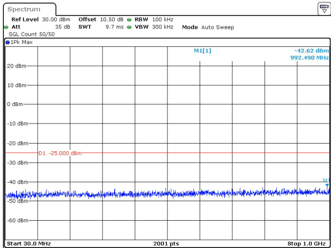
100MHz_30kHz_2592.99MHz_DFT-s-OFDM QPSK_RB270@0 -42.62 dBm
