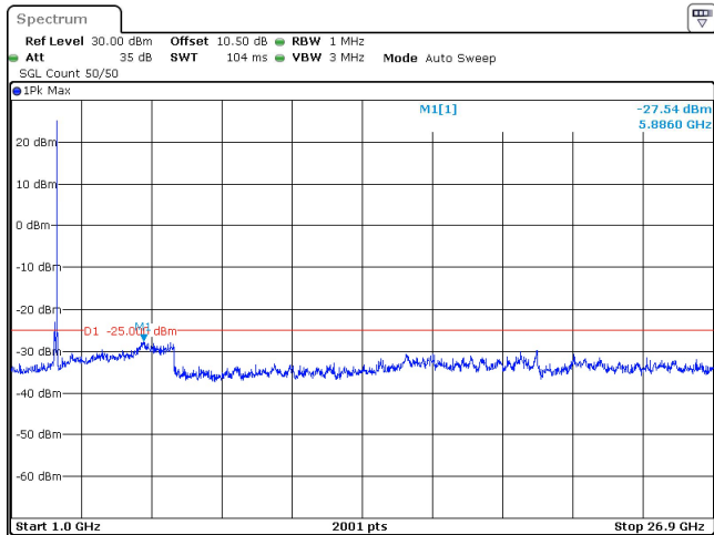
100MHz_30kHz_2640MHz_DFT-s-OFDM QPSK_RB1@272 -27.54 dBm
