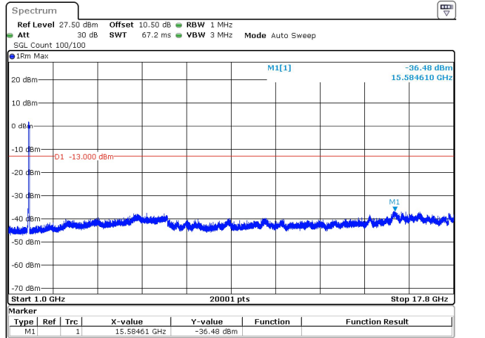
30MHz_15kHz_1765MHz_DFT-s-OFDM QPSK_RB160@0 -36.48 dBm
