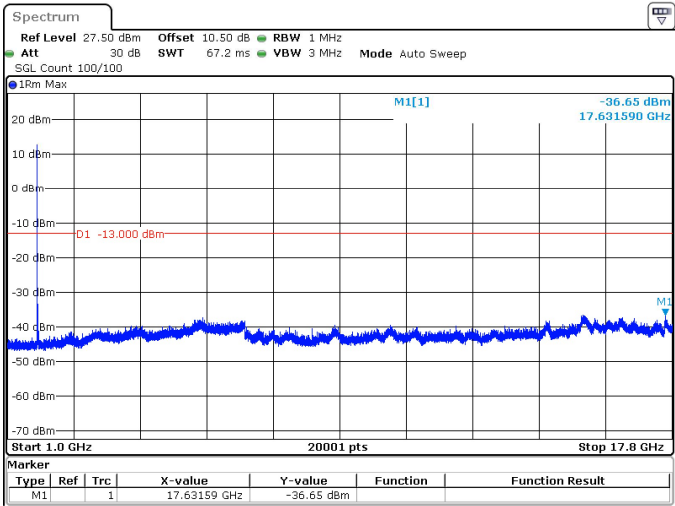
30MHz_15kHz_1765MHz_DFT-s-OFDM QPSK_RB1@0 -36.65 dBm
