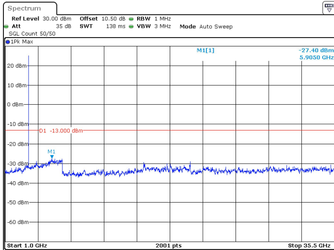
10MHz_30kHz_3455MHz_DFT-s-OFDM QPSK_RB1@23 -27.40 dBm
