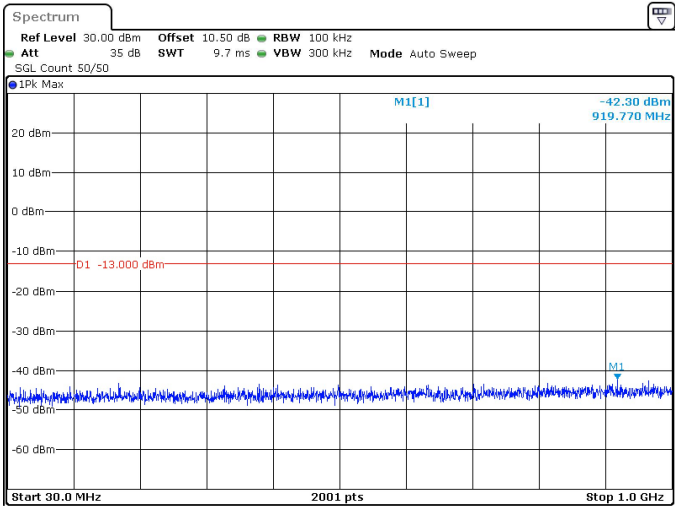
10MHz_15kHz_3455MHz_DFT-s-OFDM QPSK_RB50@0 -42.30 dBm
