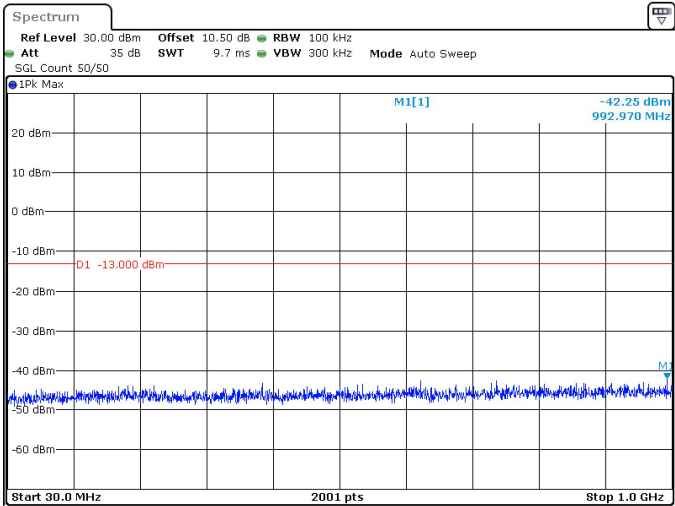
10MHz_15kHz_3455MHz_DFT-s-OFDM QPSK_RB50@0 -42.25 dBm
