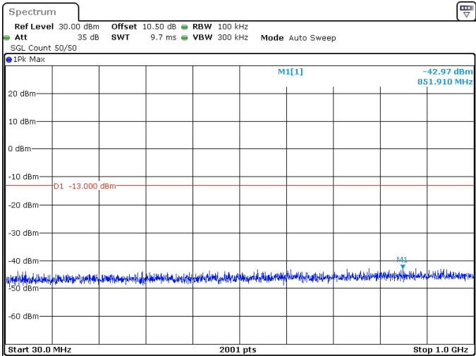
10MHz_15kHz_3500MHz_DFT-s-OFDM QPSK_RB50@0 -42.97 dBm
