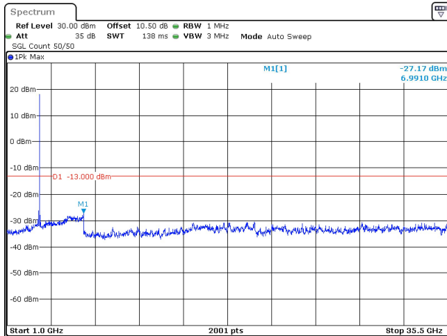
10MHz_15kHz_3545MHz_DFT-s-OFDM QPSK_RB50@0 -27.17 dBm
