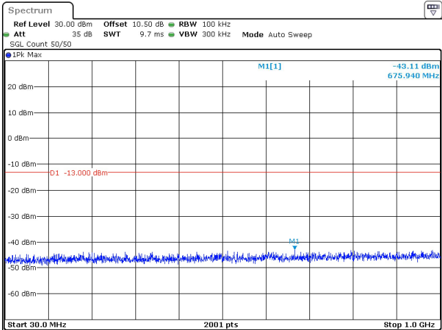
10MHz_30kHz_3455MHz_DFT-s-OFDM QPSK_RB1@23 -43.11 dBm
