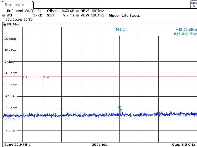
10MHz_30kHz_3455MHz_DFT-s-OFDM QPSK_RB24@0 -42.71 dBm
