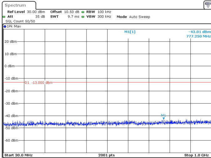
10MHz_30kHz_3455MHz_DFT-s-OFDM QPSK_RB1@0 -43.01 dBm
