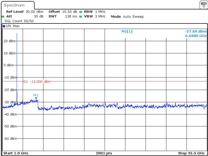
10MHz_30kHz_3455MHz_DFT-s-OFDM QPSK_RB1@0 -27.69 dBm
