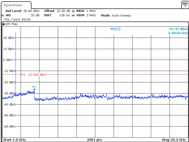
10MHz_30kHz_3500MHz_DFT-s-OFDM QPSK_RB1@23 -27.47 dBm
