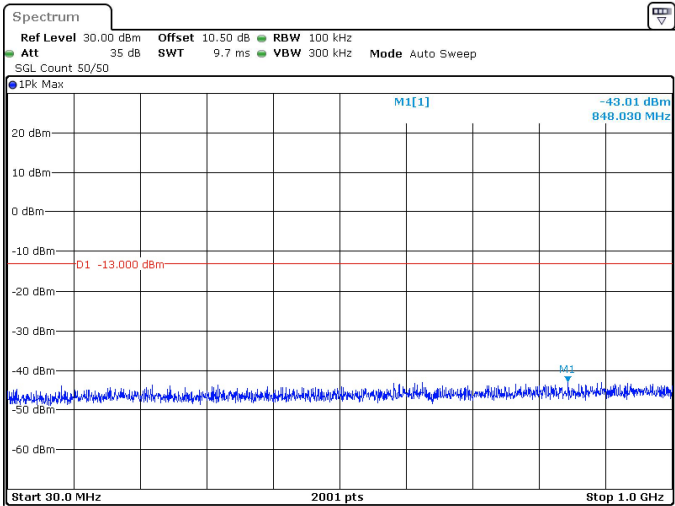
10MHz_30kHz_3500MHz_DFT-s-OFDM QPSK_RB1@0 -43.01 dBm
