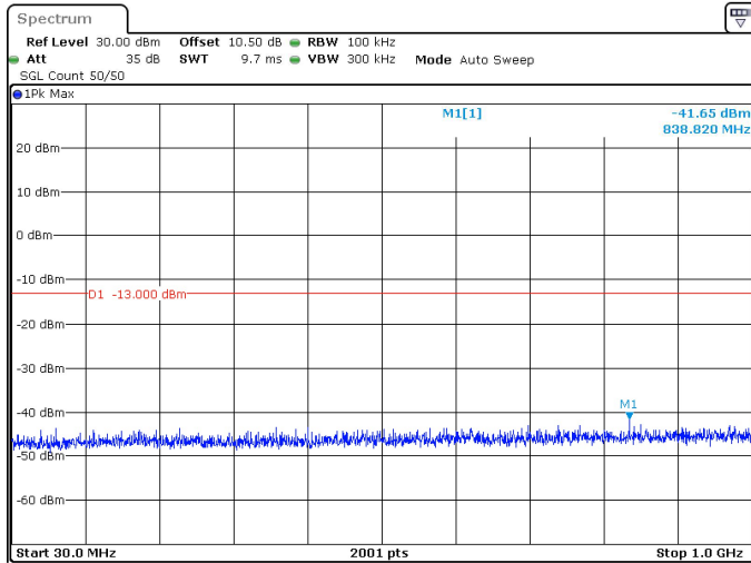
10MHz_30kHz_3500MHz_DFT-s-OFDM QPSK_RB1@23 -41.65 dBm
