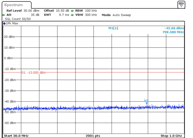
10MHz_30kHz_3545MHz_DFT-s-OFDM QPSK_RB24@0 -42.66 dBm
