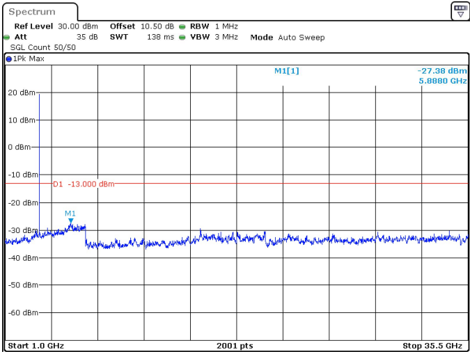
10MHz_30kHz_3545MHz_DFT-s-OFDM QPSK_RB24@0 -27.38 dBm
