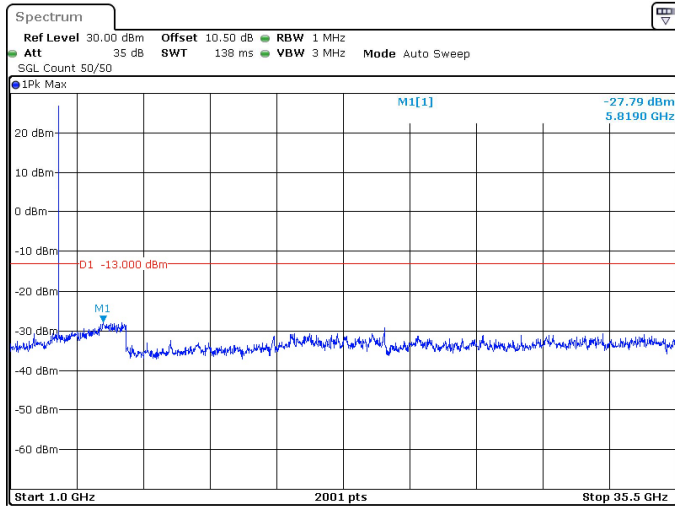
10MHz_30kHz_3500MHz_DFT-s-OFDM QPSK_RB1@0 -27.79 dBm
