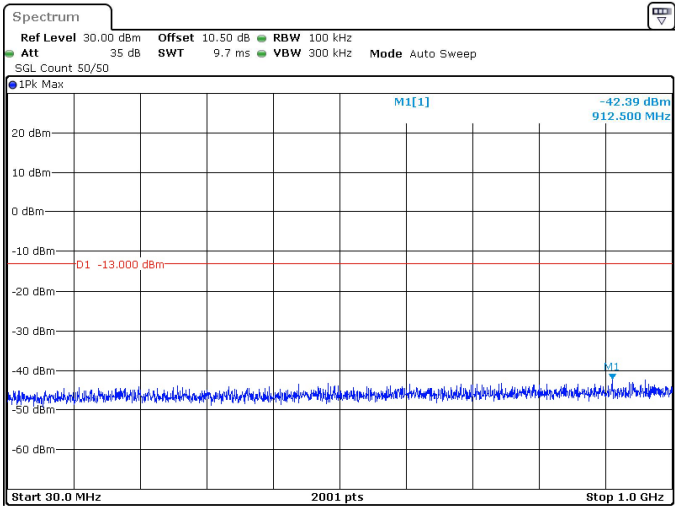
10MHz_30kHz_3500MHz_DFT-s-OFDM QPSK_RB24@0 -42.39 dBm
