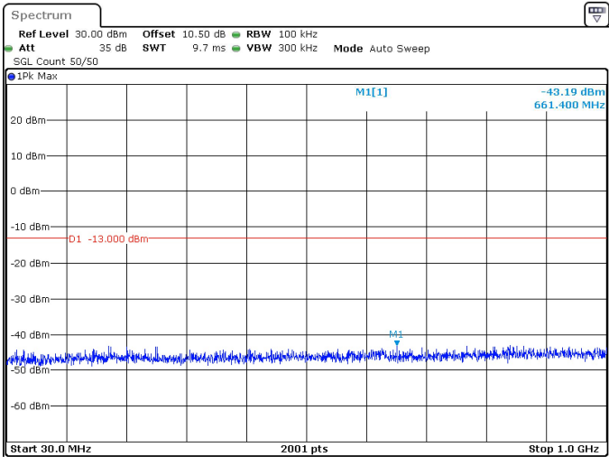
20MHz_15kHz_3460MHz_DFT-s-OFDM QPSK_RB1@0 -43.19 dBm
