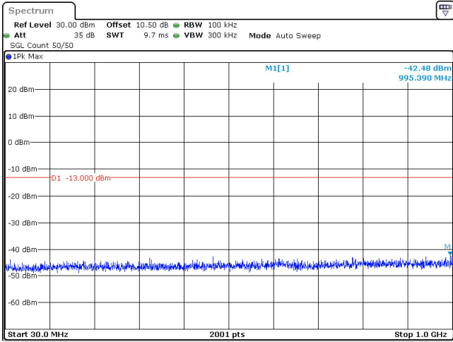
20MHz_15kHz_3460MHz_DFT-s-OFDM QPSK_RB1@105 -42.48 dBm
