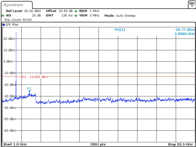
15MHz_30kHz_3500MHz_DFT-s-OFDM QPSK_RB1@0 -26.77 dBm
