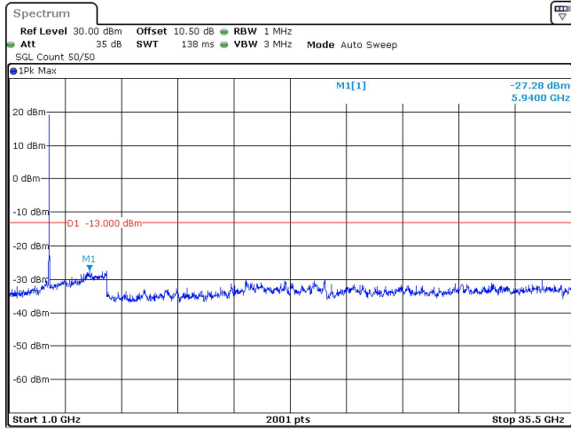
20MHz_15kHz_3460MHz_DFT-s-OFDM QPSK_RB100@0 -27.28 dBm
