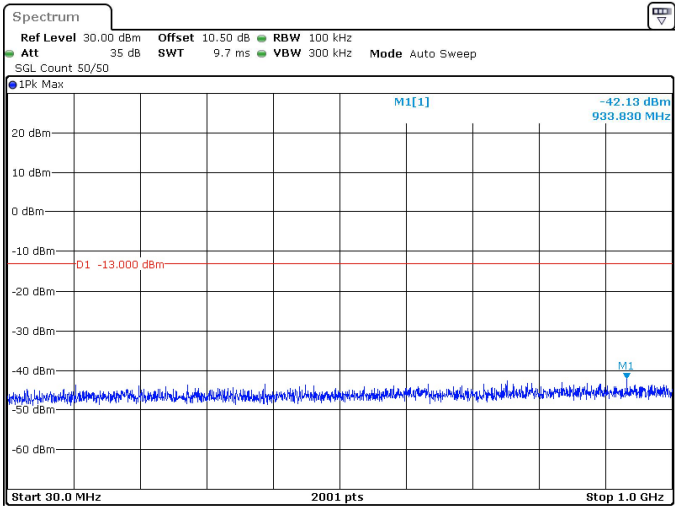
20MHz_15kHz_3460MHz_DFT-s-OFDM QPSK_RB100@0 -42.13 dBm
