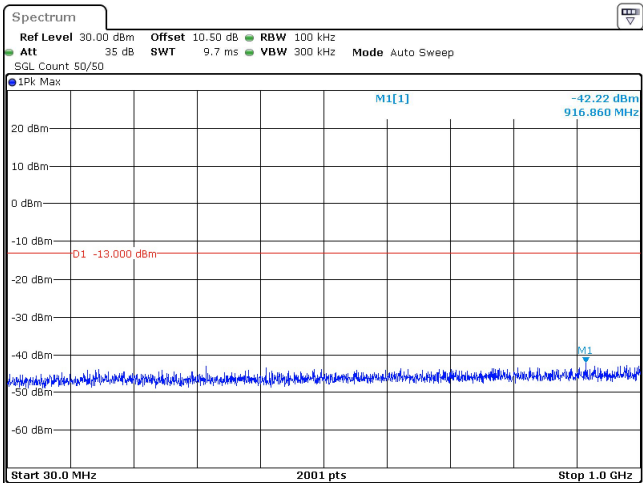
20MHz_30kHz_3460MHz_DFT-s-OFDM QPSK_RB1@50 -42.22 dBm
