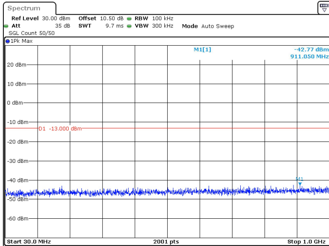
20MHz_15kHz_3500MHz_DFT-s-OFDM QPSK_RB1@105 -42.77 dBm
