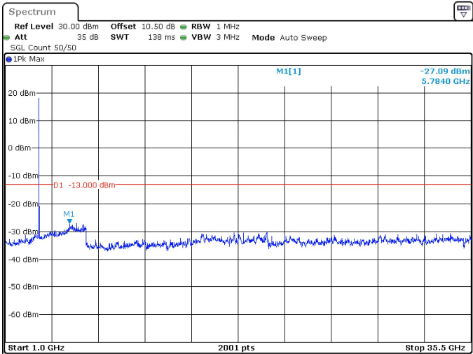
20MHz_15kHz_3500MHz_DFT-s-OFDM QPSK_RB100@0 -27.09 dBm
