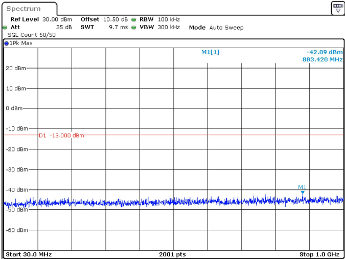
20MHz_15kHz_3500MHz_DFT-s-OFDM QPSK_RB1@0 -42.09 dBm
