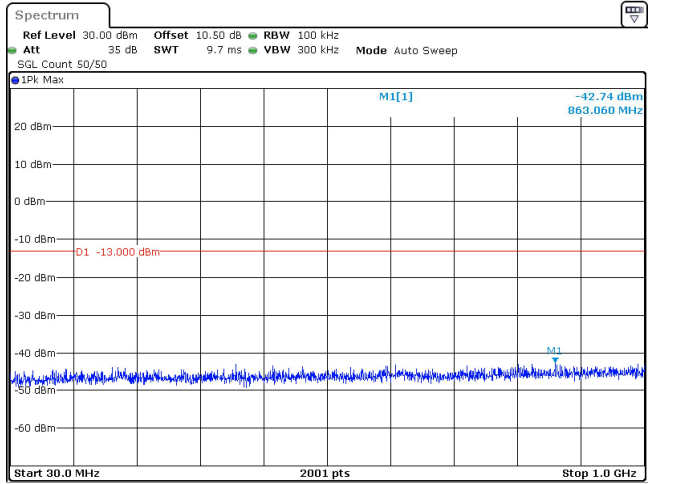
20MHz_15kHz_3500MHz_DFT-s-OFDM QPSK_RB100@0 -42.74 dBm
