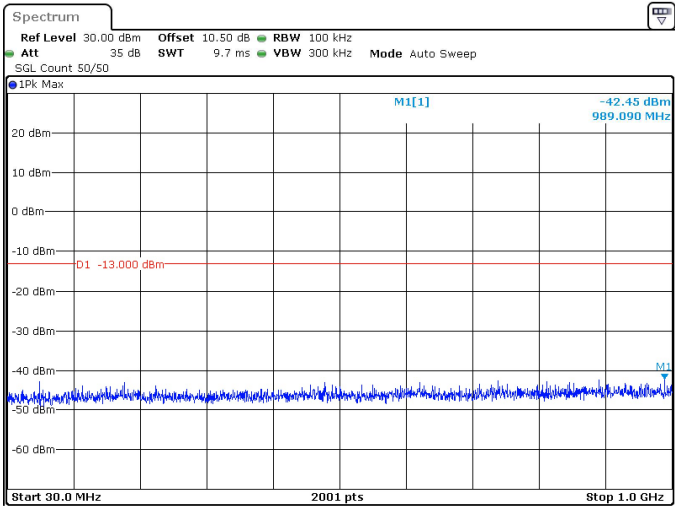
20MHz_15kHz_3540MHz_DFT-s-OFDM QPSK_RB1@0 -42.45 dBm
