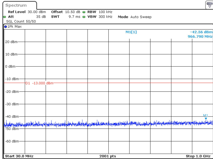
20MHz_30kHz_3460MHz_DFT-s-OFDM QPSK_RB1@0 -42.56 dBm
