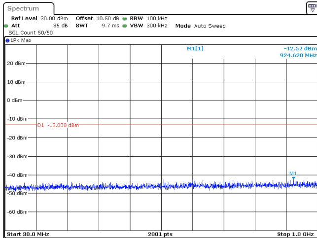
20MHz_30kHz_3500MHz_DFT-s-OFDM QPSK_RB50@0 -42.57 dBm
