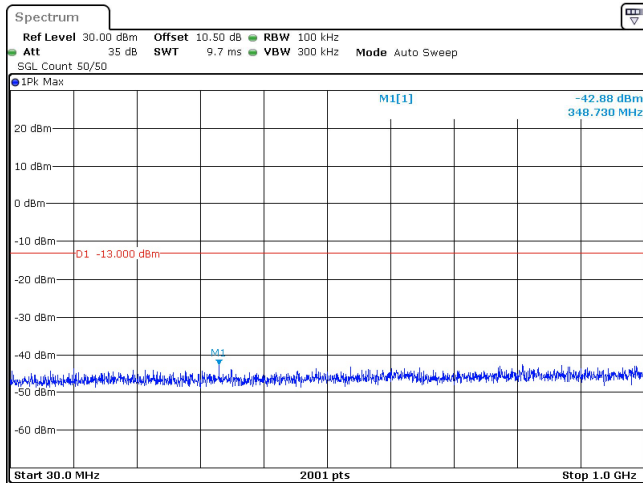
20MHz_30kHz_3540MHz_DFT-s-OFDM QPSK_RB50@0 -42.88 dBm
