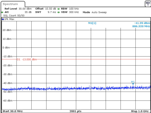
20MHz_30kHz_3540MHz_DFT-s-OFDM QPSK_RB1@50 -41.99 dBm
