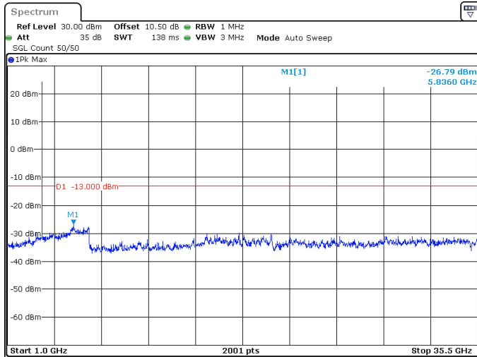
20MHz_30kHz_3540MHz_DFT-s-OFDM QPSK_RB1@0 -26.79 dBm
