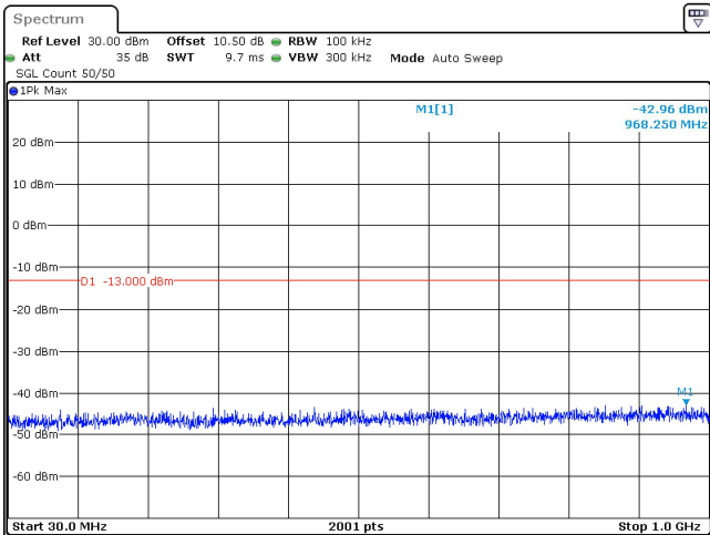
20MHz_30kHz_3500MHz_DFT-s-OFDM QPSK_RB1@50 -42.96 dBm
