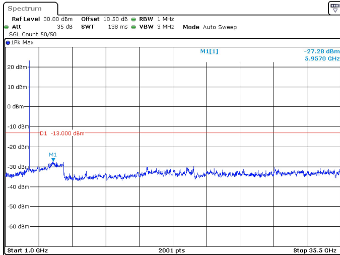
20MHz_30kHz_3500MHz_DFT-s-OFDM QPSK_RB1@50 -27.28 dBm
