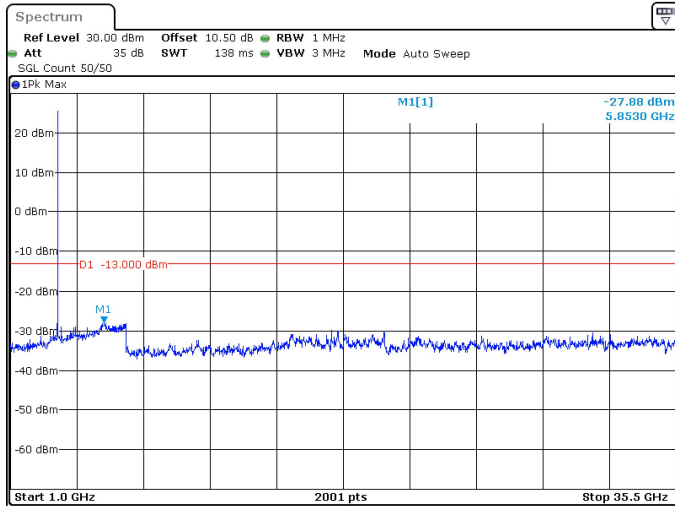
30MHz_15kHz_3465MHz_DFT-s-OFDM QPSK_RB1@0 -27.88 dBm
