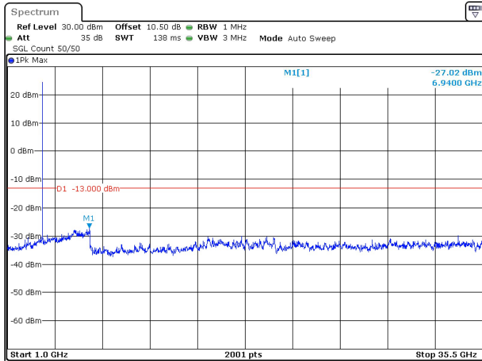
20MHz_30kHz_3540MHz_DFT-s-OFDM QPSK_RB1@50 -27.02 dBm
