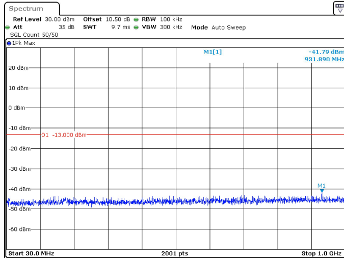
60MHz_30kHz_3480MHz_DFT-s-OFDM QPSK_RB1@161 -41.79 dBm
