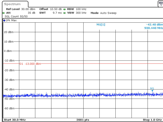
50MHz_30kHz_3500MHz_DFT-s-OFDM QPSK_RB1@0 -42.40 dBm
