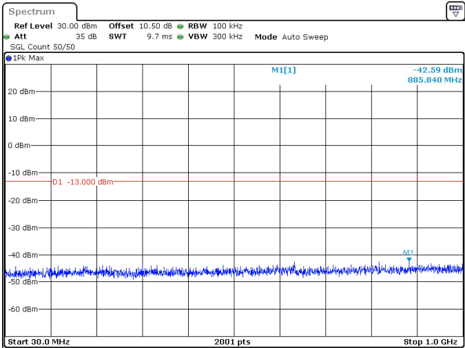
60MHz_30kHz_3480MHz_DFT-s-OFDM QPSK_RB1@0 -42.59 dBm
