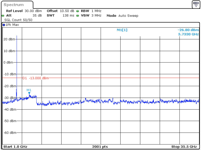
90MHz_30kHz_3500MHz_DFT-s-OFDM QPSK_RB1@244 -26.80 dBm
