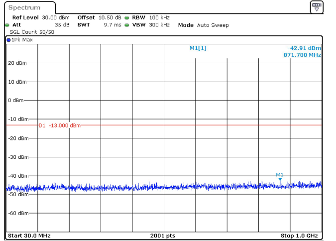
90MHz_30kHz_3500MHz_DFT-s-OFDM QPSK_RB243@0 -42.91 dBm
