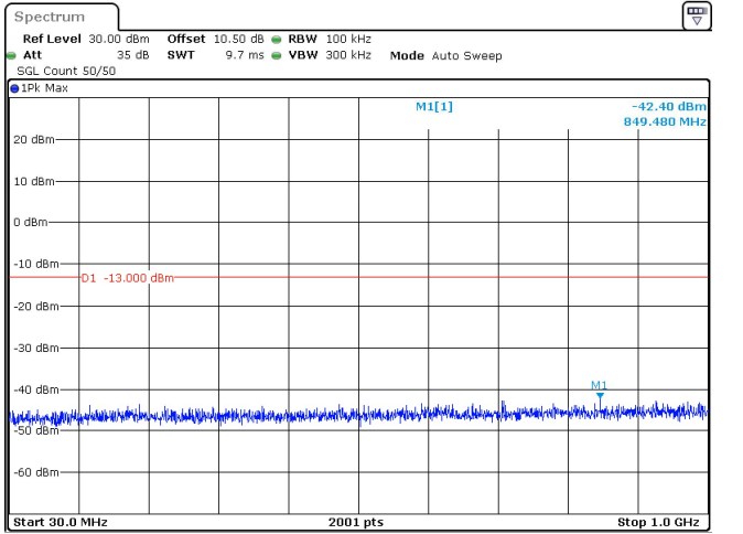
100MHz_30kHz_3500MHz_DFT-s-OFDM QPSK_RB270@0 -42.40 dBm
