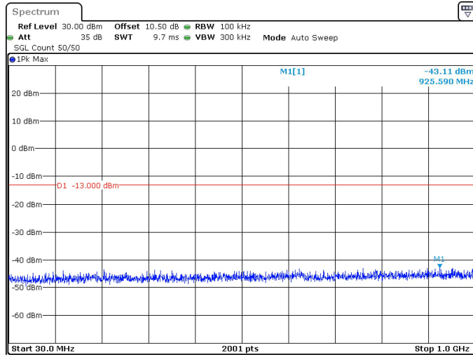
90MHz_30kHz_3500MHz_DFT-s-OFDM QPSK_RB1@0 -43.11 dBm
