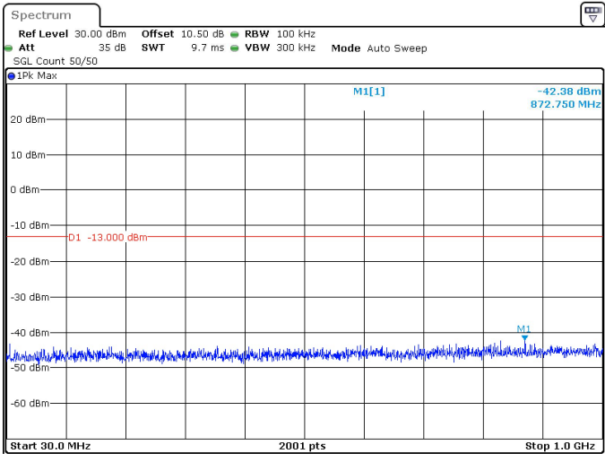
90MHz_30kHz_3505MHz_DFT-s-OFDM QPSK_RB243@0 -42.38 dBm
