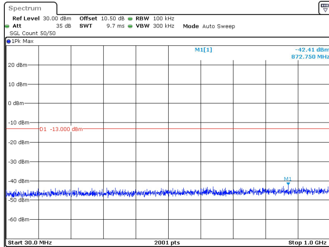
90MHz_30kHz_3505MHz_DFT-s-OFDM QPSK_RB1@0 -42.41 dBm
