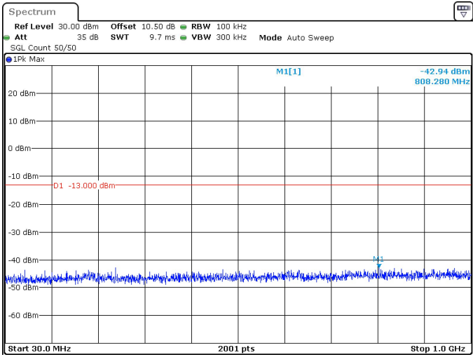
90MHz_30kHz_3495MHz_DFT-s-OFDM QPSK_RB243@0 -42.94 dBm
