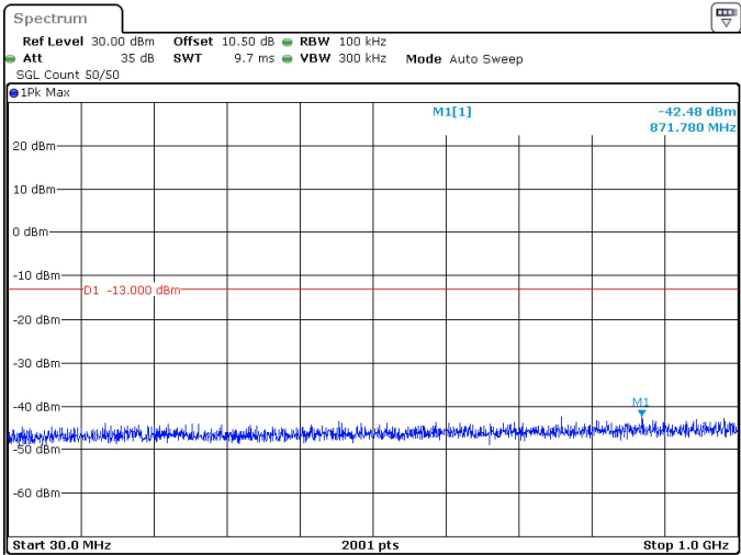
100MHz_30kHz_3500MHz_DFT-s-OFDM QPSK_RB1@0 -42.48 dBm
