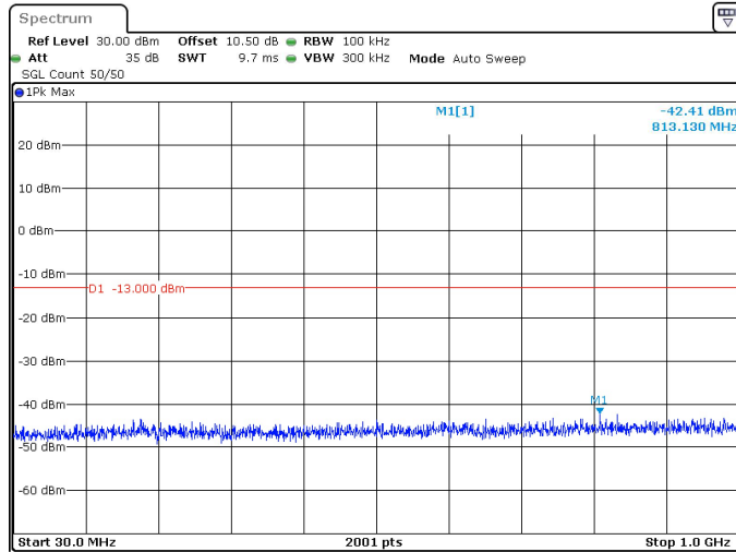
90MHz_30kHz_3500MHz_DFT-s-OFDM QPSK_RB1@244 -42.41 dBm
