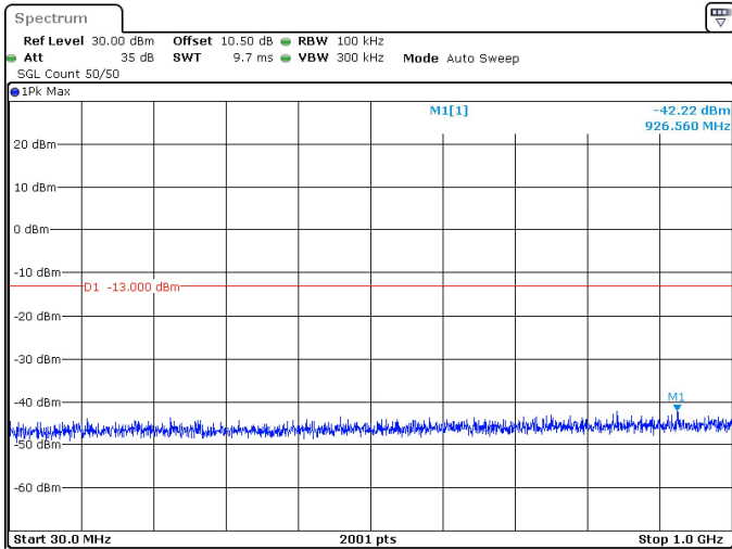
100MHz_30kHz_3500MHz_DFT-s-OFDM QPSK_RB1@272 -42.22 dBm
