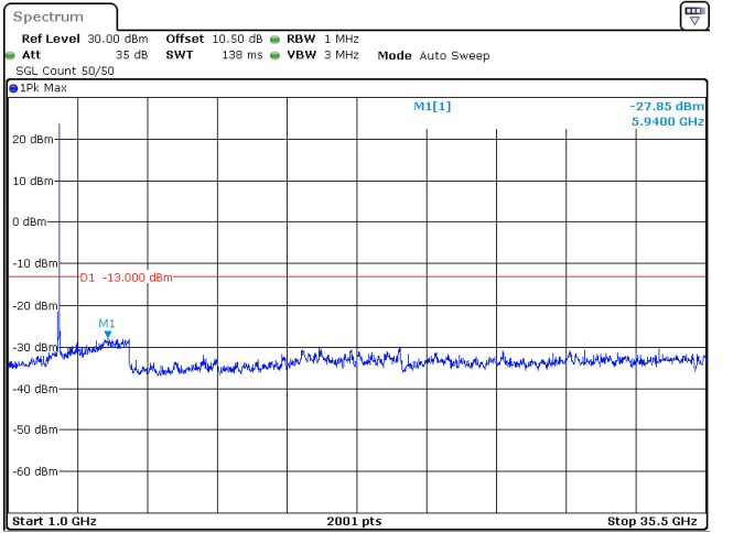
100MHz_30kHz_3500MHz_DFT-s-OFDM QPSK_RB1@272 -27.85 dBm
