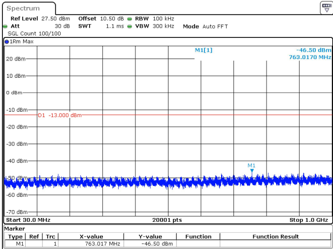
10MHz_30kHz_3840MHz_DFT-s-OFDM QPSK_RB1@0 -46.50 dBm
