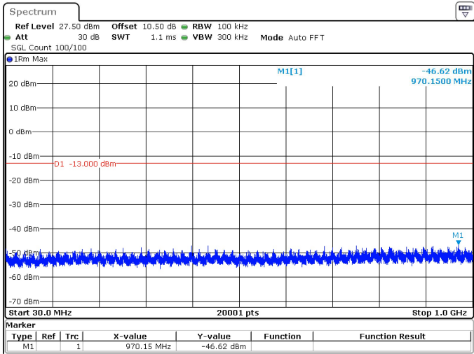
10MHz_30kHz_3705MHz_DFT-s-OFDM QPSK_RB1@23 -46.62 dBm
