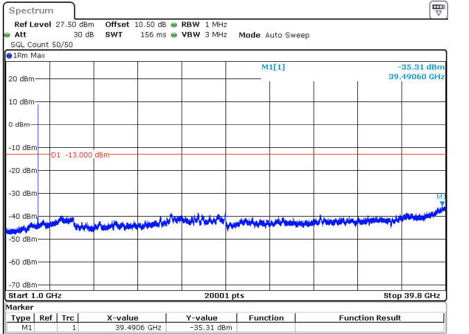
10MHz_30kHz_3840MHz_DFT-s-OFDM QPSK_RB24@0 -35.31 dBm
