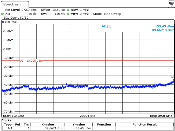
10MHz_30kHz_3705MHz_DFT-s-OFDM QPSK_RB1@0 -35.45 dBm
