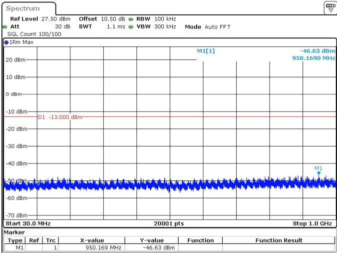
10MHz_30kHz_3975MHz_DFT-s-OFDM QPSK_RB1@23 -46.63 dBm
