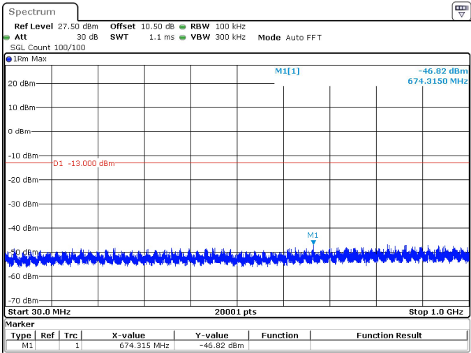
10MHz_30kHz_3840MHz_DFT-s-OFDM QPSK_RB24@0 -46.82 dBm
