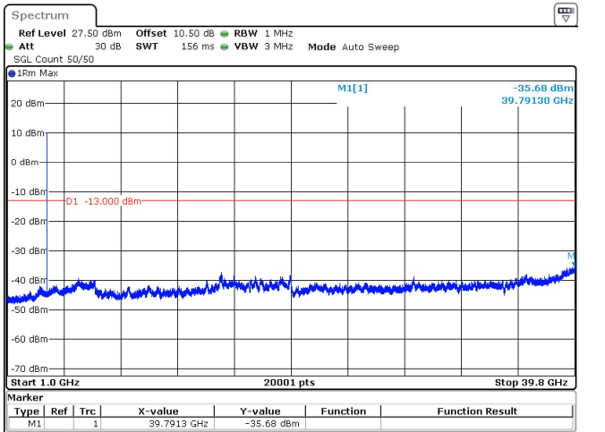
10MHz_30kHz_3705MHz_DFT-s-OFDM QPSK_RB24@0 -35.68 dBm
