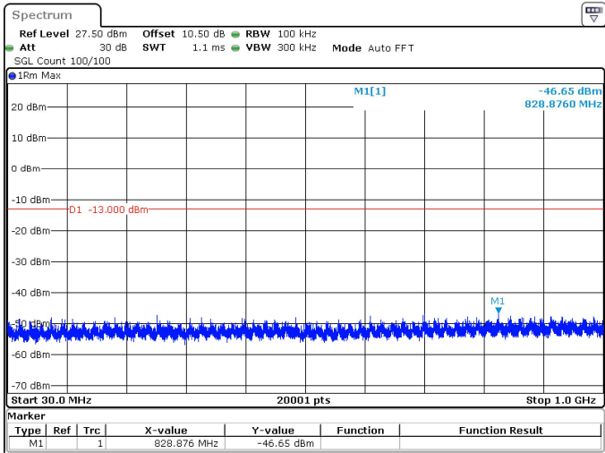
10MHz_30kHz_3705MHz_DFT-s-OFDM QPSK_RB1@0 -46.65 dBm
