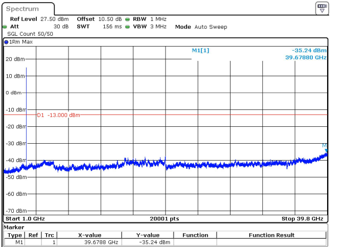
10MHz_30kHz_3705MHz_DFT-s-OFDM QPSK_RB1@23 -35.24 dBm
