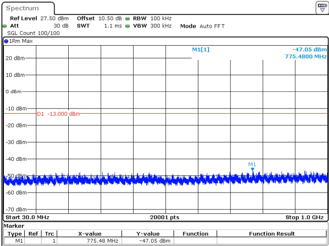
10MHz_30kHz_3705MHz_DFT-s-OFDM QPSK_RB24@0 -47.05 dBm
