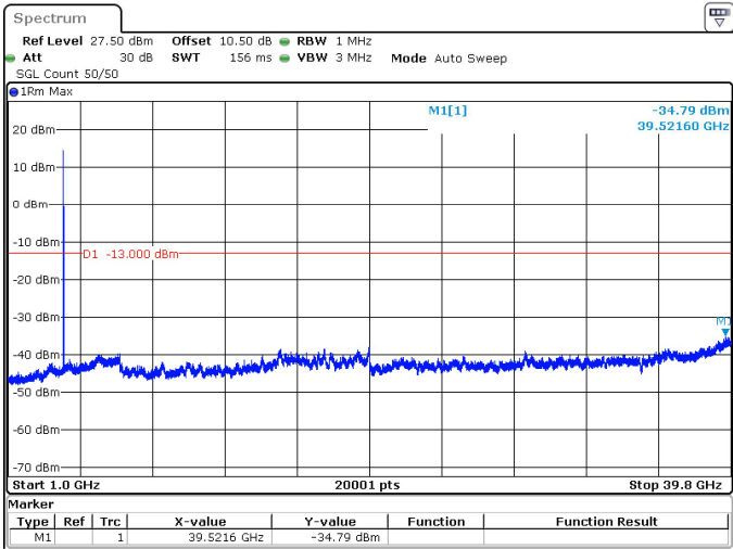
10MHz_30kHz_3975MHz_DFT-s-OFDM QPSK_RB1@0 -34.79 dBm
