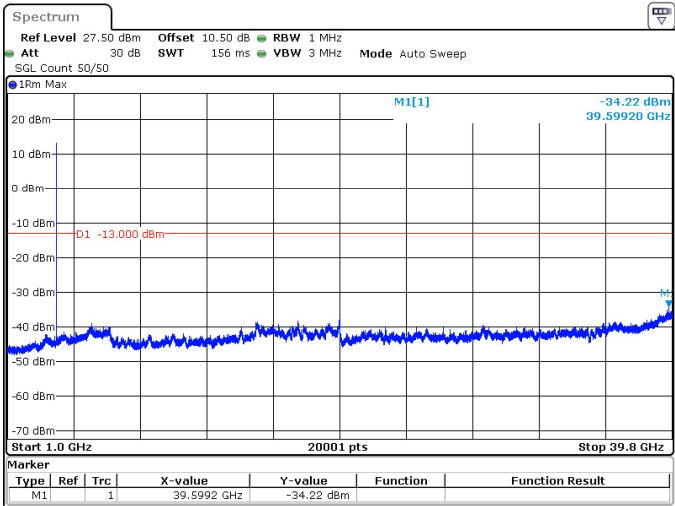
10MHz_30kHz_3840MHz_DFT-s-OFDM QPSK_RB1@0 -34.22 dBm
