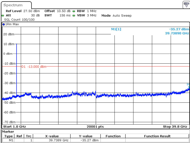
10MHz_30kHz_3975MHz_DFT-s-OFDM QPSK_RB24@0 -35.27 dBm
