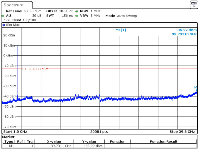
10MHz_15kHz_3975MHz_DFT-s-OFDM QPSK_RB50@0 -35.22 dBm
