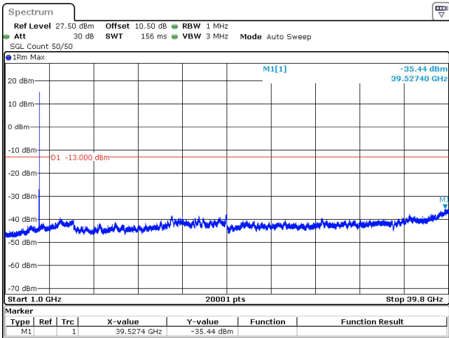
10MHz_30kHz_3975MHz_DFT-s-OFDM QPSK_RB1@23 -35.44 dBm
