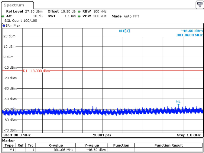
10MHz_30kHz_3975MHz_DFT-s-OFDM QPSK_RB1@0 -46.60 dBm
