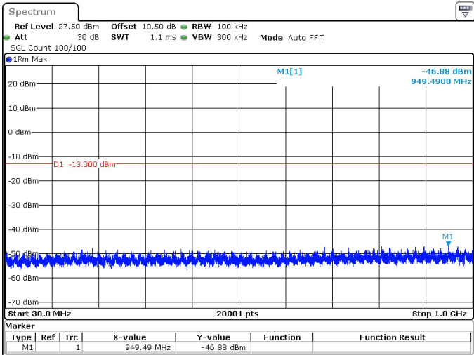
15MHz_30kHz_3707.5MHz_DFT-s-OFDM QPSK_RB1@0 -46.88 dBm
