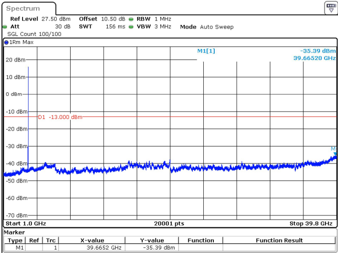
20MHz_15kHz_3840MHz_DFT-s-OFDM QPSK_RB1@0 -35.39 dBm
