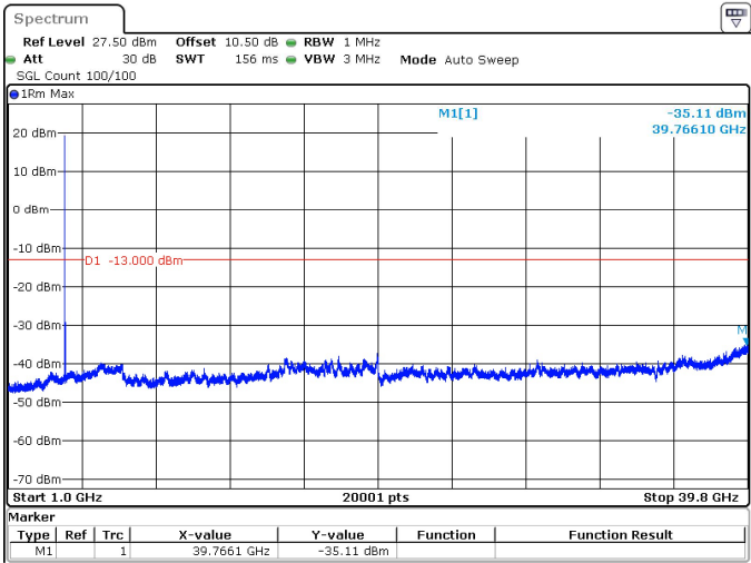
20MHz_15kHz_3970MHz_DFT-s-OFDM QPSK_RB1@0 -35.11 dBm
