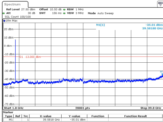
20MHz_15kHz_3970MHz_DFT-s-OFDM QPSK_RB100@0 -35.01 dBm
