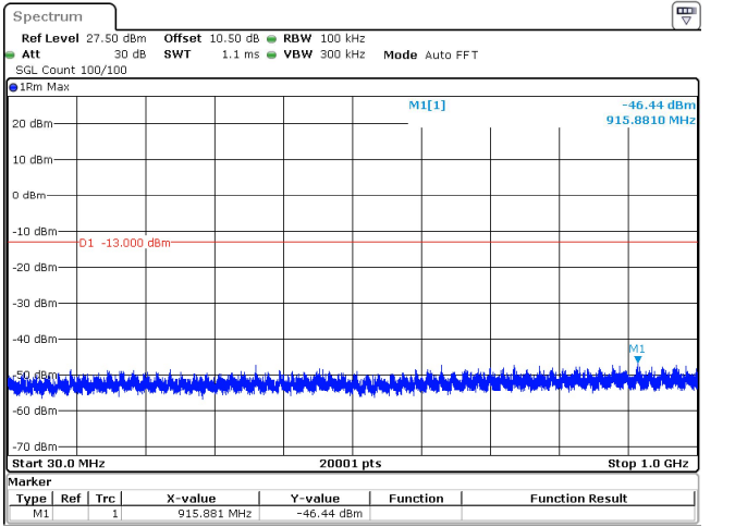
20MHz_15kHz_3710MHz_DFT-s-OFDM QPSK_RB1@105 -46.44 dBm
