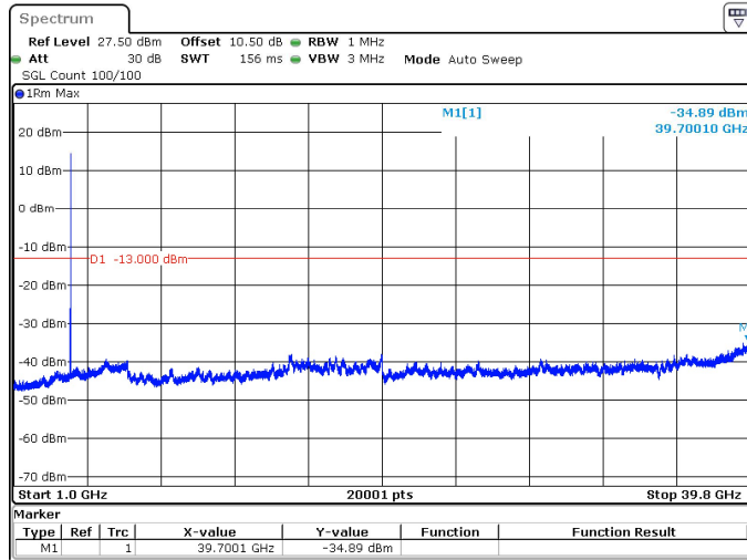
20MHz_15kHz_3970MHz_DFT-s-OFDM QPSK_RB1@105 -34.89 dBm
