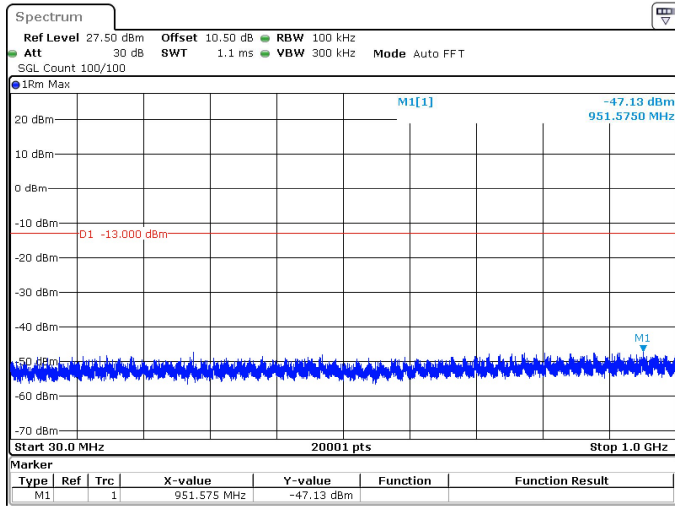
20MHz_15kHz_3710MHz_DFT-s-OFDM QPSK_RB1@0 -47.13 dBm
