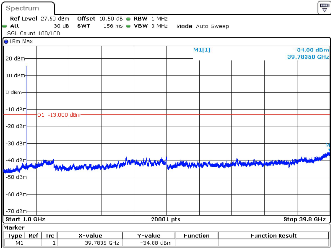
20MHz_15kHz_3710MHz_DFT-s-OFDM QPSK_RB1@0 -34.88 dBm
