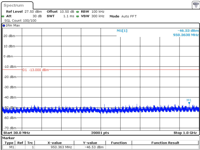
20MHz_15kHz_3970MHz_DFT-s-OFDM QPSK_RB1@105 -46.53 dBm
