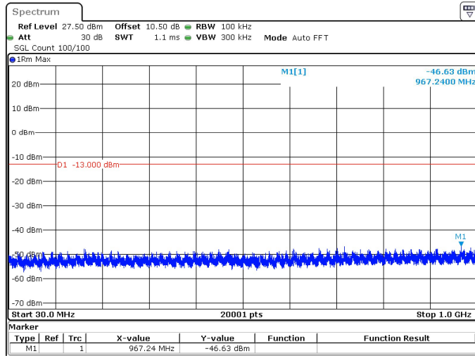
20MHz_15kHz_3970MHz_DFT-s-OFDM QPSK_RB1@0 -46.63 dBm
