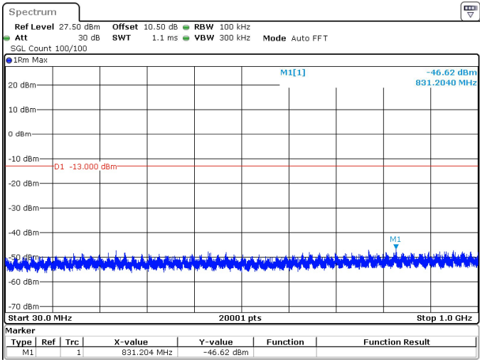
20MHz_15kHz_3710MHz_DFT-s-OFDM QPSK_RB100@0 -46.62 dBm
