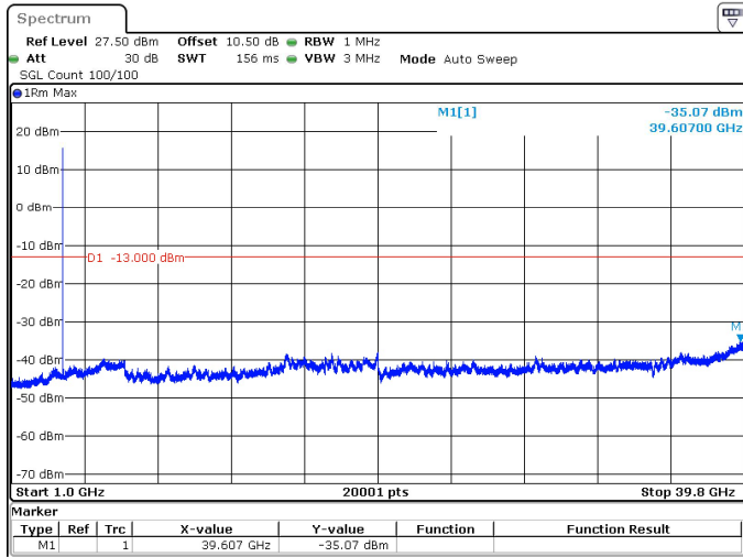
20MHz_15kHz_3710MHz_DFT-s-OFDM QPSK_RB1@105 -35.07 dBm
