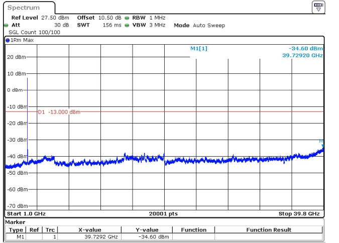
20MHz_15kHz_3710MHz_DFT-s-OFDM QPSK_RB100@0 -34.60 dBm
