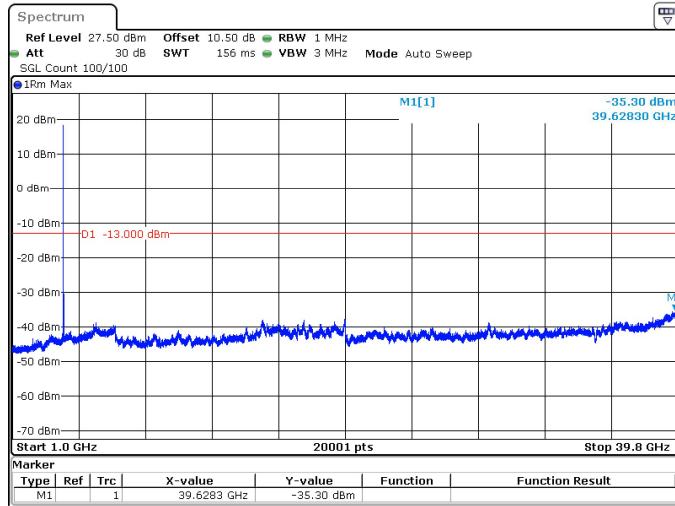
30MHz_15kHz_3965MHz_DFT-s-OFDM QPSK_RB1@0 -35.30 dBm
