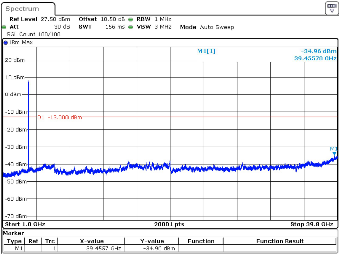
20MHz_30kHz_3970MHz_DFT-s-OFDM QPSK_RB50@0 -34.96 dBm
