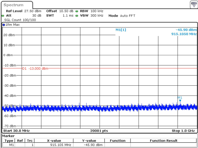
30MHz_15kHz_3965MHz_DFT-s-OFDM QPSK_RB1@0 -45.90 dBm
