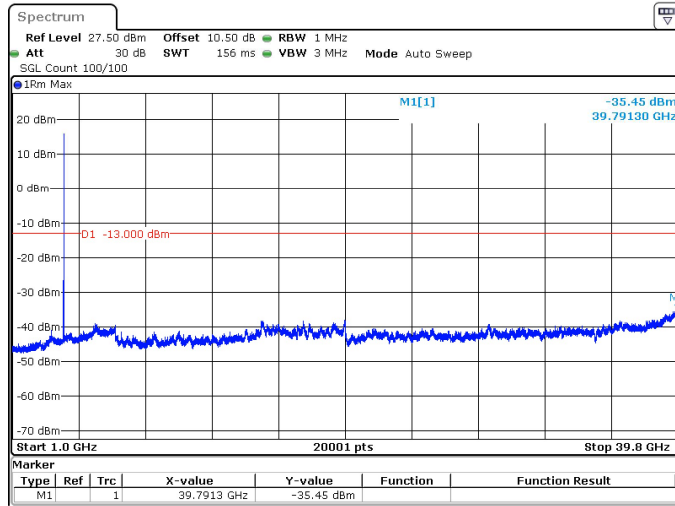
30MHz_15kHz_3965MHz_DFT-s-OFDM QPSK_RB1@159 -35.45 dBm
