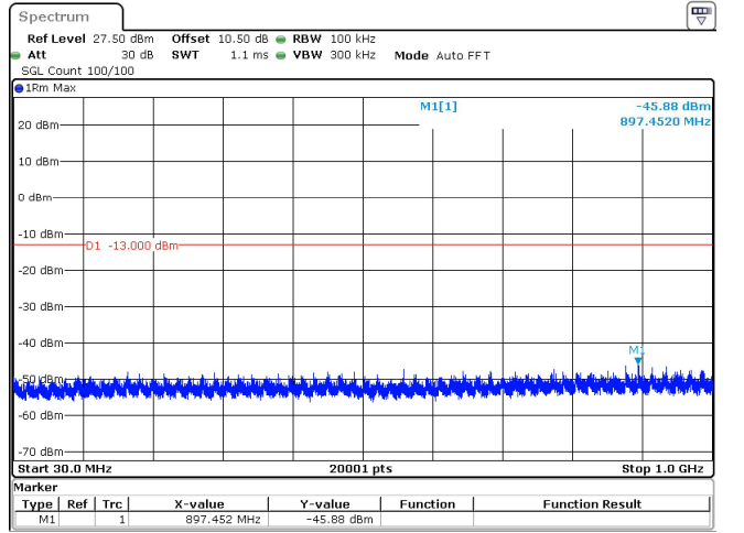
30MHz_15kHz_3965MHz_DFT-s-OFDM QPSK_RB160@0 -45.88 dBm
