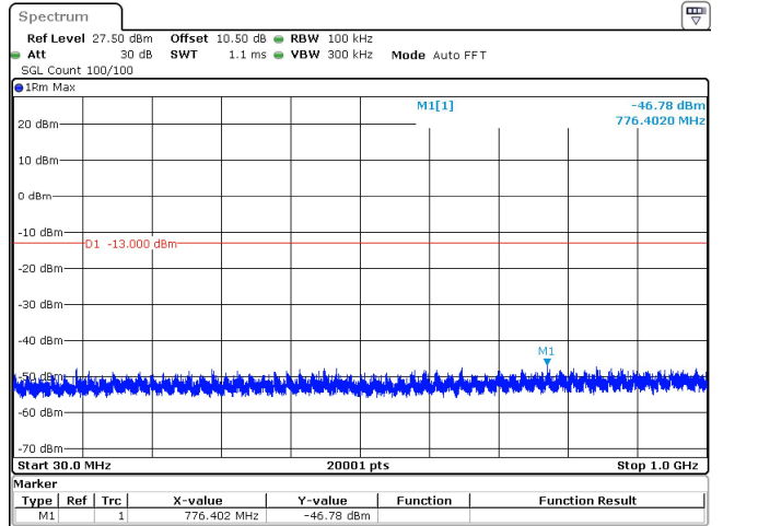
40MHz_15kHz_3960MHz_DFT-s-OFDM QPSK_RB216@0 -46.78 dBm
