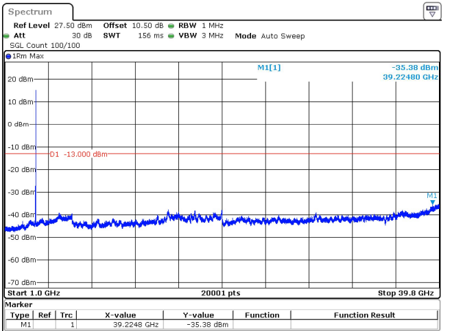
40MHz_15kHz_3720MHz_DFT-s-OFDM QPSK_RB1@215 -35.38 dBm
