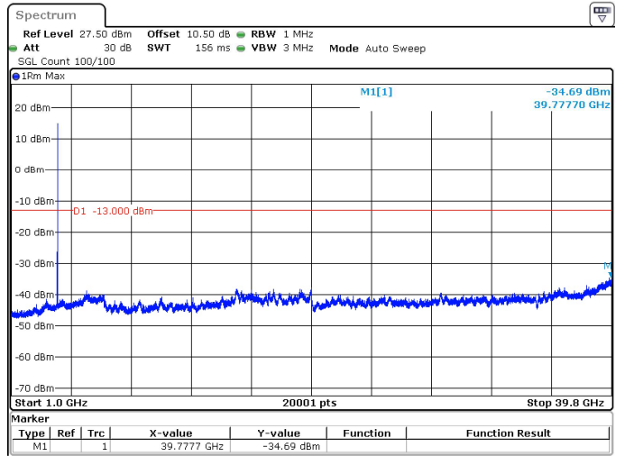
40MHz_15kHz_3960MHz_DFT-s-OFDM QPSK_RB1@215 -34.69 dBm
