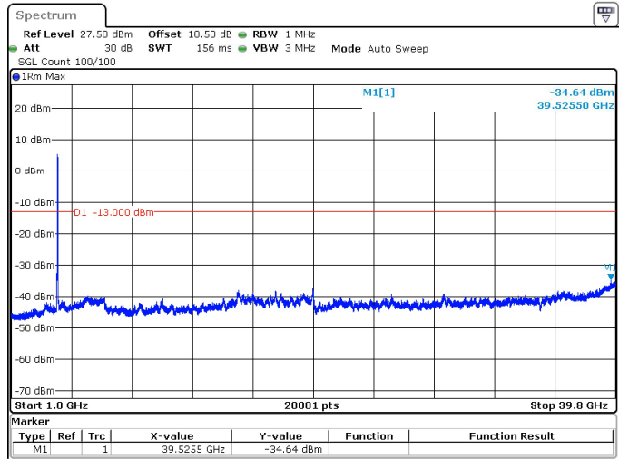
40MHz_15kHz_3960MHz_DFT-s-OFDM QPSK_RB1@0 -34.64 dBm
