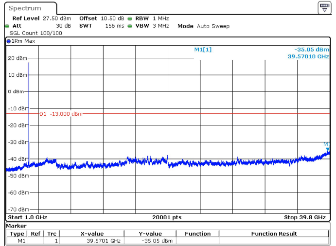
40MHz_15kHz_3720MHz_DFT-s-OFDM QPSK_RB1@0 -35.05 dBm
