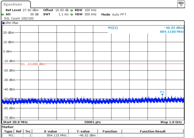
40MHz_15kHz_3960MHz_DFT-s-OFDM QPSK_RB1@215 -46.52 dBm
