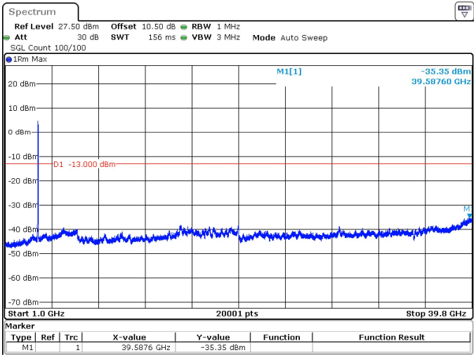
40MHz_15kHz_3720MHz_DFT-s-OFDM QPSK_RB216@0 -35.35 dBm
