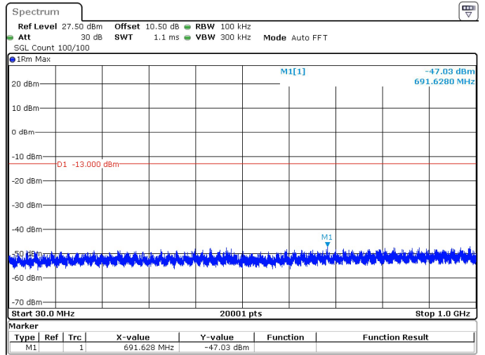
40MHz_15kHz_3720MHz_DFT-s-OFDM QPSK_RB1@215 -47.03 dBm
