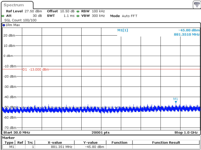
40MHz_15kHz_3960MHz_DFT-s-OFDM QPSK_RB1@0 -45.80 dBm
