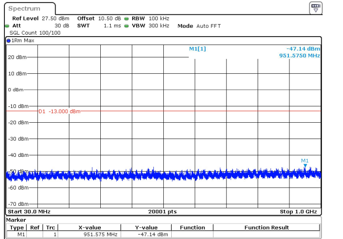
40MHz_15kHz_3720MHz_DFT-s-OFDM QPSK_RB216@0 -47.14 dBm
