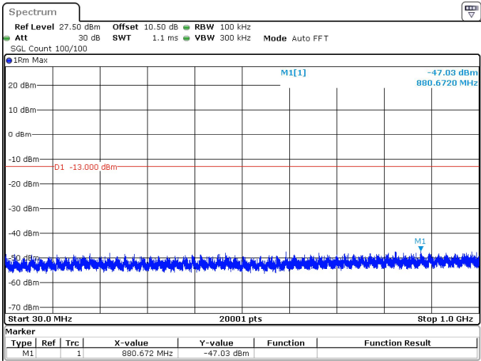
40MHz_15kHz_3720MHz_DFT-s-OFDM QPSK_RB1@0 -47.03 dBm
