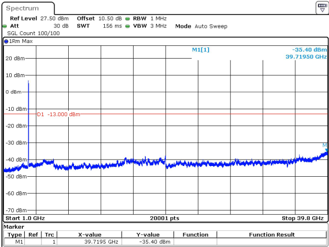
30MHz_15kHz_3965MHz_DFT-s-OFDM QPSK_RB160@0 -35.40 dBm
