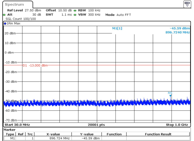
50MHz_15kHz_3955MHz_DFT-s-OFDM QPSK_RB270@0 -45.59 dBm
