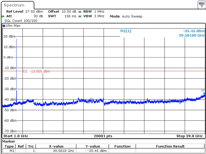
50MHz_15kHz_3725MHz_DFT-s-OFDM QPSK_RB1@0 -35.45 dBm
