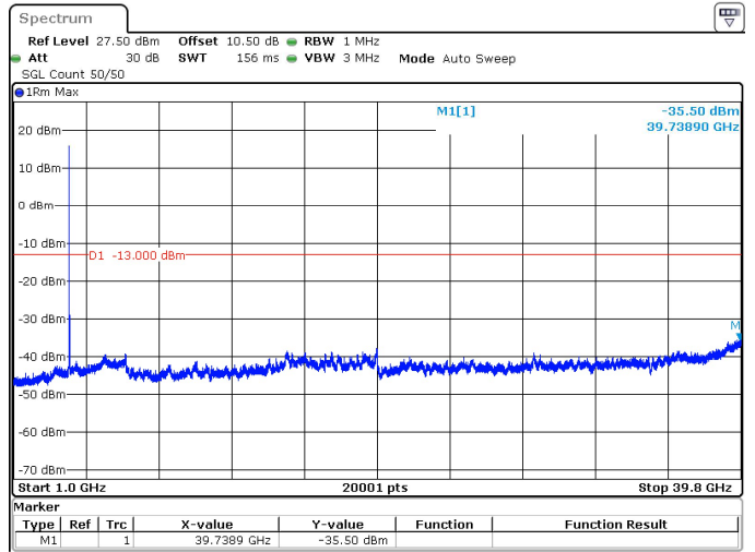
50MHz_15kHz_3955MHz_DFT-s-OFDM QPSK_RB1@0 -35.50 dBm
