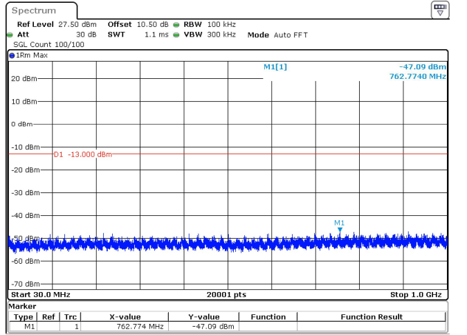
50MHz_15kHz_3725MHz_DFT-s-OFDM QPSK_RB270@0 -47.09 dBm
