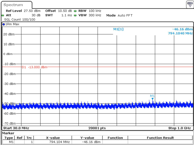
40MHz_30kHz_3960MHz_DFT-s-OFDM QPSK_RB100@0 -46.16 dBm
