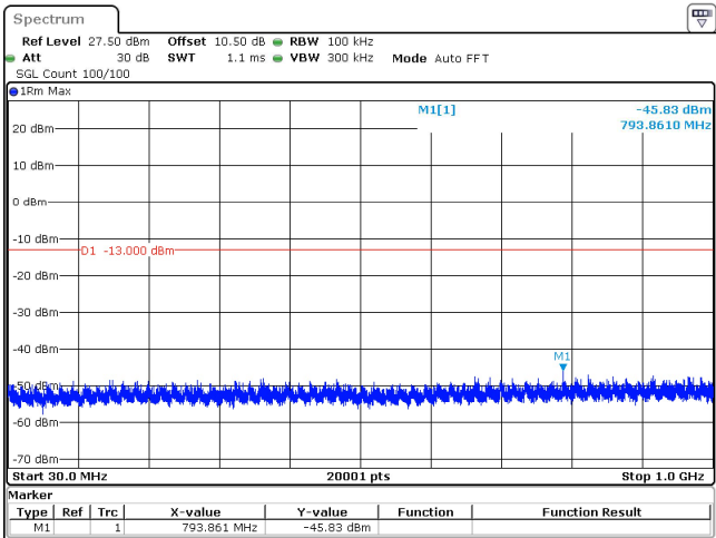
80MHz_30kHz_3740MHz_DFT-s-OFDM QPSK_RB1@216 -45.83 dBm
