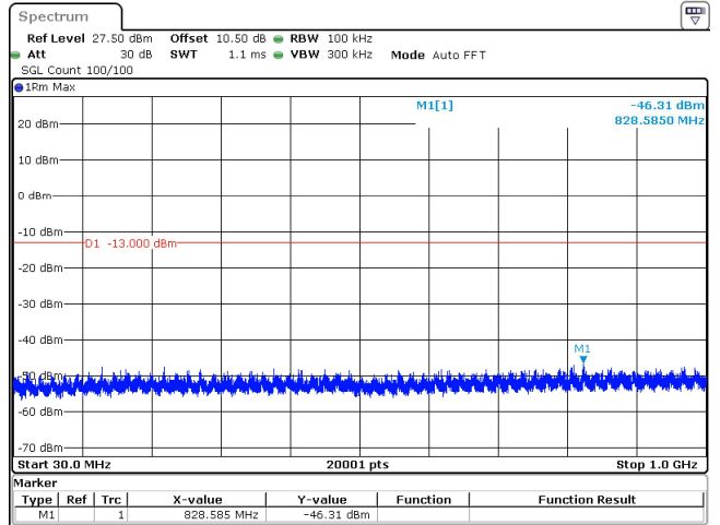
90MHz_30kHz_3935MHz_DFT-s-OFDM QPSK_RB243@0 -46.31 dBm
