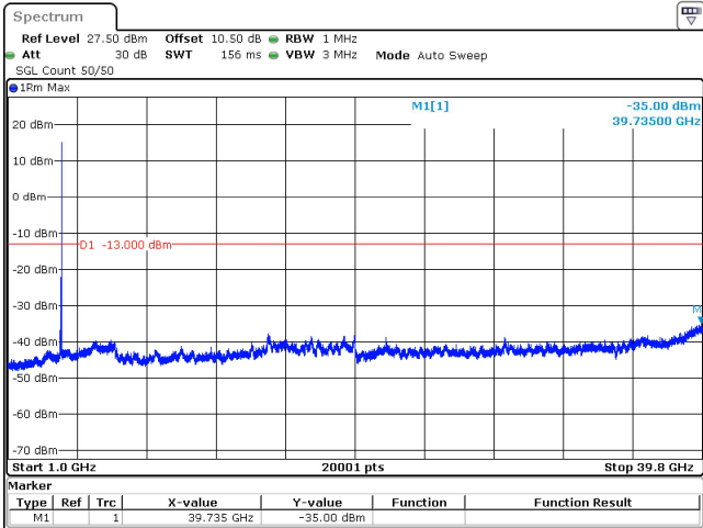
90MHz_30kHz_3935MHz_DFT-s-OFDM QPSK_RB1@244 -35.00 dBm
