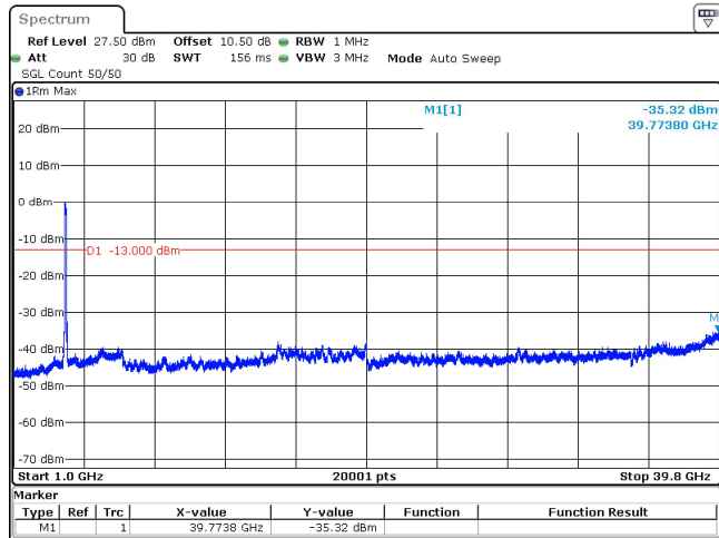
90MHz_30kHz_3840MHz_DFT-s-OFDM QPSK_RB243@0 -35.32 dBm
