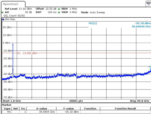
100MHz_30kHz_3840MHz_DFT-s-OFDM QPSK_RB270@0 -35.18 dBm
