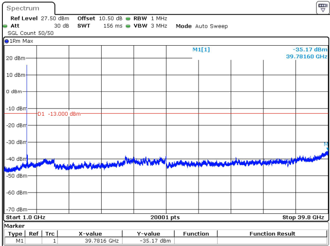
100MHz_30kHz_3750MHz_DFT-s-OFDM QPSK_RB1@0 -35.17 dBm
