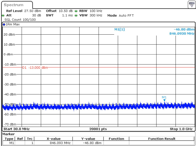
100MHz_30kHz_3750MHz_DFT-s-OFDM QPSK_RB1@272 -46.80 dBm
