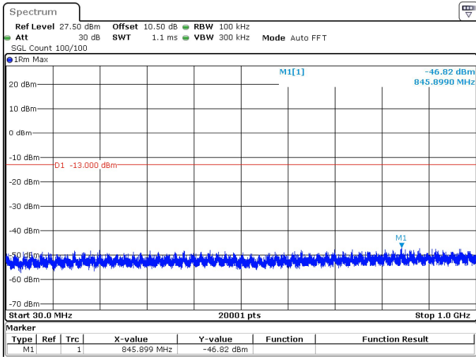
100MHz_30kHz_3930MHz_DFT-s-OFDM QPSK_RB1@272 -46.82 dBm
