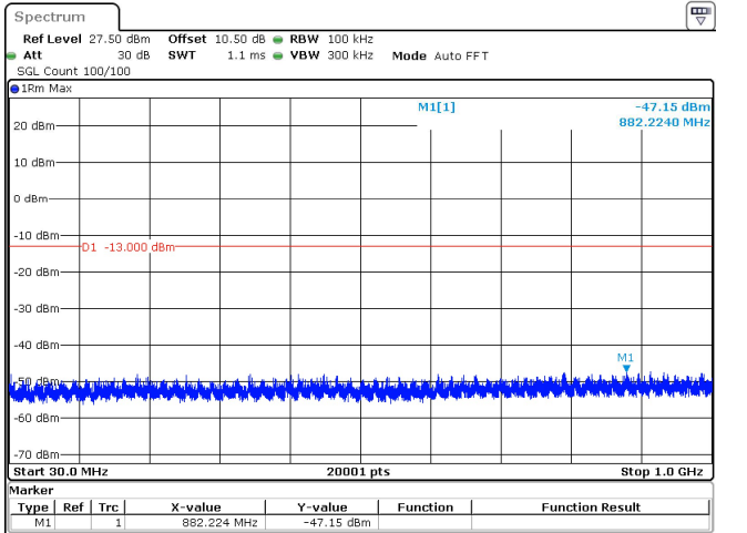
100MHz_30kHz_3930MHz_DFT-s-OFDM QPSK_RB270@0 -47.15 dBm
