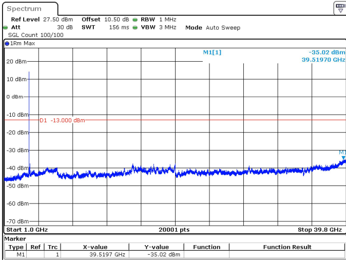
100MHz_30kHz_3840MHz_DFT-s-OFDM QPSK_RB1@0 -35.02 dBm
