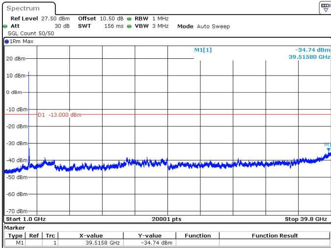
100MHz_30kHz_3930MHz_DFT-s-OFDM QPSK_RB1@0 -34.74 dBm
