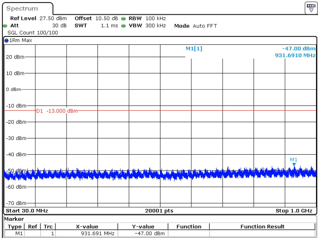
100MHz_30kHz_3750MHz_DFT-s-OFDM QPSK_RB270@0 -47.00 dBm
