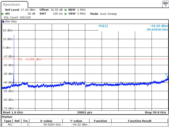
100MHz_30kHz_3750MHz_DFT-s-OFDM QPSK_RB1@272 -34.52 dBm
