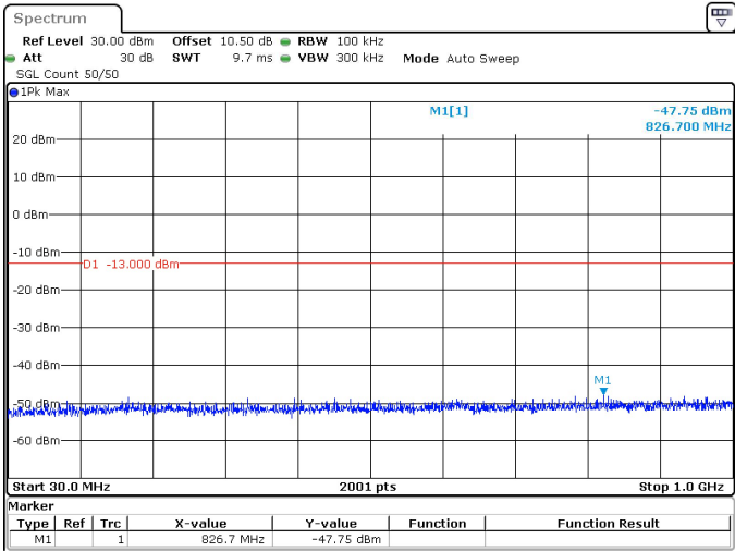
10MHz_30kHz_3455MHz_DFT-s-OFDM QPSK_RB24@0 -47.75 dBm
