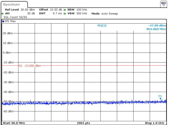
10MHz_30kHz_3455MHz_DFT-s-OFDM QPSK_RB24@0 -47.89 dBm
