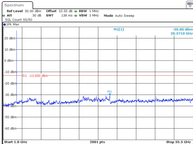
10MHz_30kHz_3455MHz_DFT-s-OFDM QPSK_RB1@23 -30.80 dBm
