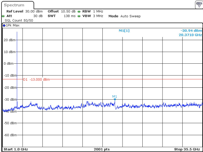
10MHz_30kHz_3500MHz_DFT-s-OFDM QPSK_RB1@0 -30.94 dBm
