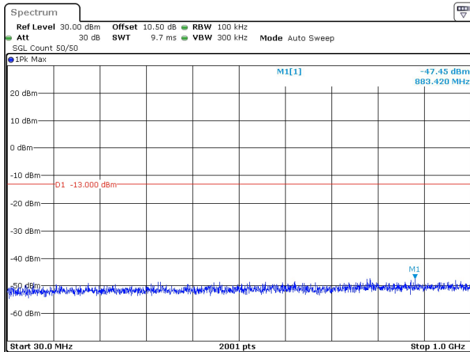
10MHz_30kHz_3455MHz_DFT-s-OFDM QPSK_RB1@0 -47.45 dBm
