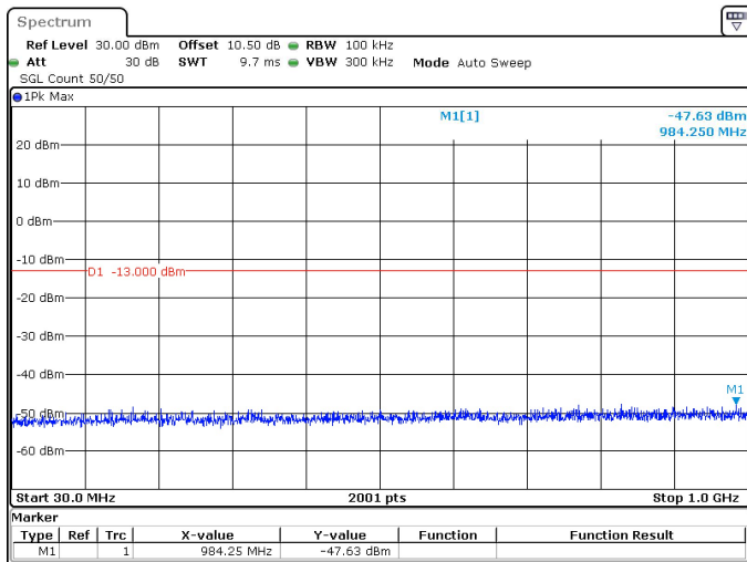
10MHz_30kHz_3455MHz_DFT-s-OFDM QPSK_RB1@0 -47.63 dBm
