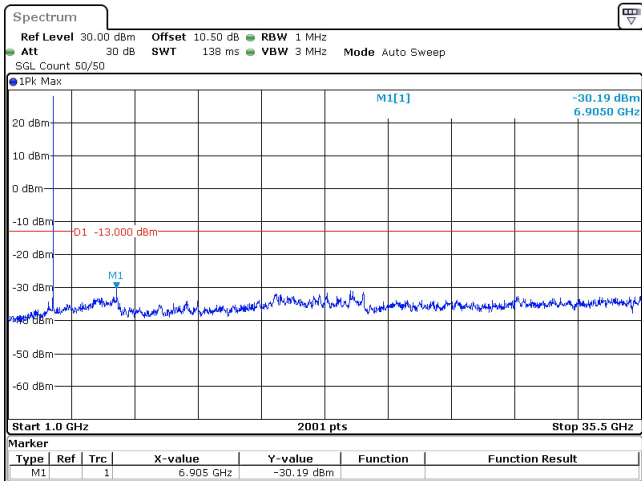
10MHz_30kHz_3455MHz_DFT-s-OFDM QPSK_RB1@0 -30.19 dBm
