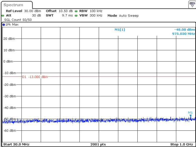
10MHz_30kHz_3455MHz_DFT-s-OFDM QPSK_RB1@23 -48.00 dBm
