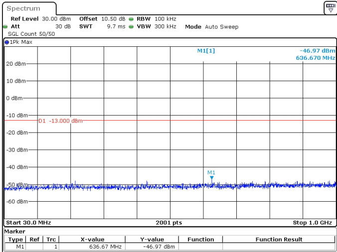
10MHz_30kHz_3500MHz_DFT-s-OFDM QPSK_RB1@0 -46.97 dBm
