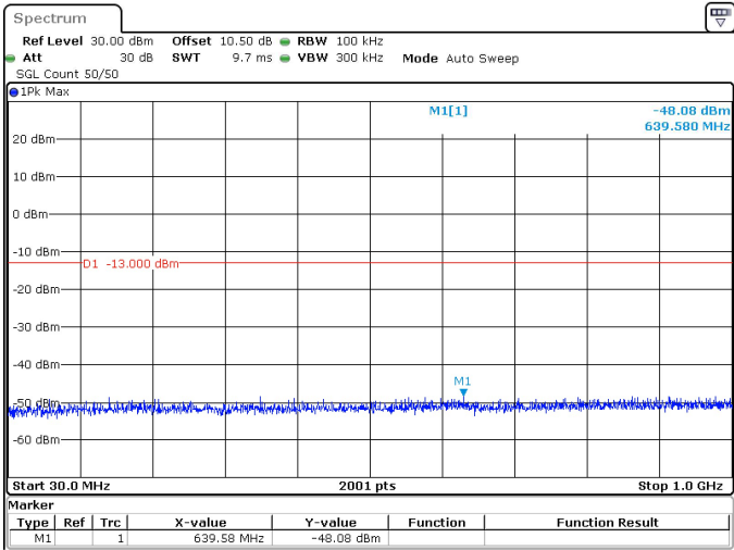
10MHz_30kHz_3500MHz_DFT-s-OFDM QPSK_RB24@0 -48.08 dBm
