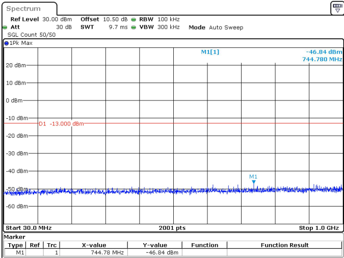
10MHz_30kHz_3500MHz_DFT-s-OFDM QPSK_RB1@23 -46.84 dBm
