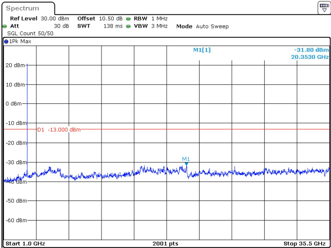
10MHz_30kHz_3500MHz_DFT-s-OFDM QPSK_RB24@0 -31.80 dBm
