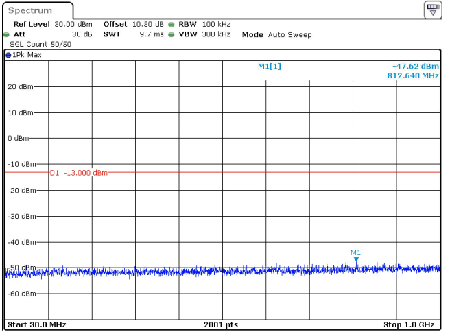
10MHz_30kHz_3500MHz_DFT-s-OFDM QPSK_RB24@0 -47.62 dBm
