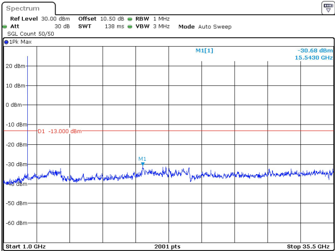
10MHz_30kHz_3500MHz_DFT-s-OFDM QPSK_RB1@23 -30.68 dBm
