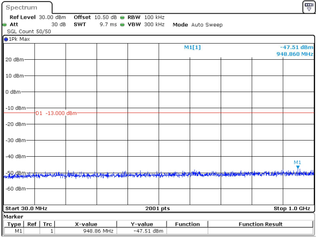
10MHz_30kHz_3545MHz_DFT-s-OFDM QPSK_RB24@0 -47.51 dBm
