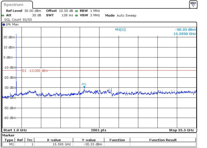
10MHz_30kHz_3500MHz_DFT-s-OFDM QPSK_RB24@0 -30.33 dBm
