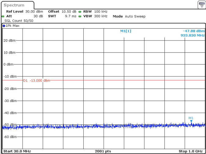
10MHz_30kHz_3545MHz_DFT-s-OFDM QPSK_RB24@0 -47.88 dBm
