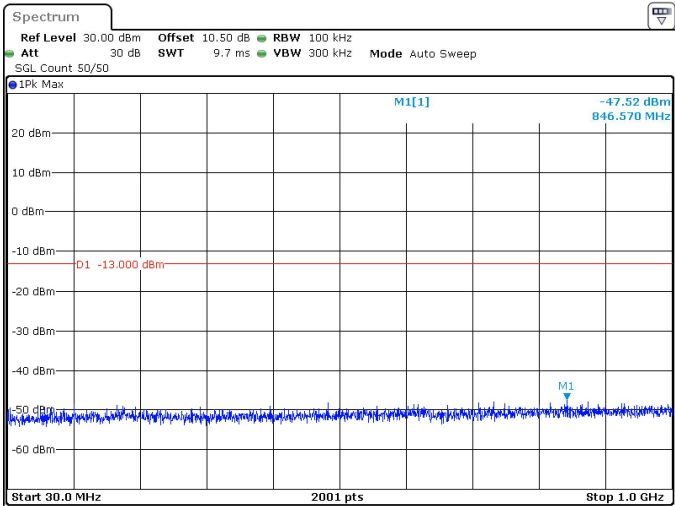
30MHz_30kHz_3465MHz_DFT-s-OFDM QPSK_RB75@0 -47.52 dBm
