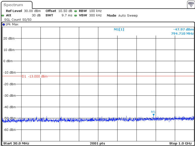
30MHz_30kHz_3500MHz_DFT-s-OFDM QPSK_RB75@0 -47.97 dBm
