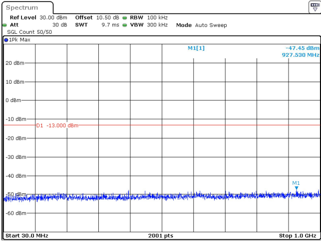
30MHz_30kHz_3500MHz_DFT-s-OFDM QPSK_RB1@0 -47.45 dBm
