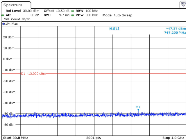
30MHz_30kHz_3465MHz_DFT-s-OFDM QPSK_RB1@0 -47.37 dBm
