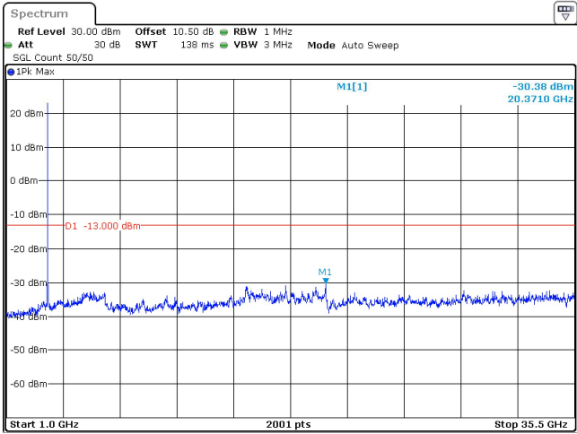
30MHz_30kHz_3500MHz_DFT-s-OFDM QPSK_RB1@0 -30.38 dBm
