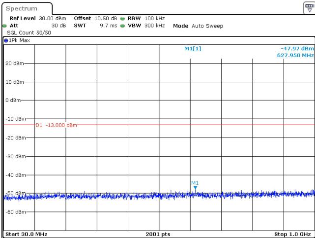
30MHz_30kHz_3535MHz_DFT-s-OFDM QPSK_RB1@0 -47.97 dBm
