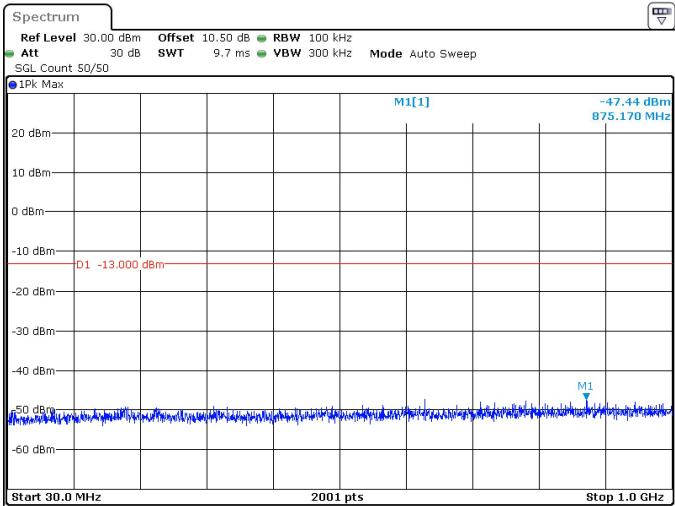
30MHz_30kHz_3465MHz_DFT-s-OFDM QPSK_RB1@77 -47.44 dBm
