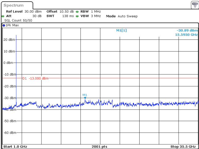
30MHz_30kHz_3465MHz_DFT-s-OFDM QPSK_RB1@0 -30.89 dBm
