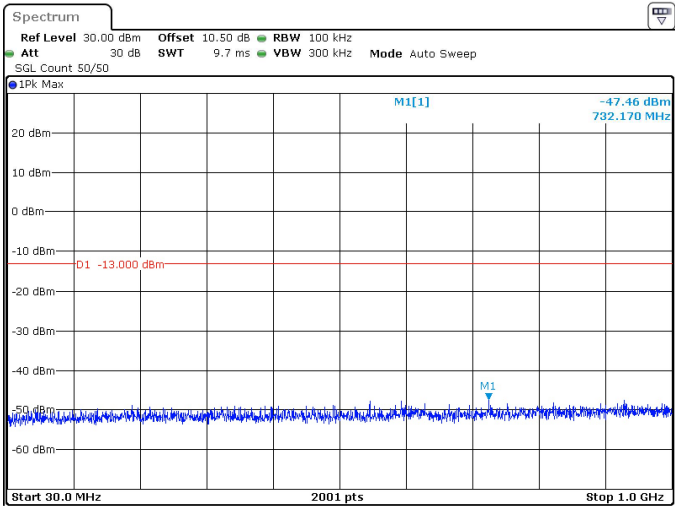
25MHz_30kHz_3537.5MHz_DFT-s-OFDM QPSK_RB64@0 -47.46 dBm
