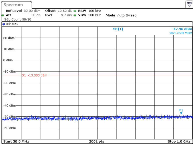
25MHz_30kHz_3537.5MHz_DFT-s-OFDM QPSK_RB1@64 -47.96 dBm
