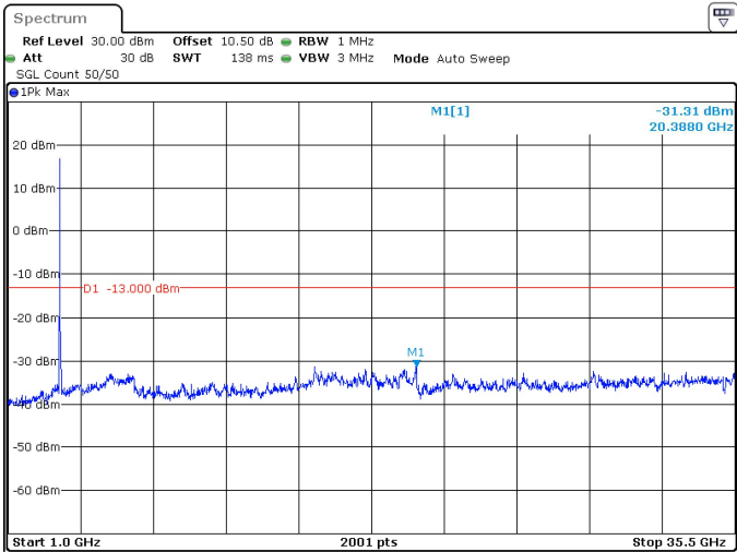
30MHz_30kHz_3465MHz_DFT-s-OFDM QPSK_RB75@0 -31.31 dBm
