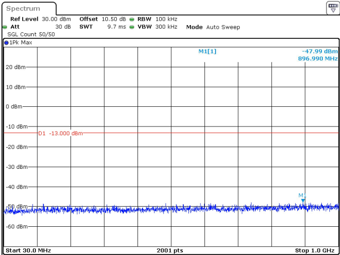
30MHz_30kHz_3500MHz_DFT-s-OFDM QPSK_RB1@77 -47.99 dBm
