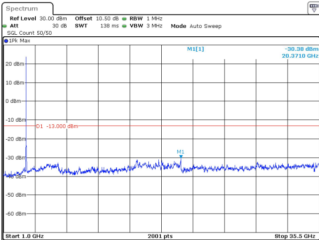
60MHz_30kHz_3480MHz_DFT-s-OFDM QPSK_RB1@0 -30.38 dBm
