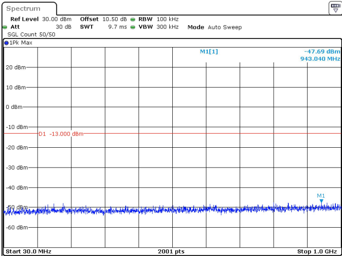
60MHz_30kHz_3500MHz_DFT-s-OFDM QPSK_RB162@0 -47.69 dBm
