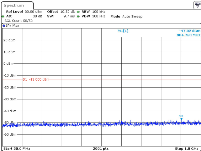
60MHz_30kHz_3500MHz_DFT-s-OFDM QPSK_RB1@0 -47.82 dBm
