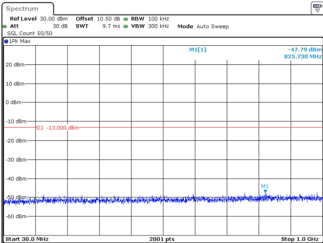
60MHz_30kHz_3480MHz_DFT-s-OFDM QPSK_RB1@0 -47.79 dBm
