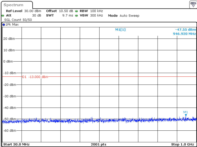
60MHz_30kHz_3480MHz_DFT-s-OFDM QPSK_RB1@161 -47.55 dBm
