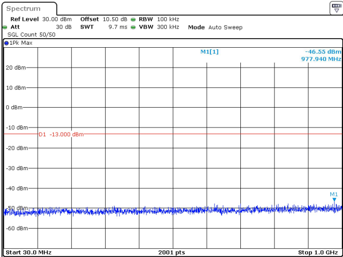
60MHz_30kHz_3480MHz_DFT-s-OFDM QPSK_RB162@0 -46.55 dBm
