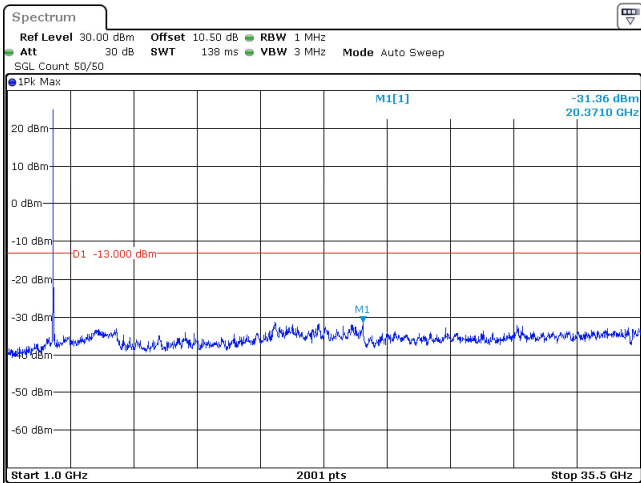
60MHz_30kHz_3520MHz_DFT-s-OFDM QPSK_RB1@0 -31.36 dBm
