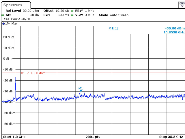
60MHz_30kHz_3500MHz_DFT-s-OFDM QPSK_RB1@0 -30.80 dBm
