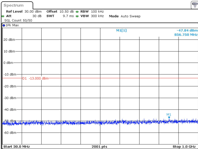
60MHz_30kHz_3520MHz_DFT-s-OFDM QPSK_RB1@0 -47.84 dBm
