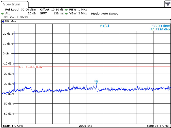
90MHz_30kHz_3500MHz_DFT-s-OFDM QPSK_RB1@244 -30.51 dBm
