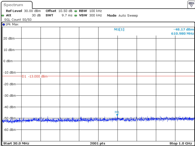
90MHz_30kHz_3495MHz_DFT-s-OFDM QPSK_RB243@0 -48.17 dBm
