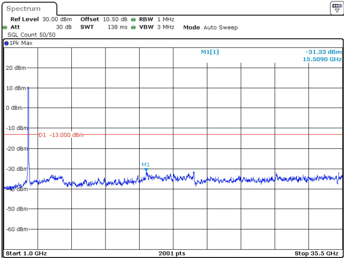
80MHz_30kHz_3510MHz_DFT-s-OFDM QPSK_RB216@0 -31.33 dBm
