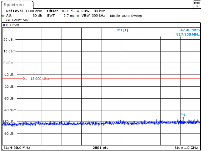
90MHz_30kHz_3505MHz_DFT-s-OFDM QPSK_RB1@0 -47.48 dBm
