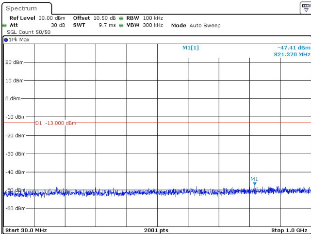
90MHz_30kHz_3495MHz_DFT-s-OFDM QPSK_RB1@0 -47.41 dBm
