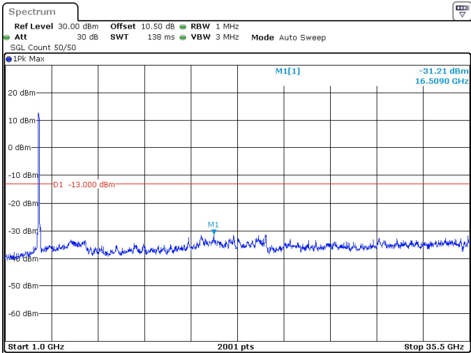
90MHz_30kHz_3500MHz_DFT-s-OFDM QPSK_RB243@0 -31.21 dBm
