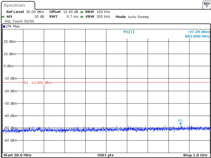
90MHz_30kHz_3500MHz_DFT-s-OFDM QPSK_RB243@0 -47.39 dBm
