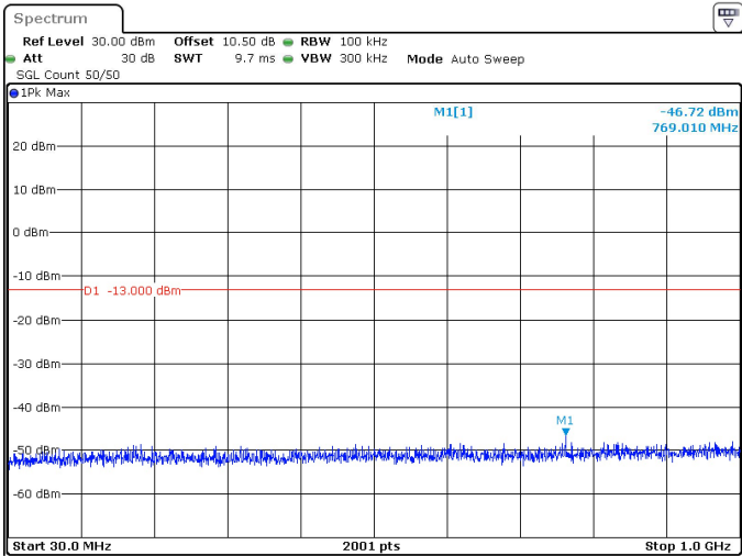
80MHz_30kHz_3510MHz_DFT-s-OFDM QPSK_RB1@216 -46.72 dBm
