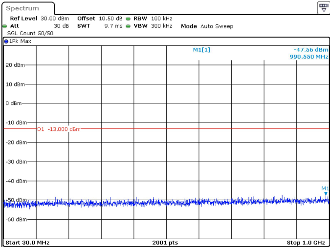
80MHz_30kHz_3510MHz_DFT-s-OFDM QPSK_RB216@0 -47.56 dBm
