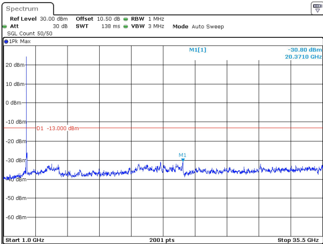
90MHz_30kHz_3495MHz_DFT-s-OFDM QPSK_RB1@0 -30.80 dBm
