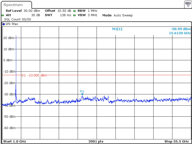
80MHz_30kHz_3510MHz_DFT-s-OFDM QPSK_RB1@216 -30.99 dBm
