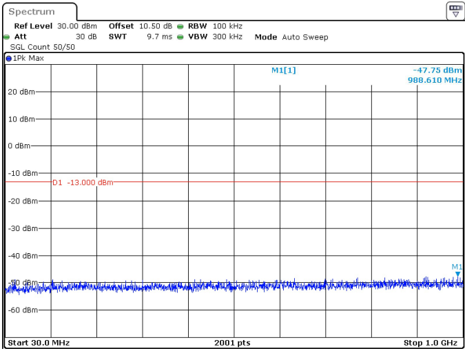
90MHz_30kHz_3500MHz_DFT-s-OFDM QPSK_RB1@244 -47.75 dBm
