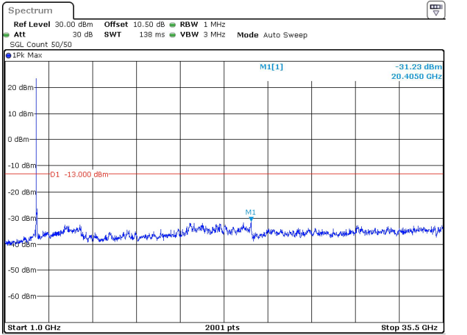
90MHz_30kHz_3500MHz_DFT-s-OFDM QPSK_RB1@0 -31.23 dBm
