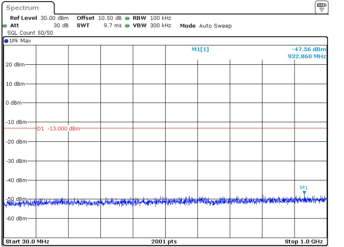
90MHz_30kHz_3500MHz_DFT-s-OFDM QPSK_RB1@0 -47.56 dBm
