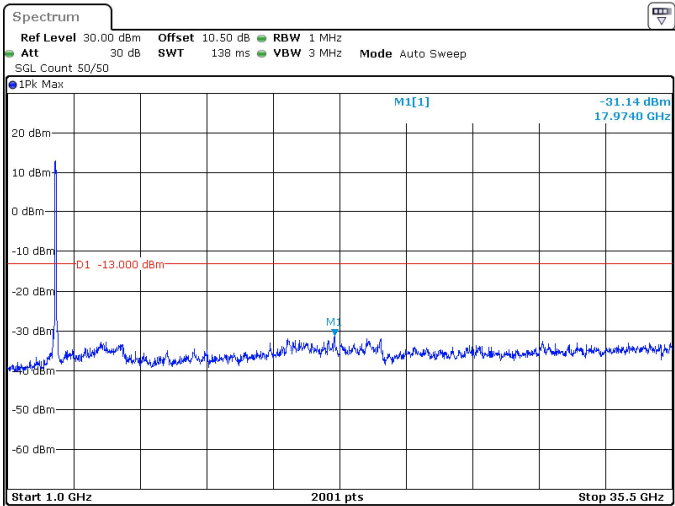
90MHz_30kHz_3495MHz_DFT-s-OFDM QPSK_RB243@0 -31.14 dBm
