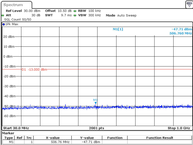
10MHz_30kHz_3750MHz_DFT-s-OFDM QPSK_RB1@23 -47.71 dBm
