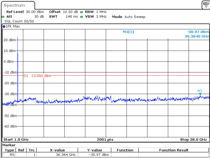
10MHz_30kHz_3750MHz_DFT-s-OFDM QPSK_RB24@0 -30.97 dBm
