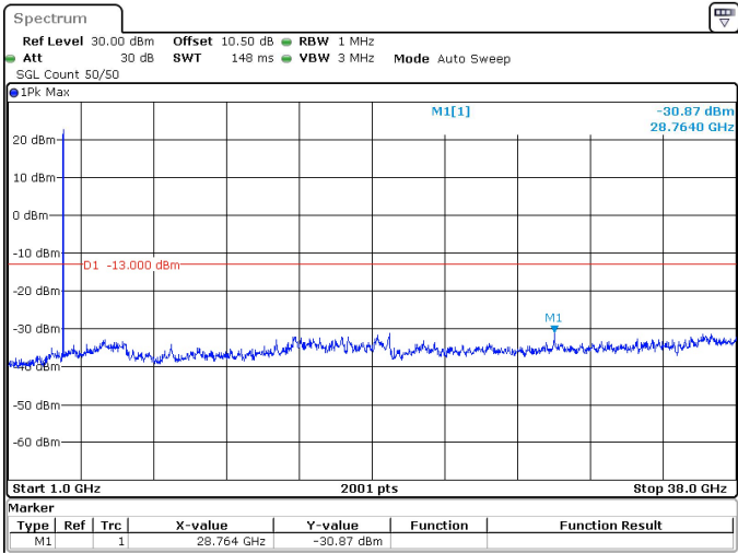
10MHz_30kHz_3795MHz_DFT-s-OFDM QPSK_RB24@0 -30.87 dBm
