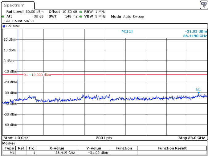
10MHz_30kHz_3795MHz_DFT-s-OFDM QPSK_RB1@23 -31.02 dBm
