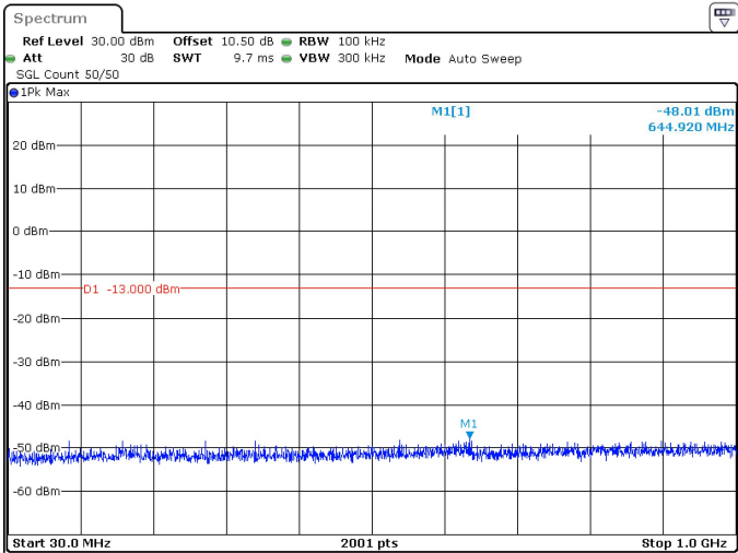
15MHz_15kHz_3707.5MHz_DFT-s-OFDM QPSK_RB75@0 -48.01 dBm
