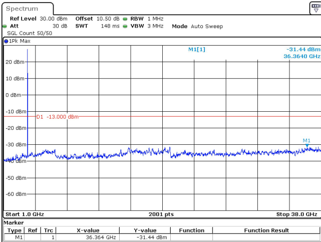
10MHz_30kHz_3795MHz_DFT-s-OFDM QPSK_RB1@0 -31.44 dBm
