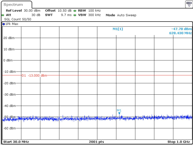
15MHz_15kHz_3707.5MHz_DFT-s-OFDM QPSK_RB1@0 -47.78 dBm
