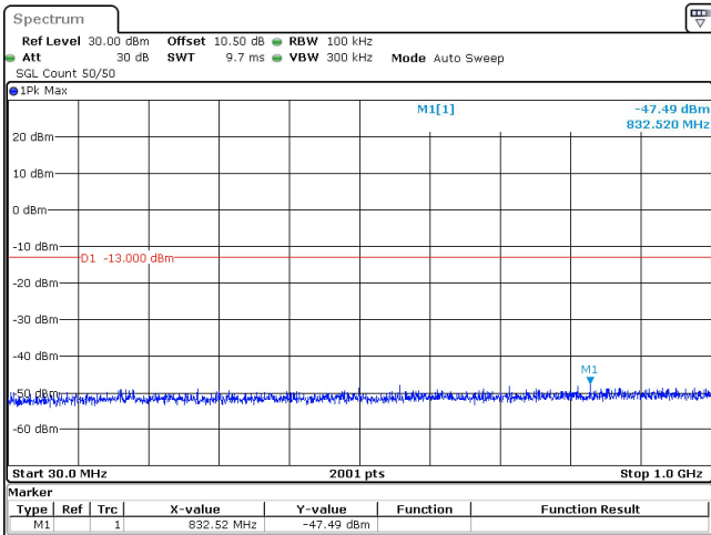
15MHz_30kHz_3750MHz_DFT-s-OFDM QPSK_RB1@0 -47.49 dBm
