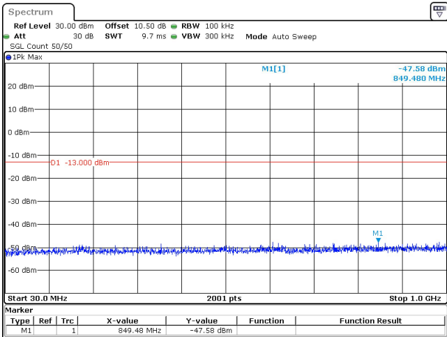
15MHz_30kHz_3707.5MHz_DFT-s-OFDM QPSK_RB1@0 -47.58 dBm
