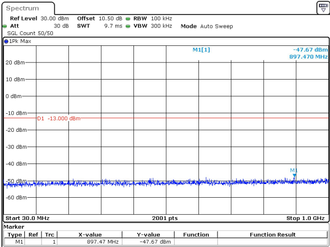
15MHz_30kHz_3707.5MHz_DFT-s-OFDM QPSK_RB1@37 -47.67 dBm
