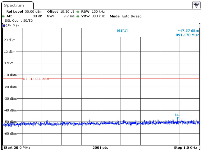
25MHz_15kHz_3712.5MHz_DFT-s-OFDM QPSK_RB1@0 -47.57 dBm
