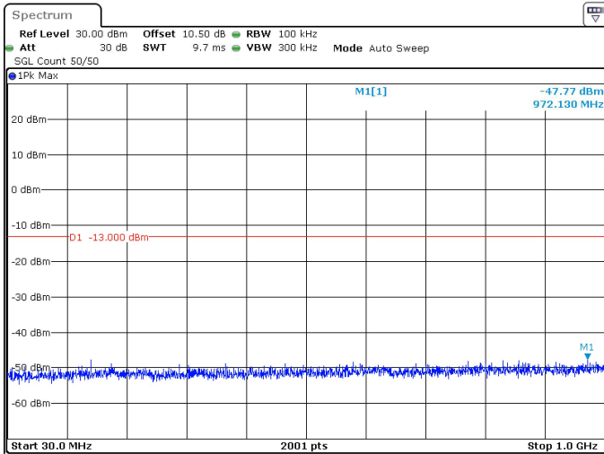
25MHz_15kHz_3712.5MHz_DFT-s-OFDM QPSK_RB128@0 -47.77 dBm
