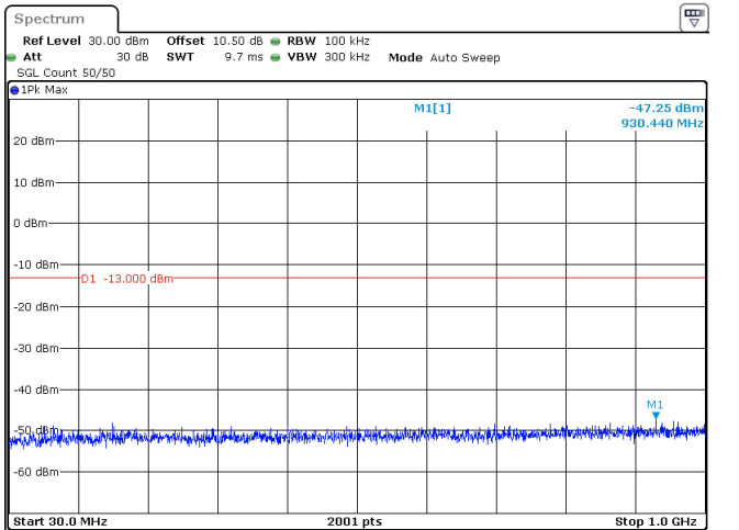
25MHz_15kHz_3750MHz_DFT-s-OFDM QPSK_RB1@0 -47.25 dBm
