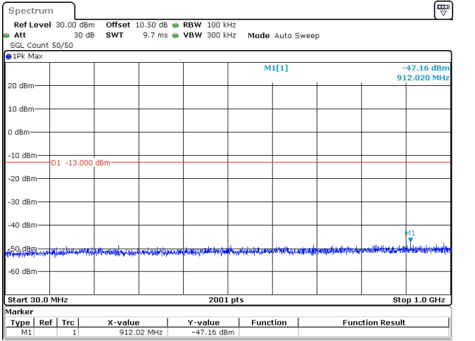
15MHz_30kHz_3792.5MHz_DFT-s-OFDM QPSK_RB1@0 -47.16 dBm
