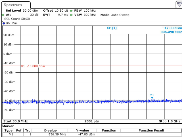
25MHz_30kHz_3750MHz_DFT-s-OFDM QPSK_RB1@0 -47.80 dBm
