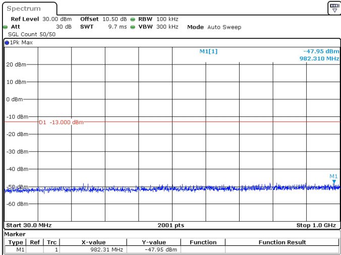
25MHz_30kHz_3712.5MHz_DFT-s-OFDM QPSK_RB1@64 -47.95 dBm
