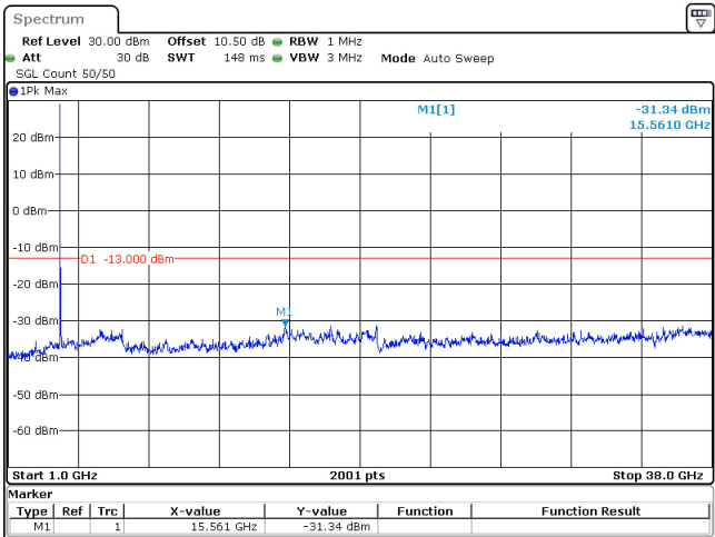
25MHz_30kHz_3750MHz_DFT-s-OFDM QPSK_RB1@0 -31.34 dBm
