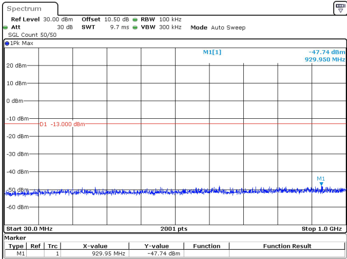
25MHz_30kHz_3712.5MHz_DFT-s-OFDM QPSK_RB64@0 -47.74 dBm
