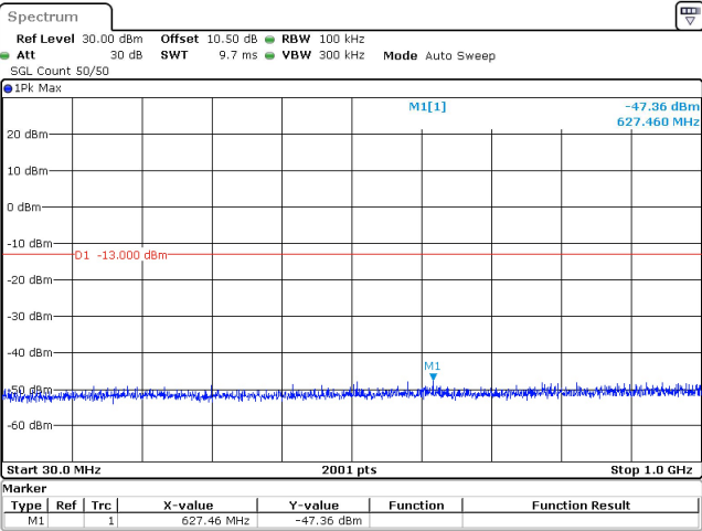
25MHz_30kHz_3712.5MHz_DFT-s-OFDM QPSK_RB1@0 -47.36 dBm
