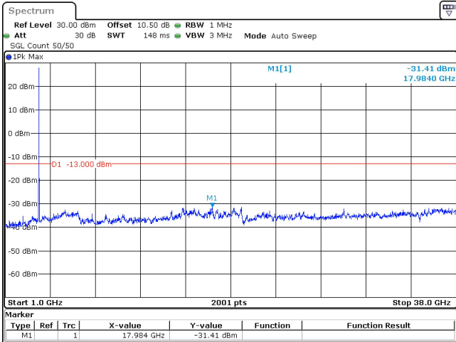
30MHz_30kHz_3785MHz_DFT-s-OFDM QPSK_RB1@0 -31.41 dBm
