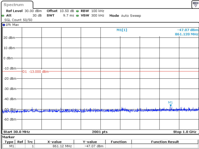
30MHz_30kHz_3785MHz_DFT-s-OFDM QPSK_RB1@0 -47.07 dBm
