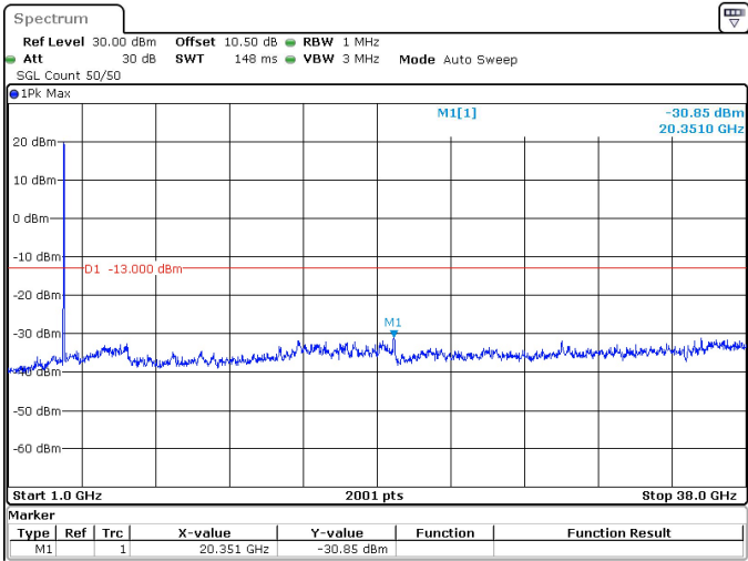
30MHz_30kHz_3785MHz_DFT-s-OFDM QPSK_RB75@0 -30.85 dBm
