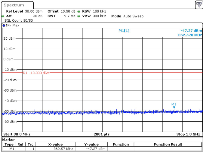
30MHz_30kHz_3750MHz_DFT-s-OFDM QPSK_RB1@77 -47.27 dBm
