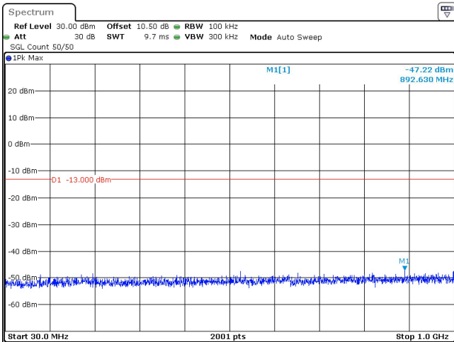
40MHz_15kHz_3720MHz_DFT-s-OFDM QPSK_RB1@0 -47.22 dBm
