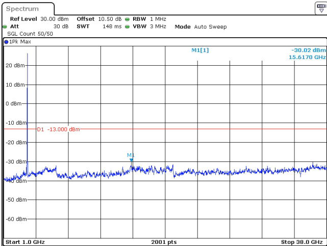
40MHz_15kHz_3720MHz_DFT-s-OFDM QPSK_RB1@0 -30.02 dBm
