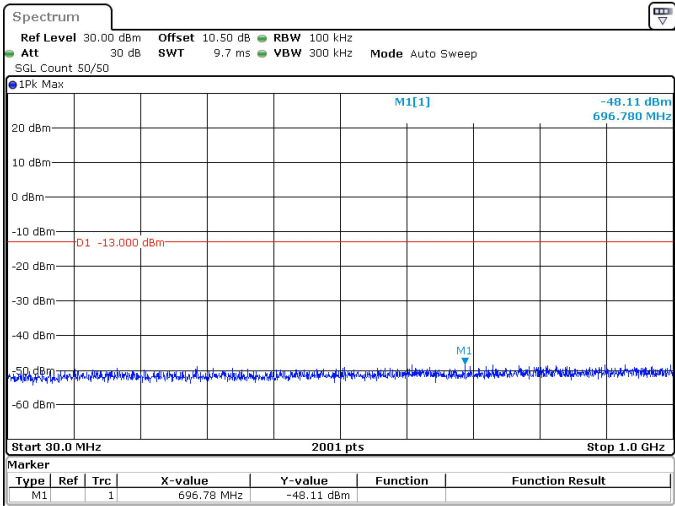
30MHz_30kHz_3785MHz_DFT-s-OFDM QPSK_RB1@77 -48.11 dBm
