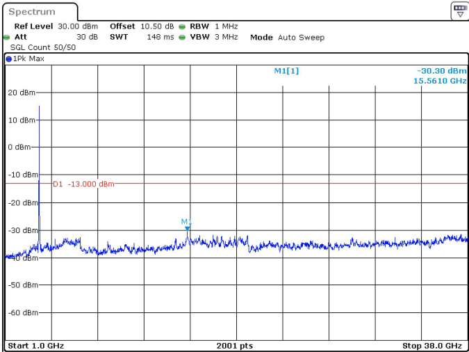
40MHz_15kHz_3720MHz_DFT-s-OFDM QPSK_RB216@0 -30.30 dBm
