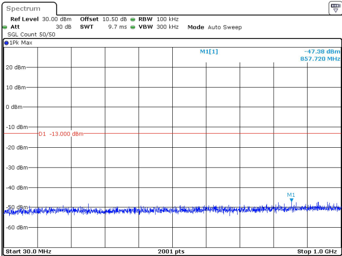
40MHz_15kHz_3720MHz_DFT-s-OFDM QPSK_RB1@215 -47.38 dBm
