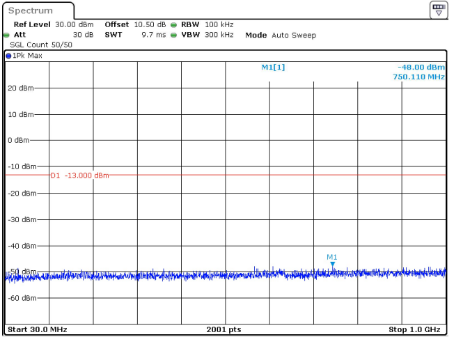
40MHz_15kHz_3750MHz_DFT-s-OFDM QPSK_RB1@0 -48.00 dBm
