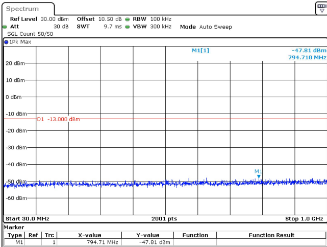
40MHz_30kHz_3720MHz_DFT-s-OFDM QPSK_RB1@0 -47.81 dBm
