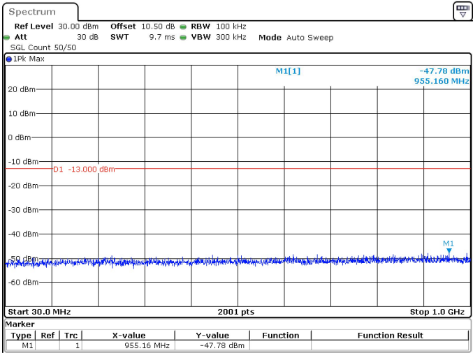
40MHz_30kHz_3720MHz_DFT-s-OFDM QPSK_RB100@0 -47.78 dBm
