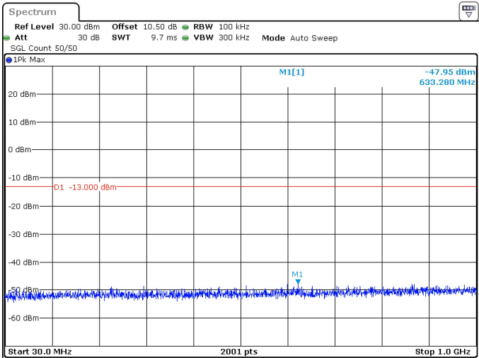
40MHz_15kHz_3750MHz_DFT-s-OFDM QPSK_RB216@0 -47.95 dBm
