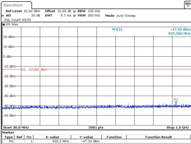
40MHz_30kHz_3750MHz_DFT-s-OFDM QPSK_RB1@0 -47.33 dBm
