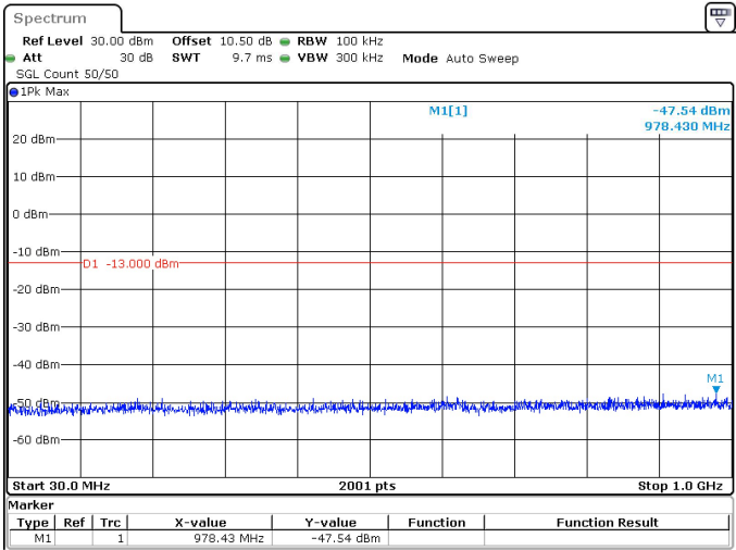
40MHz_30kHz_3720MHz_DFT-s-OFDM QPSK_RB1@105 -47.54 dBm
