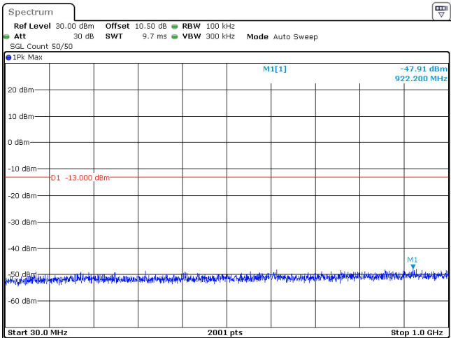
40MHz_15kHz_3780MHz_DFT-s-OFDM QPSK_RB1@0 -47.91 dBm
