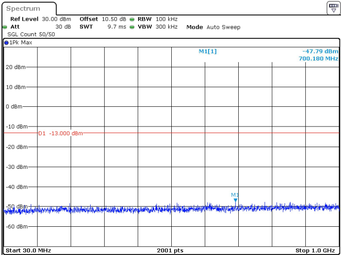
40MHz_15kHz_3750MHz_DFT-s-OFDM QPSK_RB1@215 -47.79 dBm
