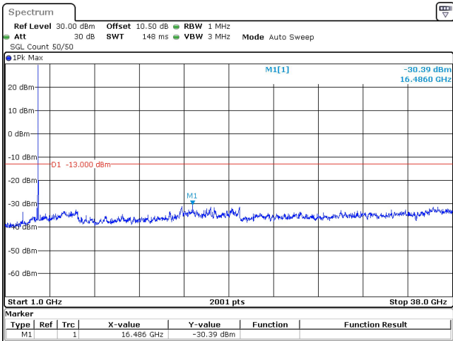
40MHz_30kHz_3750MHz_DFT-s-OFDM QPSK_RB1@0 -30.39 dBm
