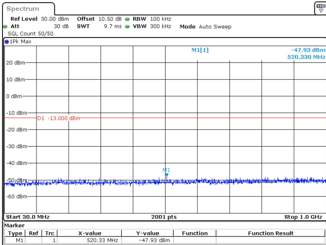
40MHz_30kHz_3780MHz_DFT-s-OFDM QPSK_RB1@0 -47.93 dBm
