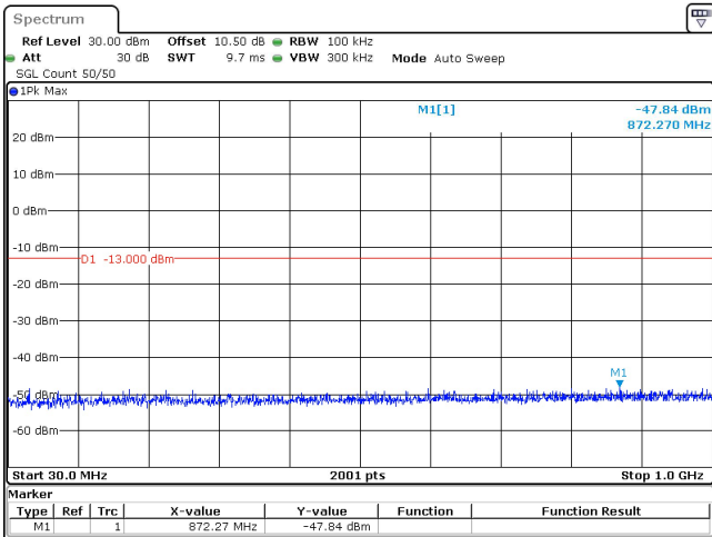
50MHz_15kHz_3750MHz_DFT-s-OFDM QPSK_RB1@0 -47.84 dBm
