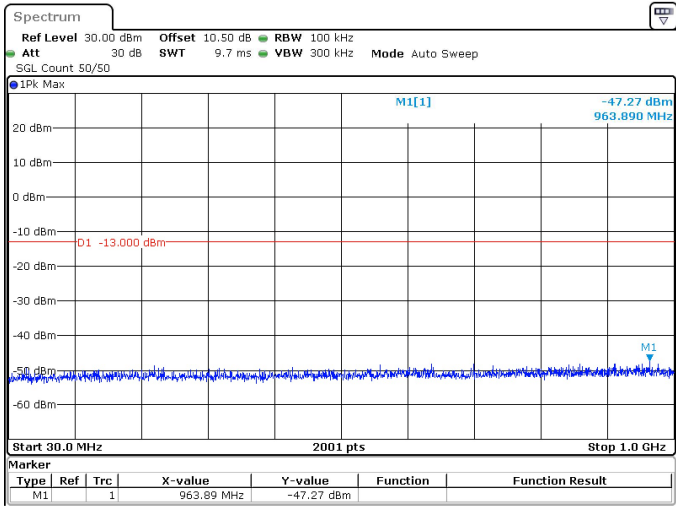
40MHz_30kHz_3750MHz_DFT-s-OFDM QPSK_RB100@0 -47.27 dBm
