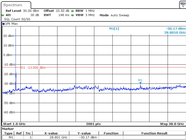
50MHz_30kHz_3775MHz_DFT-s-OFDM QPSK_RB1@0 -30.17 dBm
