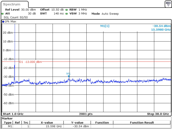
60MHz_30kHz_3770MHz_DFT-s-OFDM QPSK_RB1@161 -30.54 dBm
