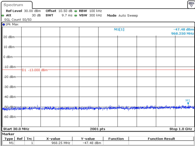
70MHz_30kHz_3735MHz_DFT-s-OFDM QPSK_RB180@0 -47.48 dBm
