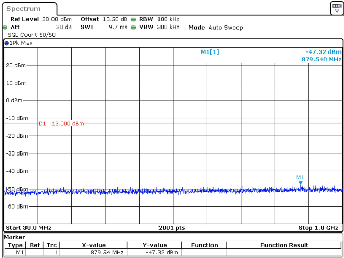
60MHz_30kHz_3770MHz_DFT-s-OFDM QPSK_RB1@161 -47.32 dBm
