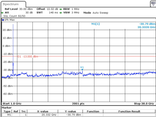
70MHz_30kHz_3750MHz_DFT-s-OFDM QPSK_RB1@0 -30.79 dBm
