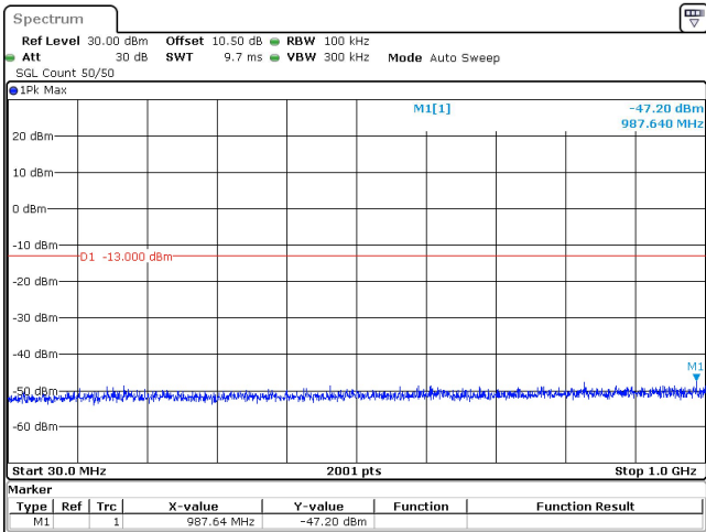
60MHz_30kHz_3770MHz_DFT-s-OFDM QPSK_RB1@0 -47.20 dBm
