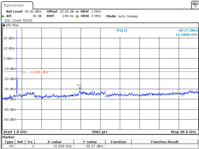
60MHz_30kHz_3770MHz_DFT-s-OFDM QPSK_RB1@0 -30.27 dBm
