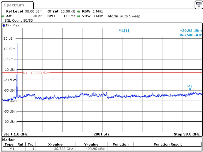
70MHz_30kHz_3735MHz_DFT-s-OFDM QPSK_RB180@0 -29.95 dBm
