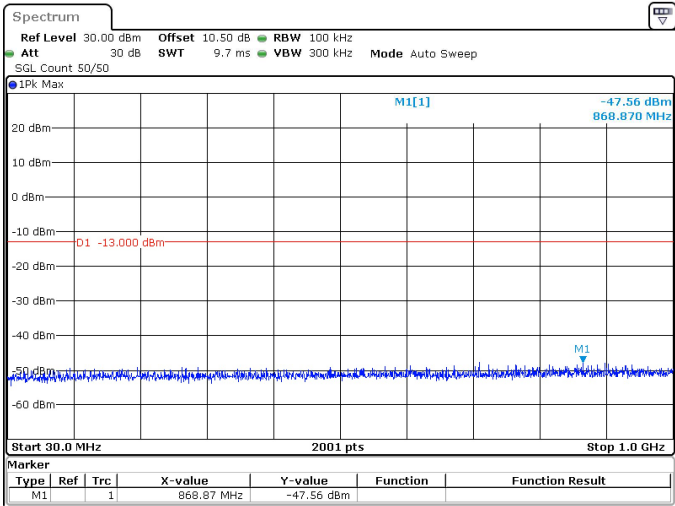
60MHz_30kHz_3750MHz_DFT-s-OFDM QPSK_RB162@0 -47.56 dBm
