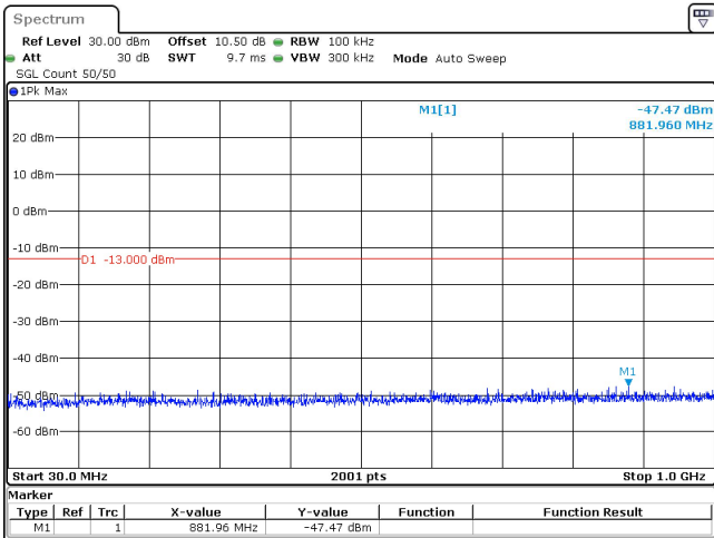
70MHz_30kHz_3750MHz_DFT-s-OFDM QPSK_RB1@0 -47.47 dBm
