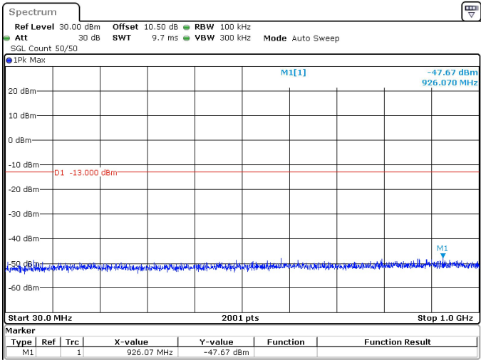
60MHz_30kHz_3750MHz_DFT-s-OFDM QPSK_RB1@161 -47.67 dBm
