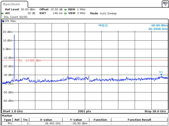
60MHz_30kHz_3770MHz_DFT-s-OFDM QPSK_RB162@0 -30.80 dBm
