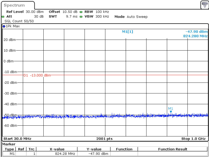
60MHz_30kHz_3770MHz_DFT-s-OFDM QPSK_RB162@0 -47.90 dBm
