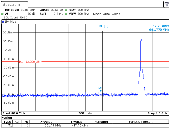
10MHz_15kHz_836.5MHz_DFT-s-OFDM QPSK_RB50@0&-47.70 dBm
