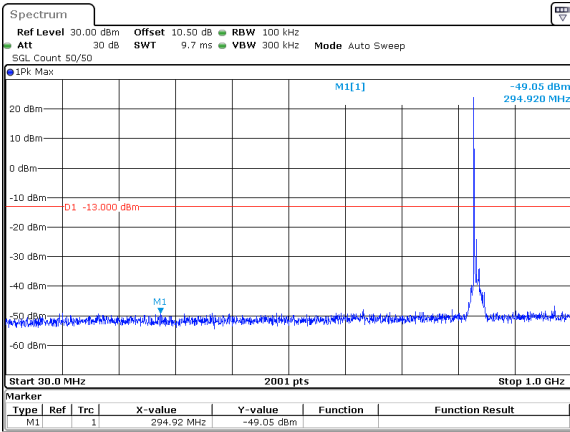
10MHz_15kHz_836.5MHz_DFT-s-OFDM QPSK_RB1@0&-49.05 dBm
