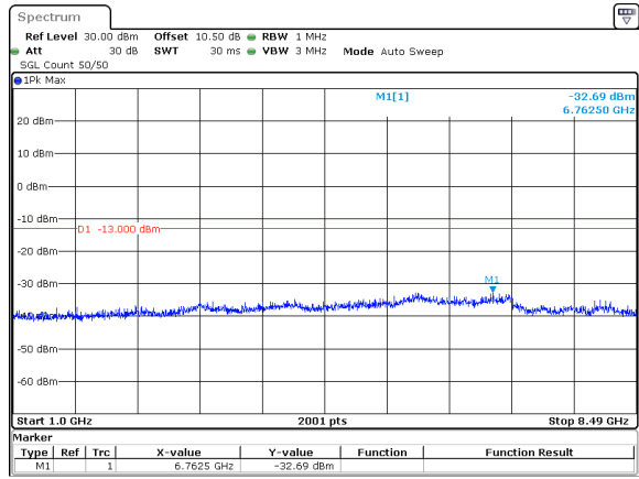
20MHz_15kHz_839MHz_DFT-s-OFDM QPSK_RB100@0&-32.69 dBm
