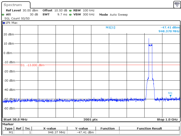
20MHz_15kHz_839MHz_DFT-s-OFDM QPSK_RB100@0&-47.41 dBm
