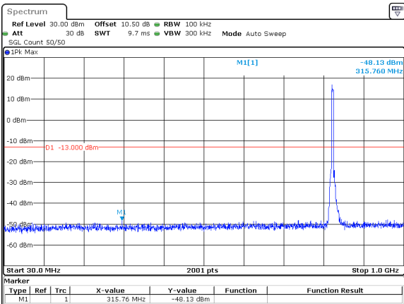
5MHz_15kHz_826.5MHz_DFT-s-OFDM QPSK_RB25@0&-48.13 dBm
