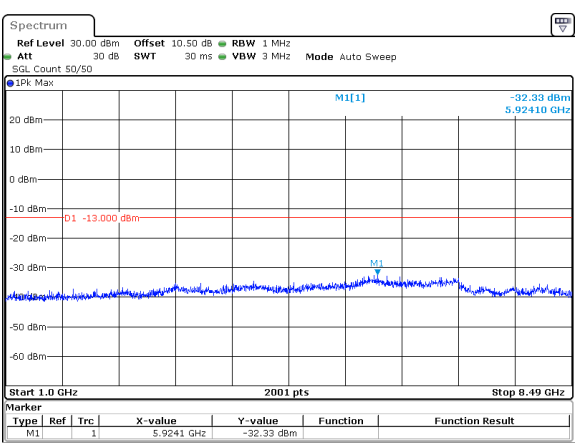
10MHz_15kHz_844MHz_DFT-s-OFDM QPSK_RB50@0&-32.33 dBm
