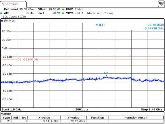
20MHz_15kHz_834MHz_DFT-s-OFDM QPSK_RB1@0&-32.78 dBm
