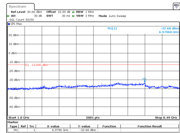
20MHz_15kHz_839MHz_DFT-s-OFDM QPSK_RB1@0&-32.68 dBm
