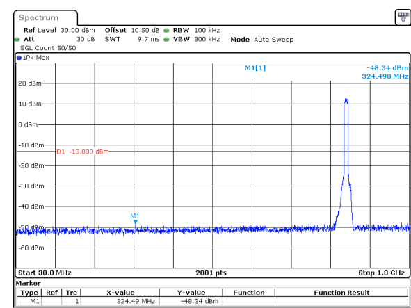
10MHz_15kHz_844MHz_DFT-s-OFDM QPSK_RB50@0&-48.34 dBm
