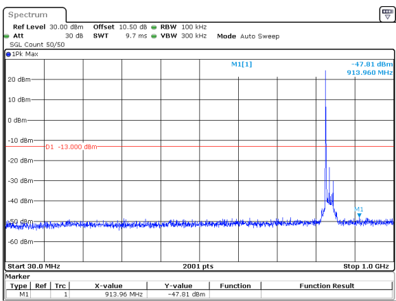
20MHz_15kHz_839MHz_DFT-s-OFDM QPSK_RB1@0&-47.81 dBm
