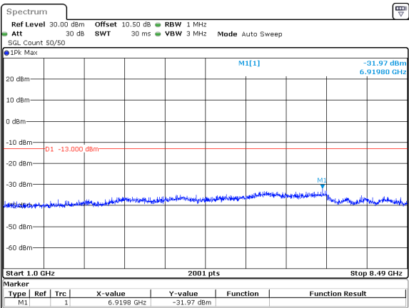
10MHz_15kHz_829MHz_DFT-s-OFDM QPSK_RB50@0&-31.97 dBm
