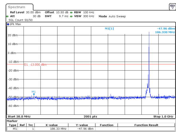
10MHz_15kHz_844MHz_DFT-s-OFDM QPSK_RB1@51&-47.96 dBm
