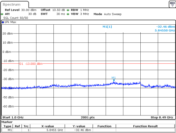
10MHz_15kHz_829MHz_DFT-s-OFDM QPSK_RB1@0&-32.46 dBm
