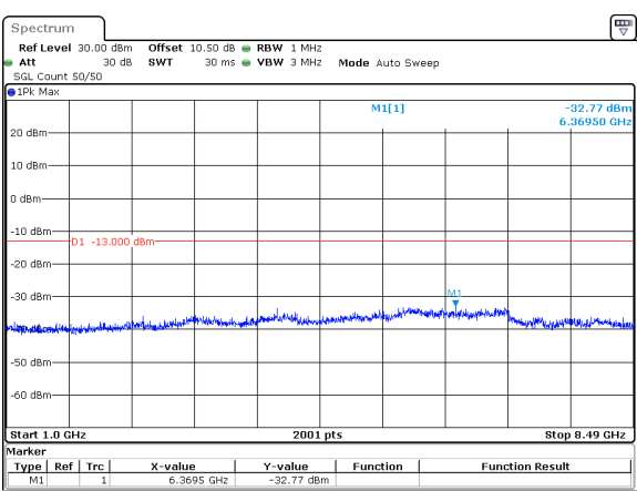
10MHz_15kHz_844MHz_DFT-s-OFDM QPSK_RB1@0&-32.77 dBm
