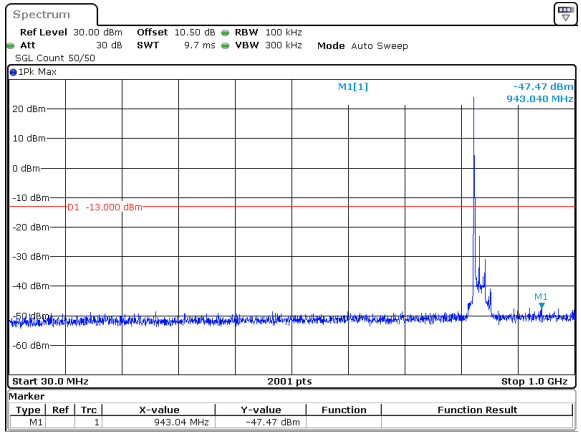
20MHz_15kHz_836.5MHz_DFT-s-OFDM QPSK_RB1@0&-47.47 dBm
