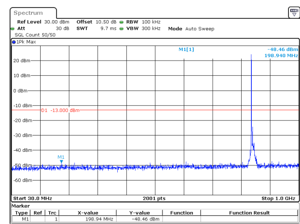
10MHz_15kHz_844MHz_DFT-s-OFDM QPSK_RB1@0&-48.46 dBm
