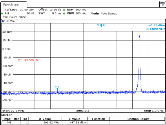
5MHz_15kHz_846.5MHz_DFT-s-OFDM QPSK_RB25@0&-47.88 dBm
